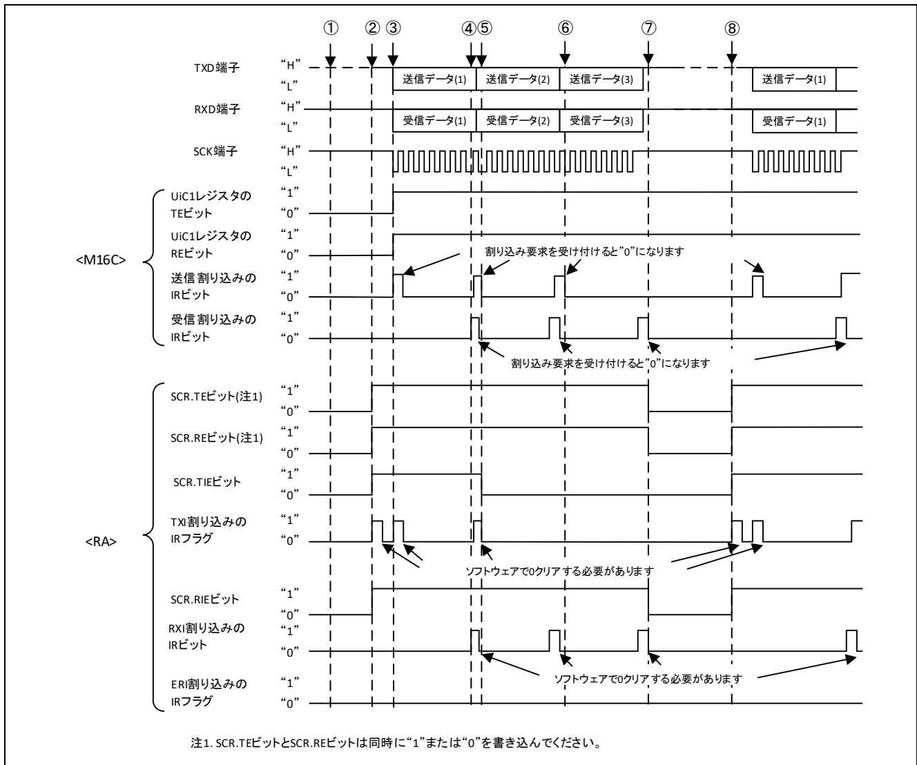
図 3-1 RA ファミリと M16C ファミリの送受信タイミング相違点(3 バイトずつ送受信する場合)
