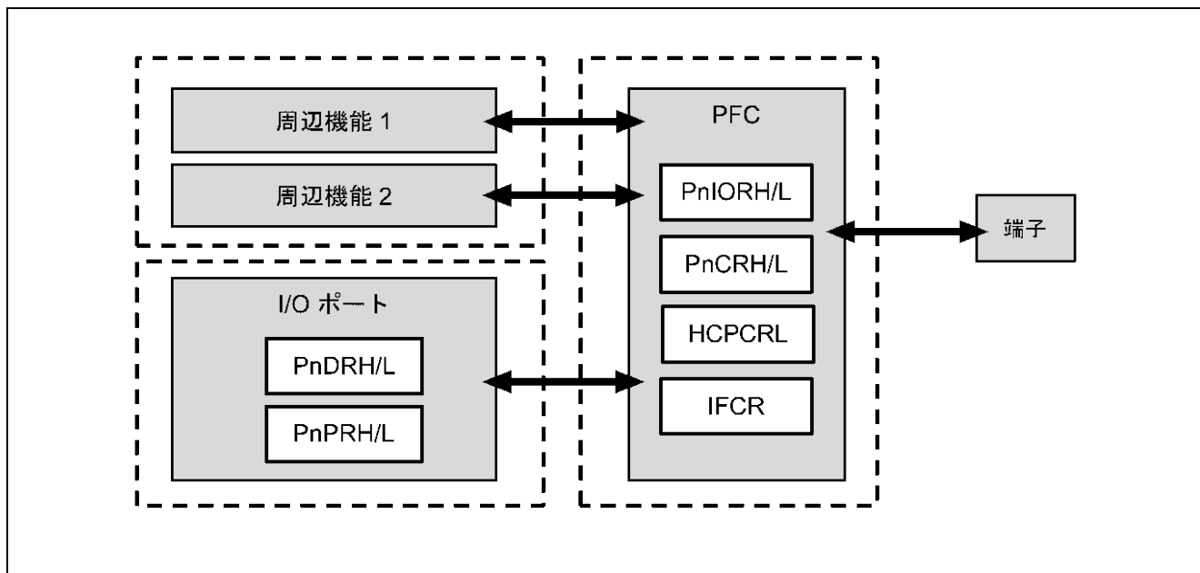
図 3.1 SH7080 グループ I/O 設定
