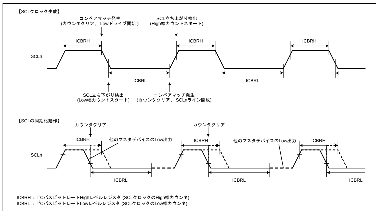
図 3.5 SCL クロック生成および SCL 同期化動作
