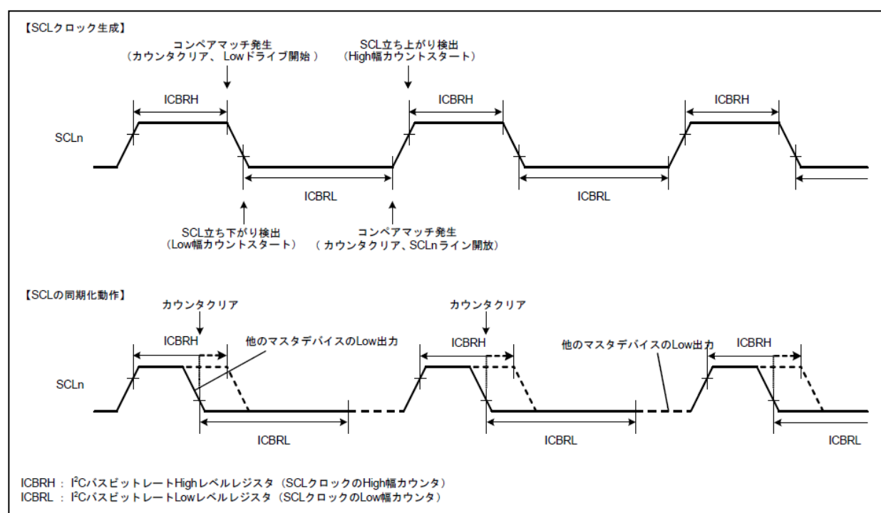
図 3-5 SCL クロック生成および SCL 同期化動作
