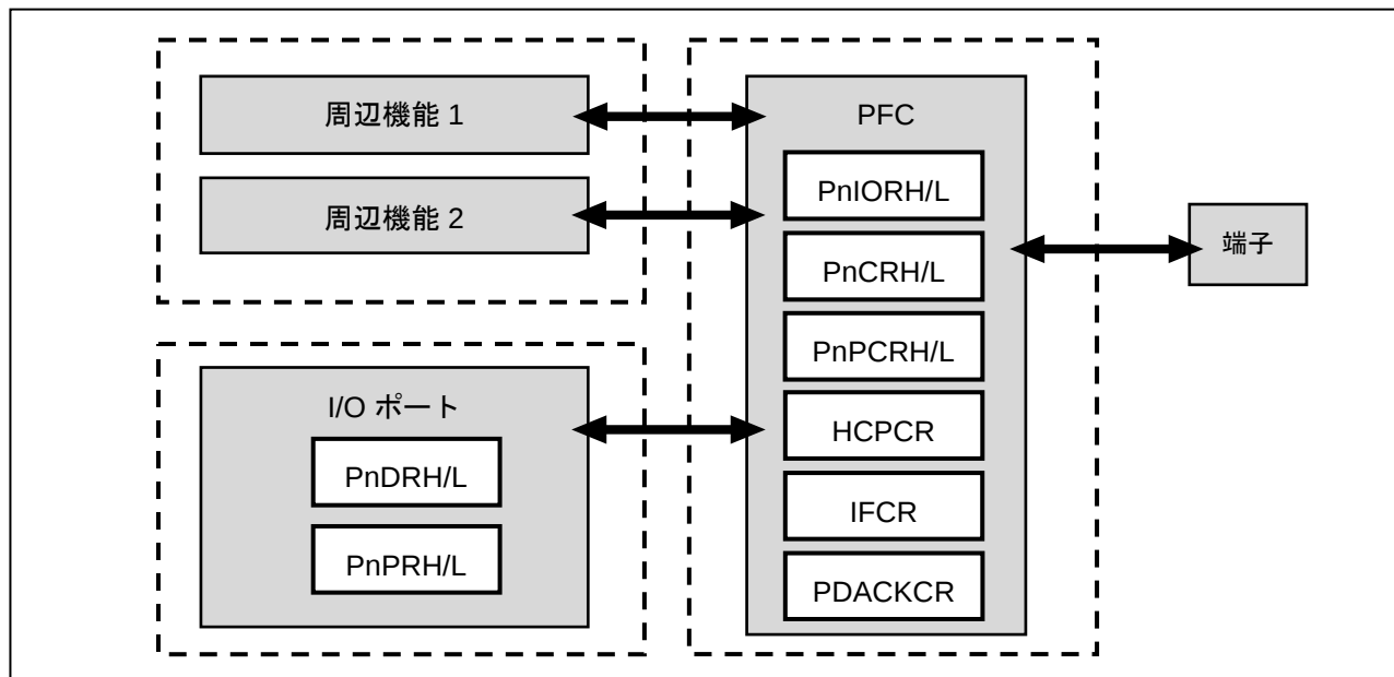
図 3-1 SH7216 グループ I/O ポートのブロック図
