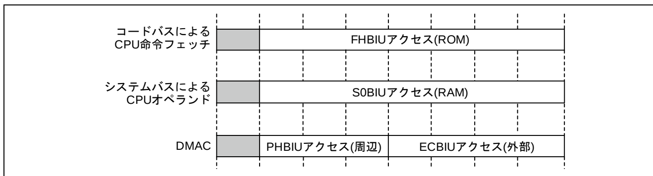
図 3-3 RA6M5 グループのバスの並列動作
