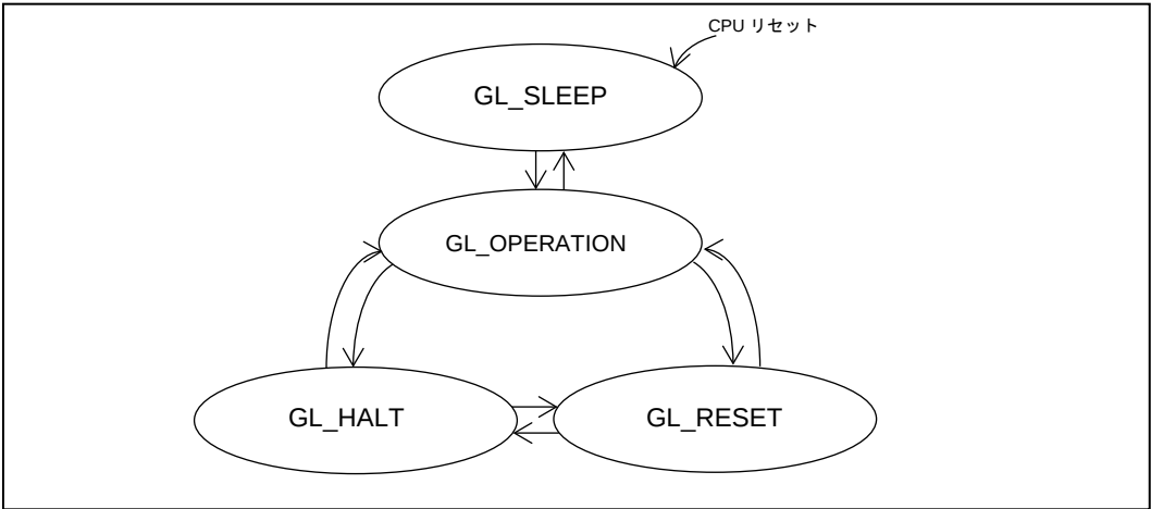
図 3-9 RA6M5 グループ グローバルモード間の状態遷移
