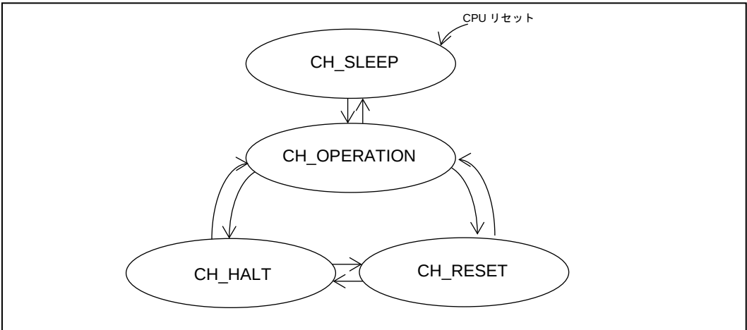
図 3-10 RA6M5 グループ チャネルモード間の状態遷移
