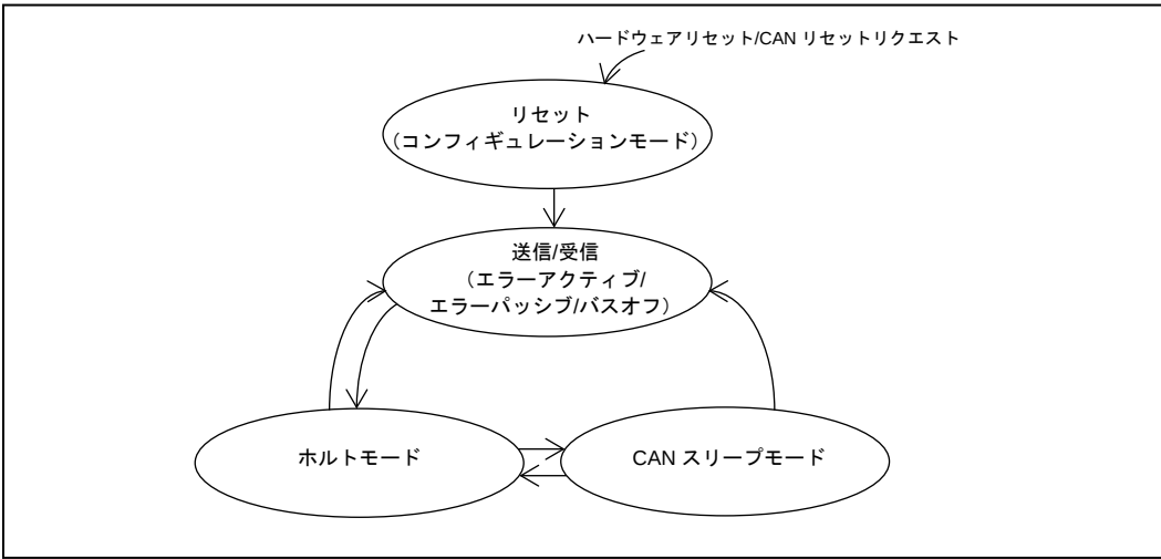
図 3-8 SH7216 状態遷移
