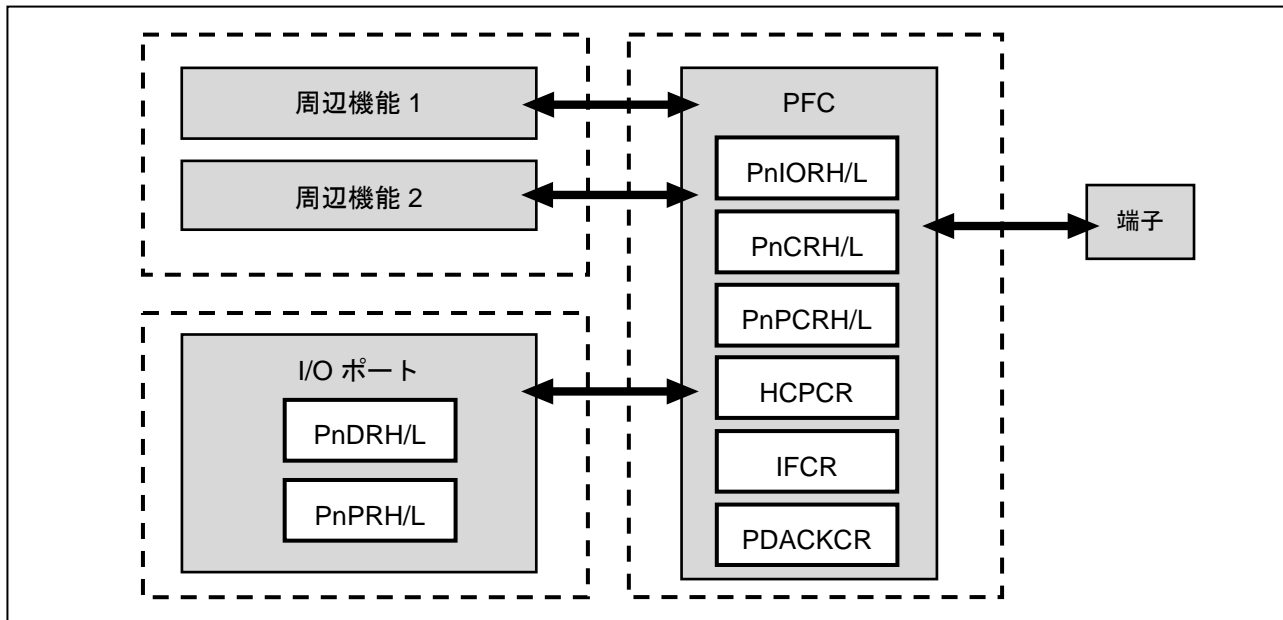
図 3-1 SH7216 グループ I/O ポートのブロック図
