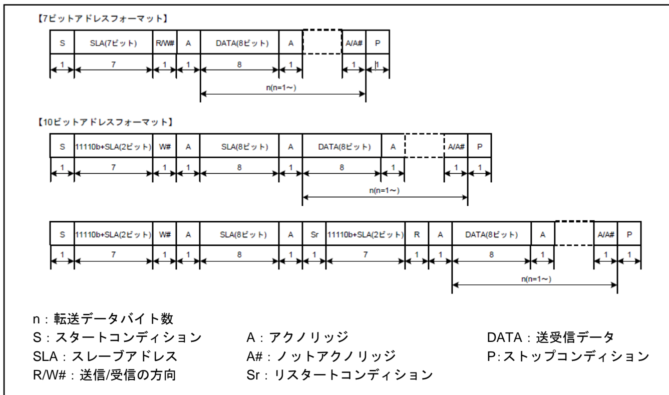
図 3-4 RA6M5 グループ I 2 C バスフォーマット
