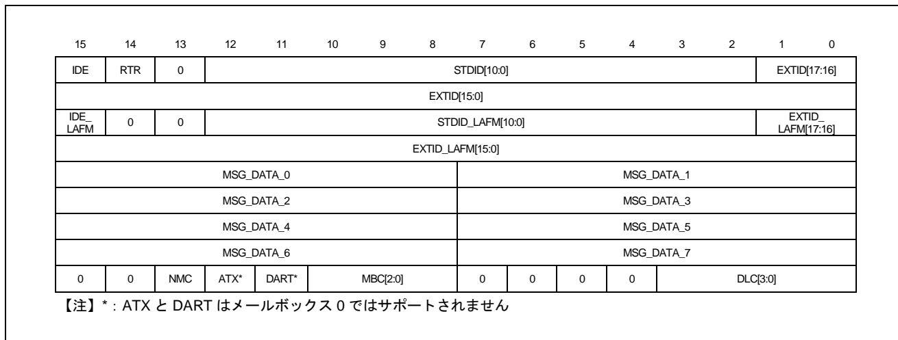
図 3-6 SH7216 グループのメールボックス構成
