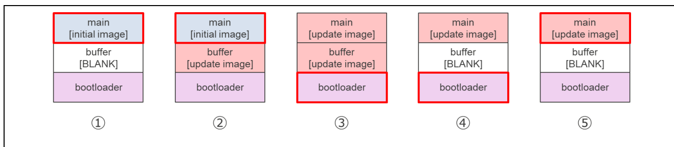
図 4-2 アップデート実行中のセカンダリ MCU の ROM の状態
