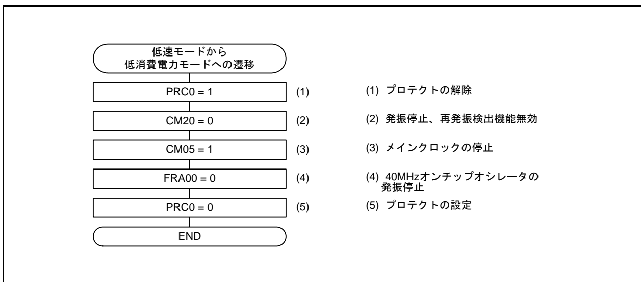
図3.4 低速モードから低消費電力モードに遷移する手順
