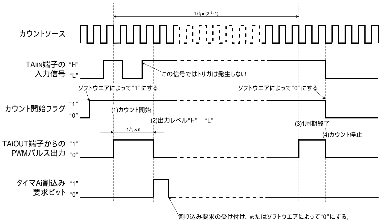
図 1 パルス幅変調モード動作、16 ビット PWM モード選択時のタイミング
