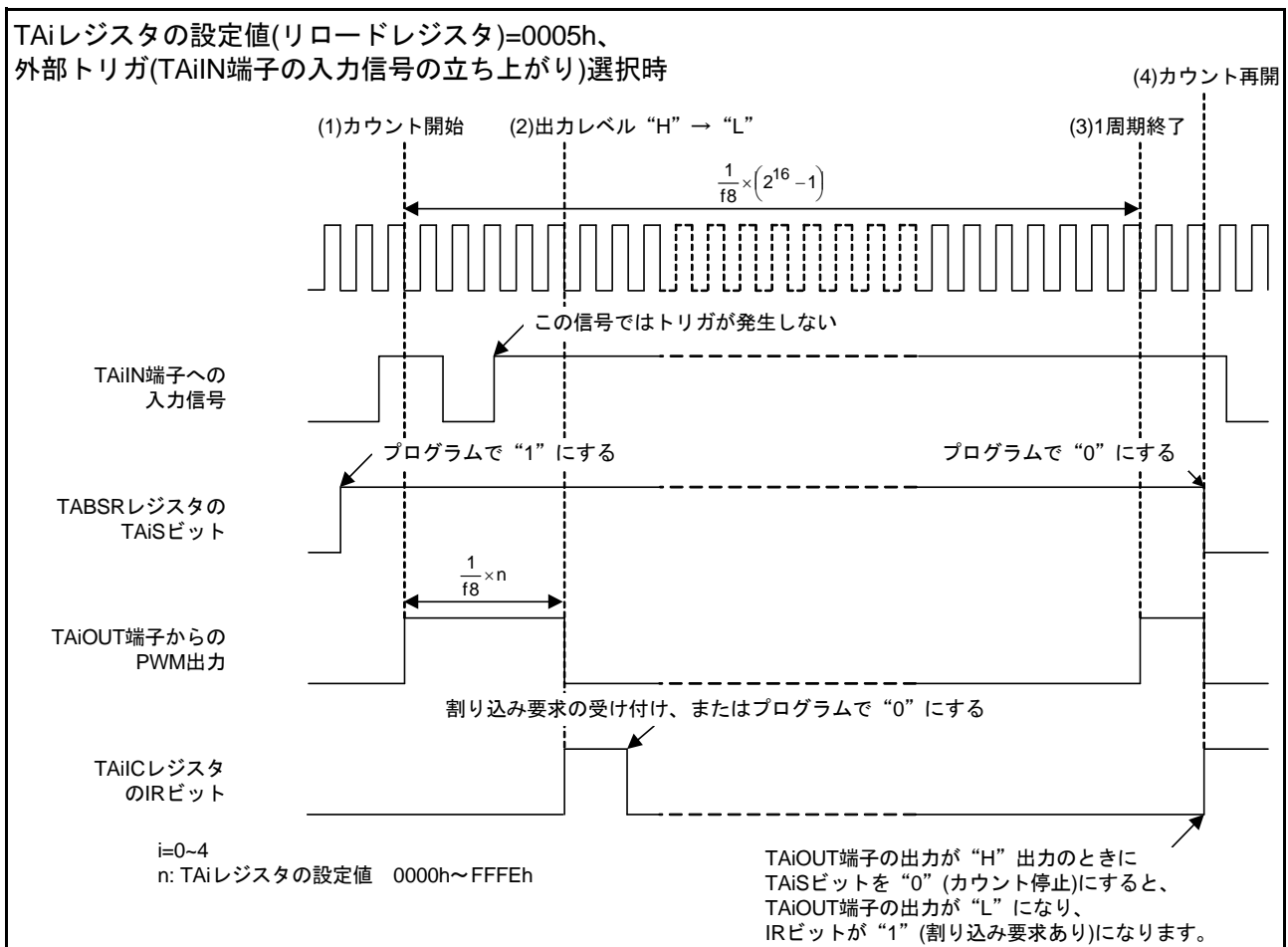
図 3.1 パルス幅変調モード(16ビットPWM)の動作
