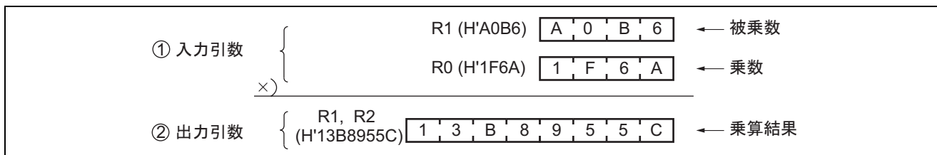
図 2 ソフトウェア MUL の実行例
