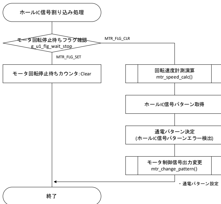
Figure 3-9 フローチャート(ホール IC 信号割り込み処理)
