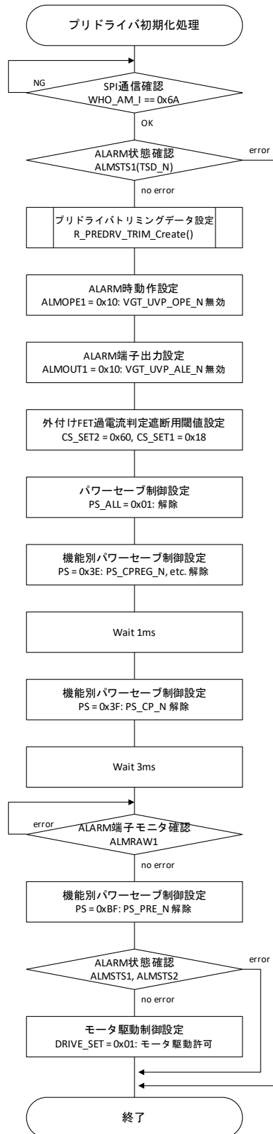
Figure 3-8 フローチャート(プリドライバ初期化処理)
