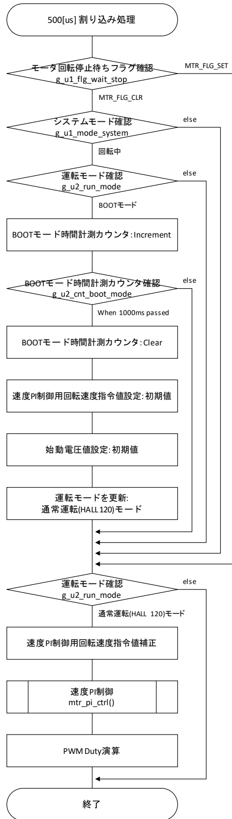
Figure 3-11 フローチャート(500[us] 割り込み処理)
