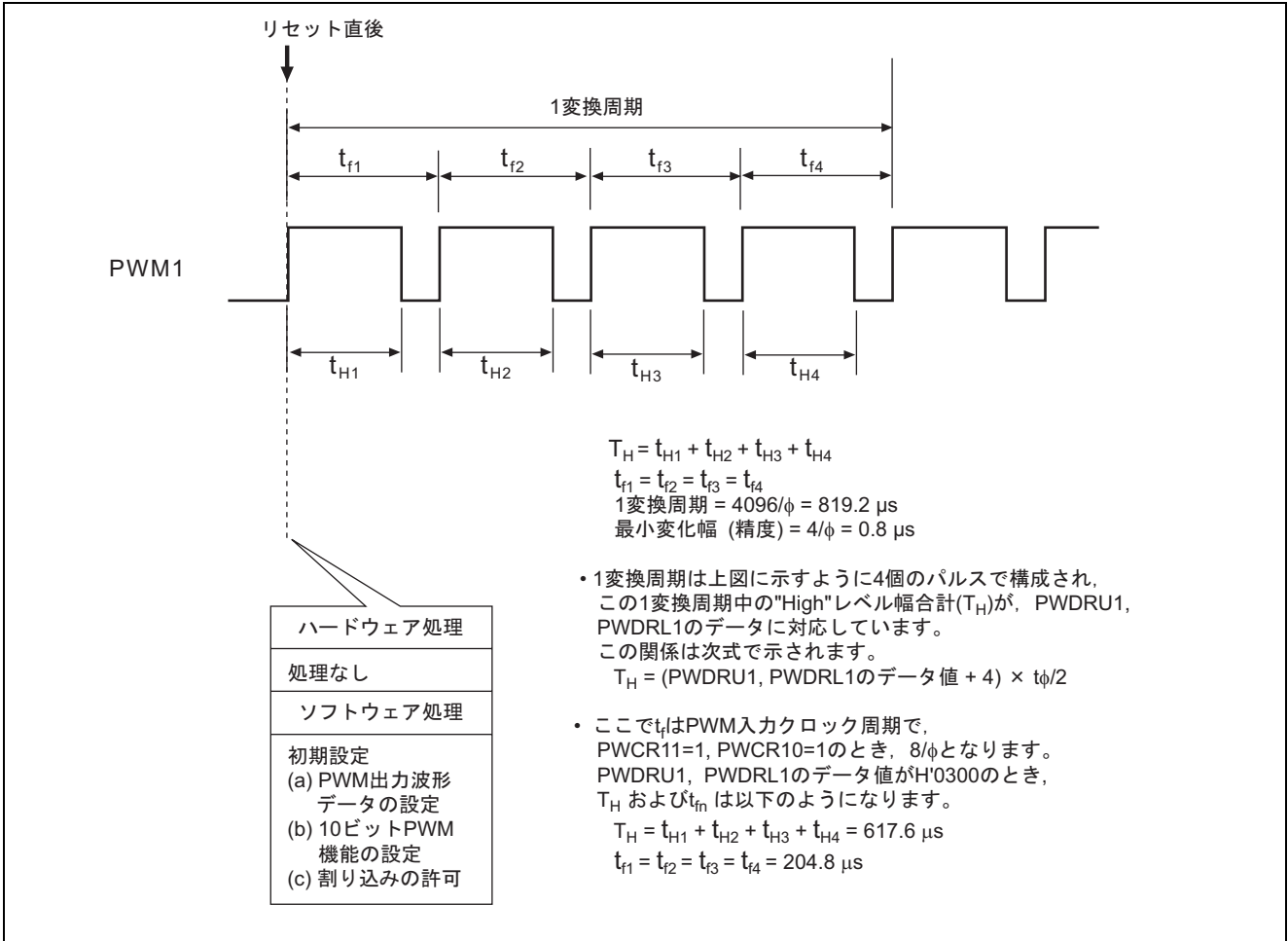
図3 10ビットPWM機能によるデューティパルス出力動作説明
