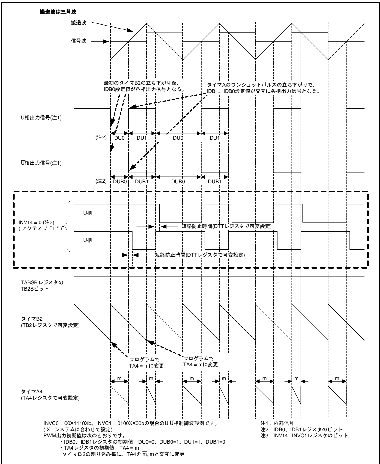
図 3.1 三角波変調(三相モード0)動作タイミング
