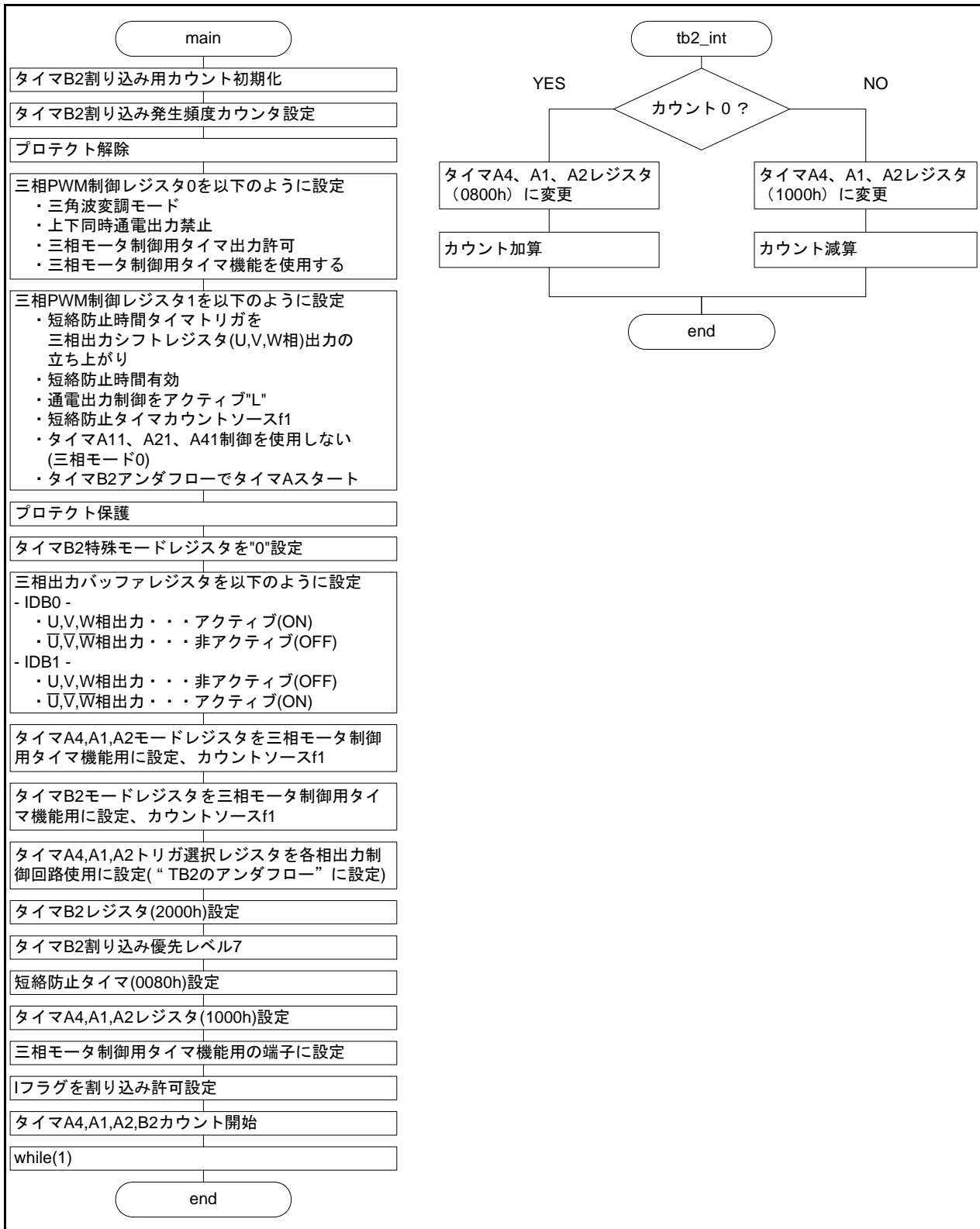
図 4.1 三角波変調（三相モード0）・フローチャート図
