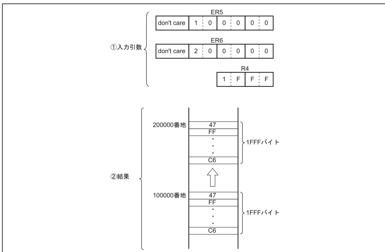
図1 ソフトウェアEEPROMの実行例
