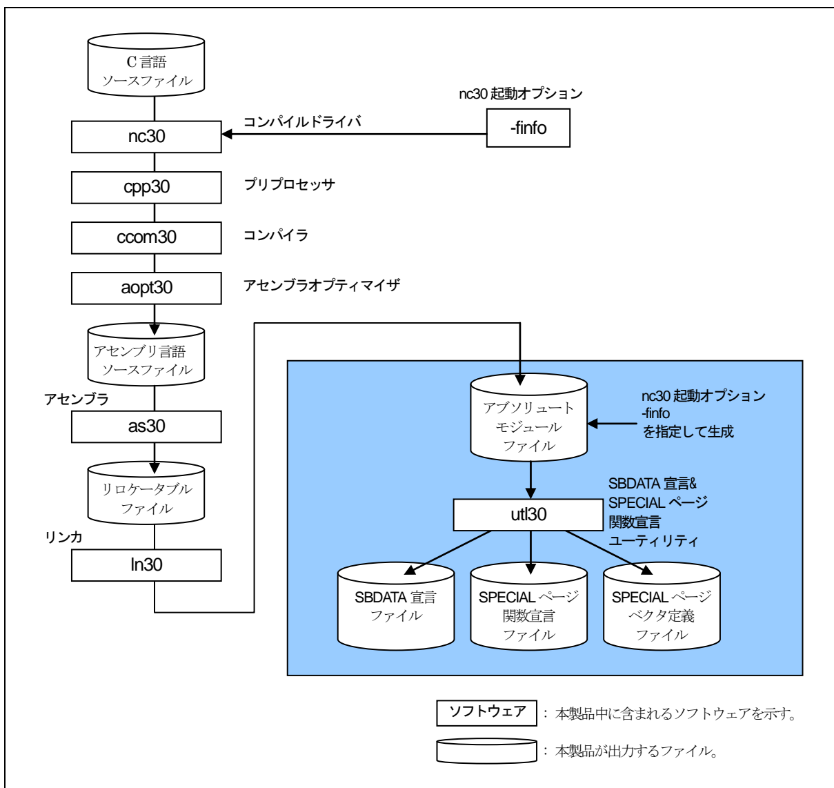
図G.1 NC30 の処理フロー
