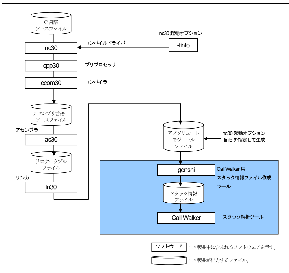
図H.1 NC30 の処理フロー
