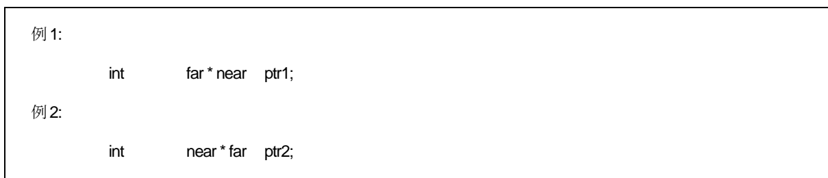
図B.8 アドレスを扱うポインタ型変数の宣言例(2)
