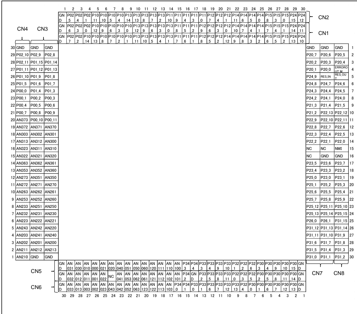
図 2-3 ピンヘッダのアサイン
