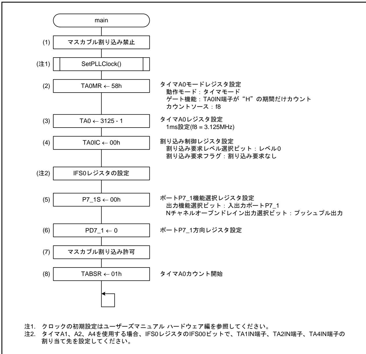
図 3.2 メイン関数のフローチャート
