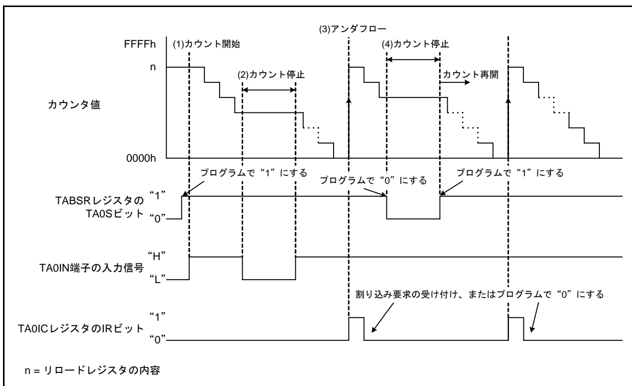
図 3.1 タイマモード、ゲート機能選択時の動作タイミング
