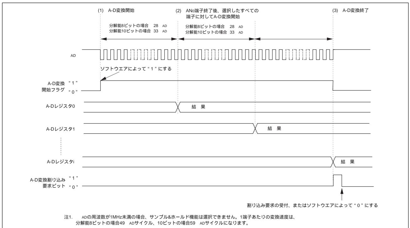
図1 単掃引モード動作タイミング
