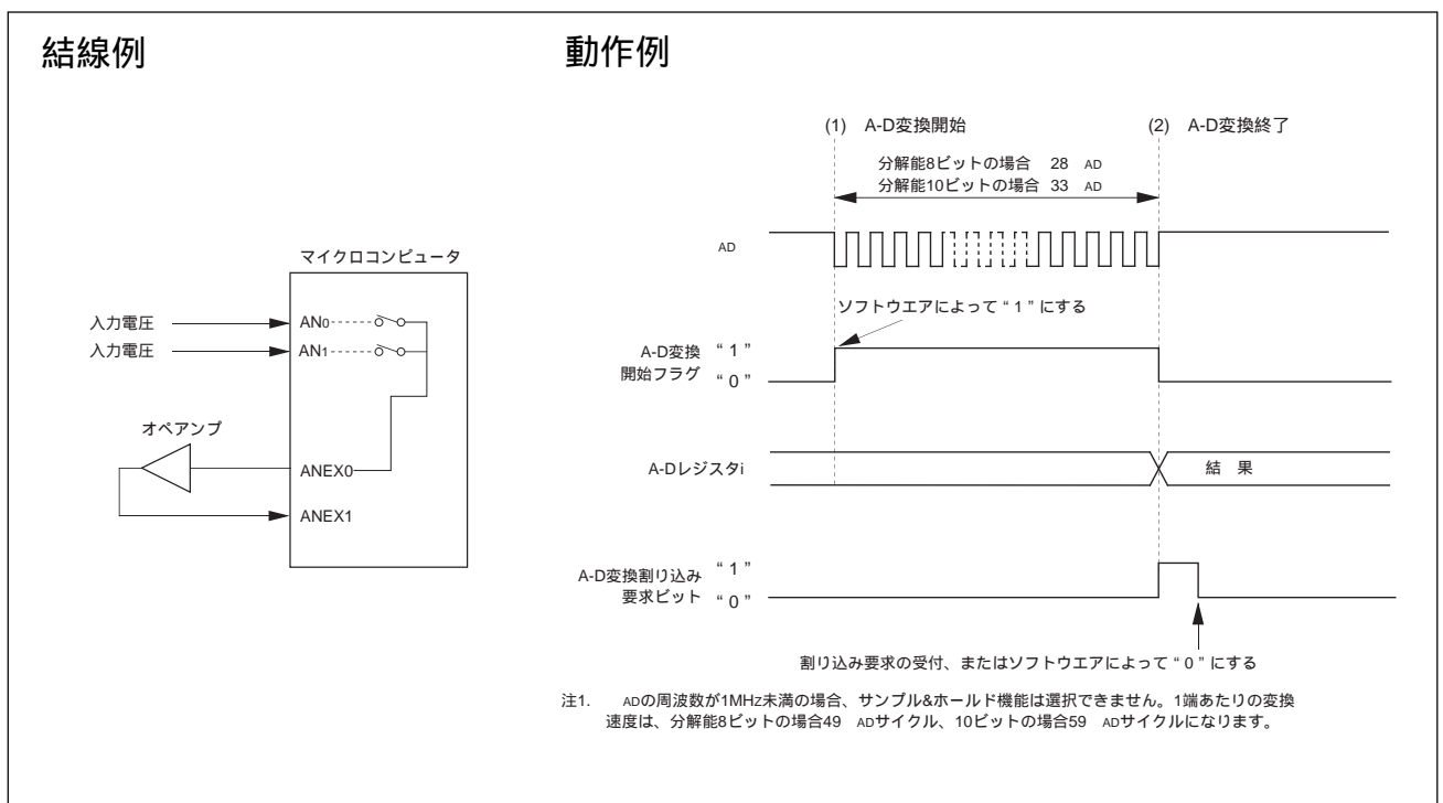
図1 単発モード、外部オペアンプ接続モード選択時の動作タイミング
