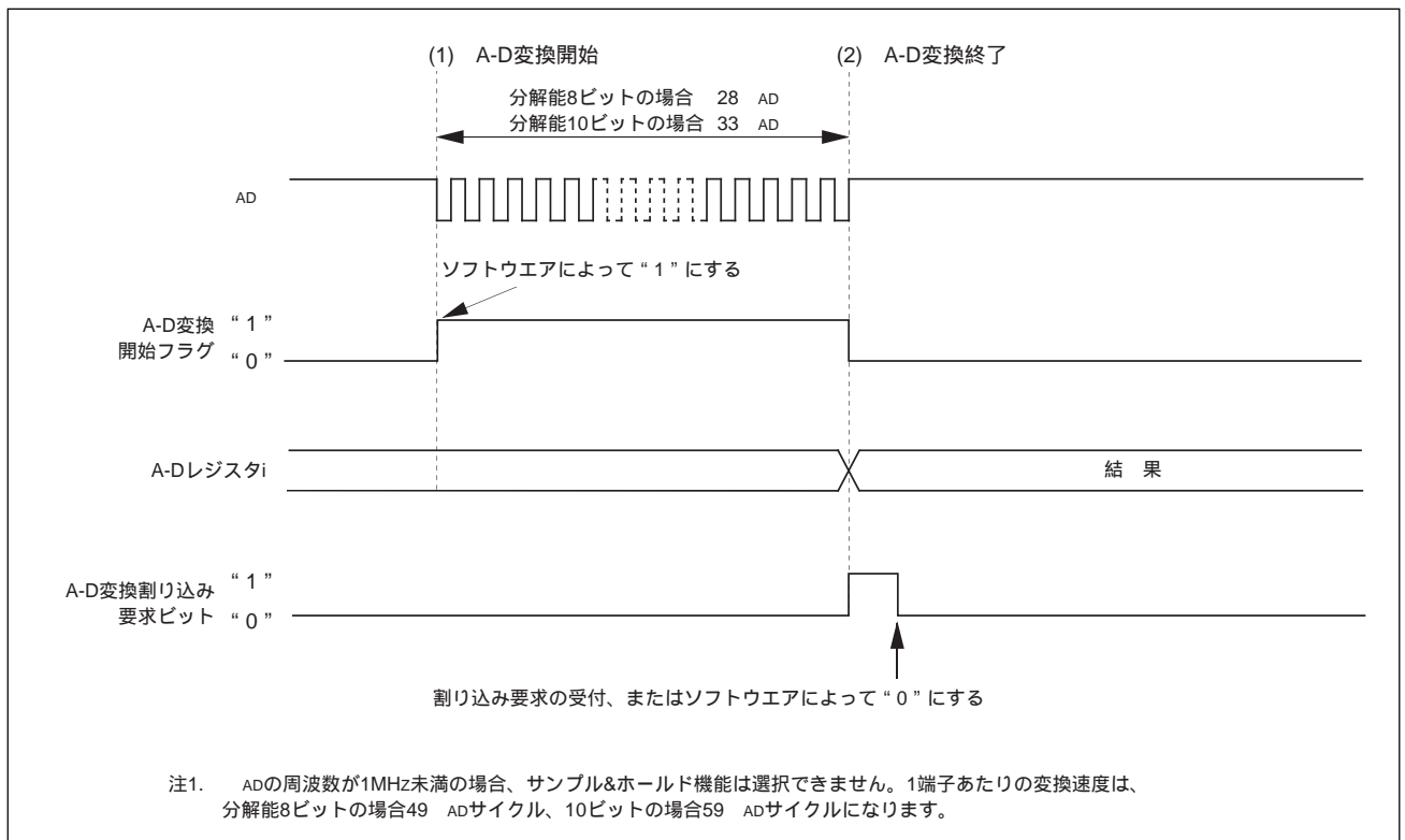
図1 単発モード動作タイミング
