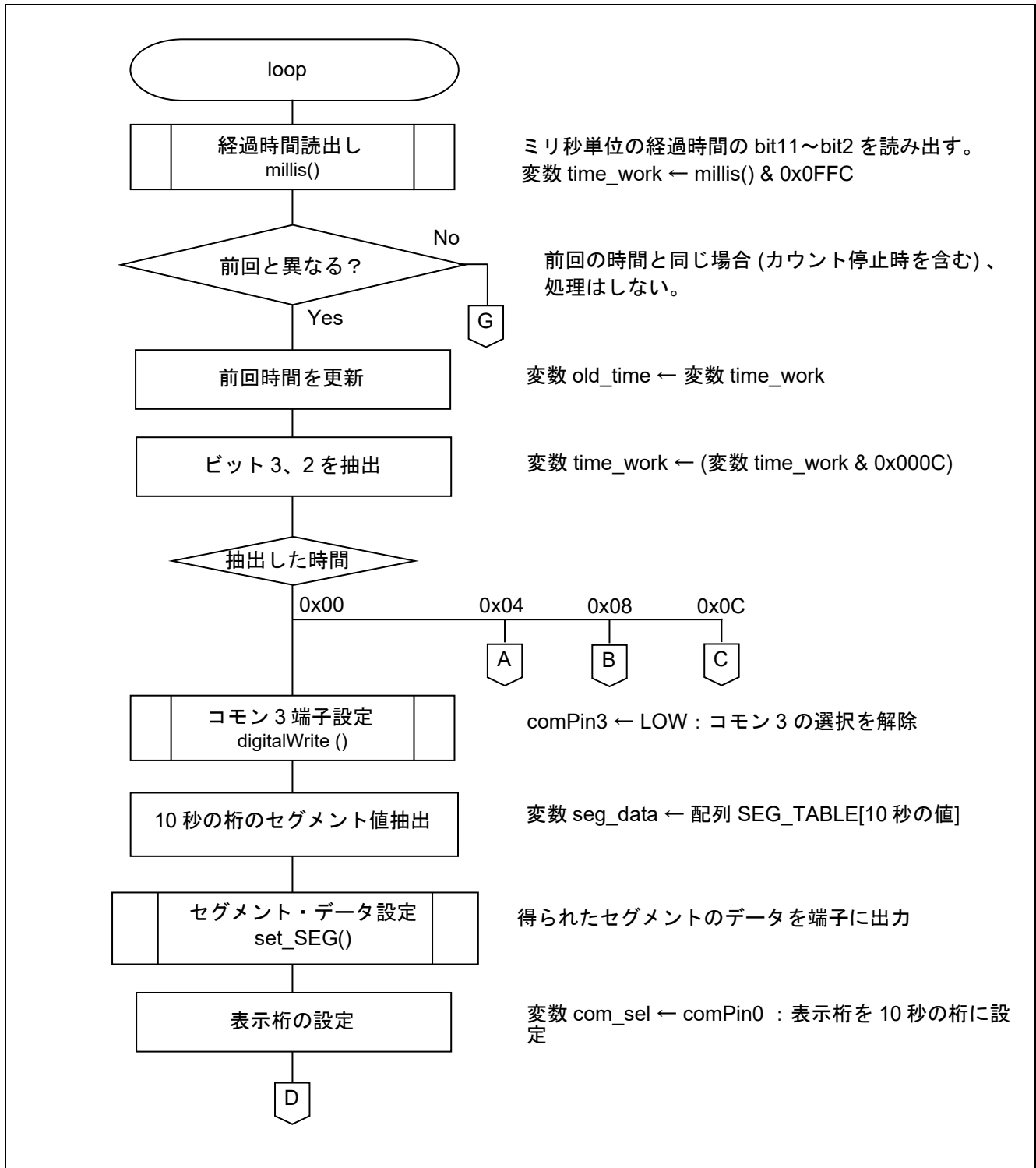
図 5.3 メイン関数 (1/4)
