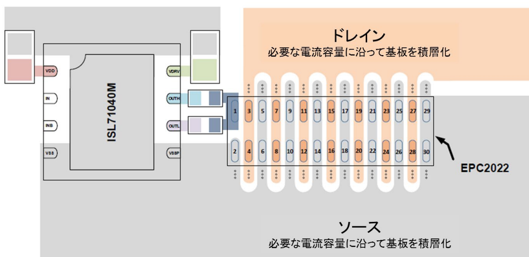
図4- ゲート駆動ループのインダクタンスを最小にするための最適化されたレイアウト：ゲートループは可能な限り太く短くする。最小化するパスは、VDRV（緑）から OUTH（青）を通過してゲート（濃い青）へ、そして OUTL（紫）を通過して VSSP（灰色）に戻る経路です。
