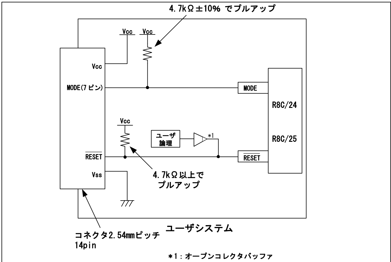
図 5.1 E8 の接続例
