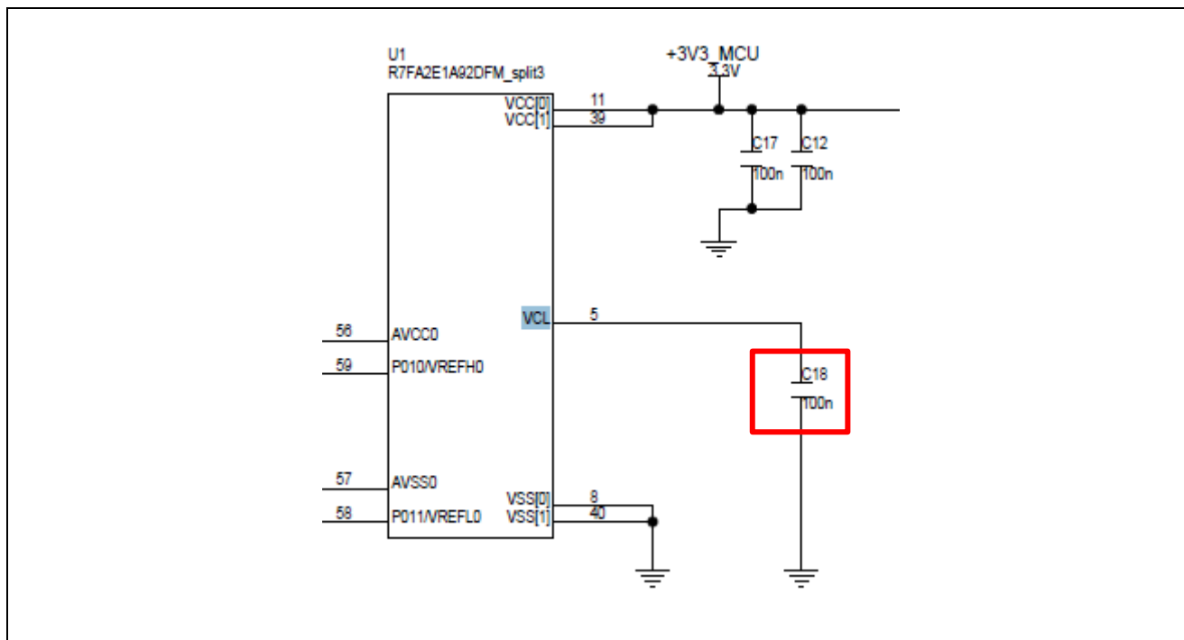
図 2 MCU VCL 端子のコンデンサ値の違い
