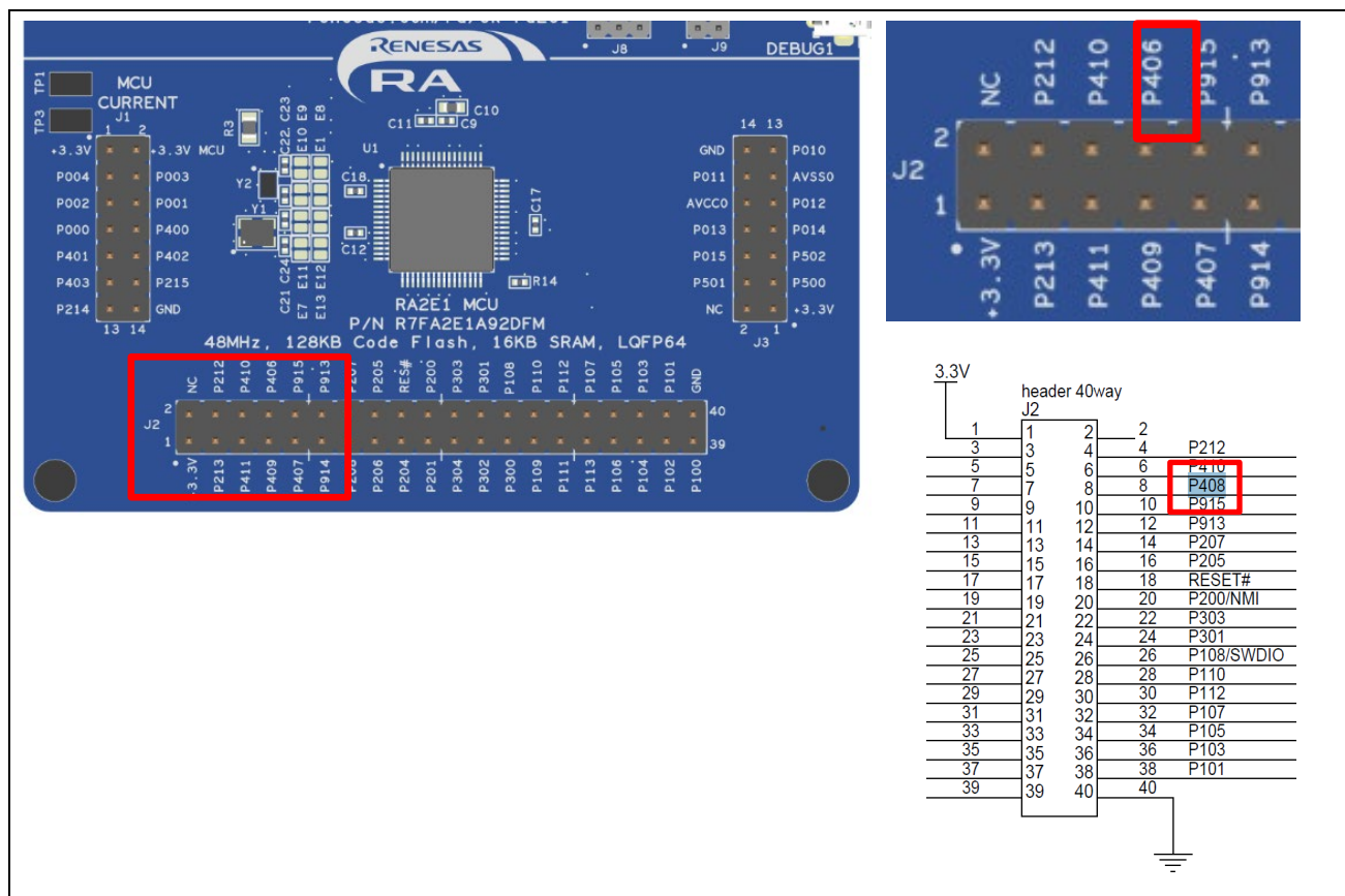
図 3 MCU ピンヘッダ J2 8 ピンのシルク表示の間違い
