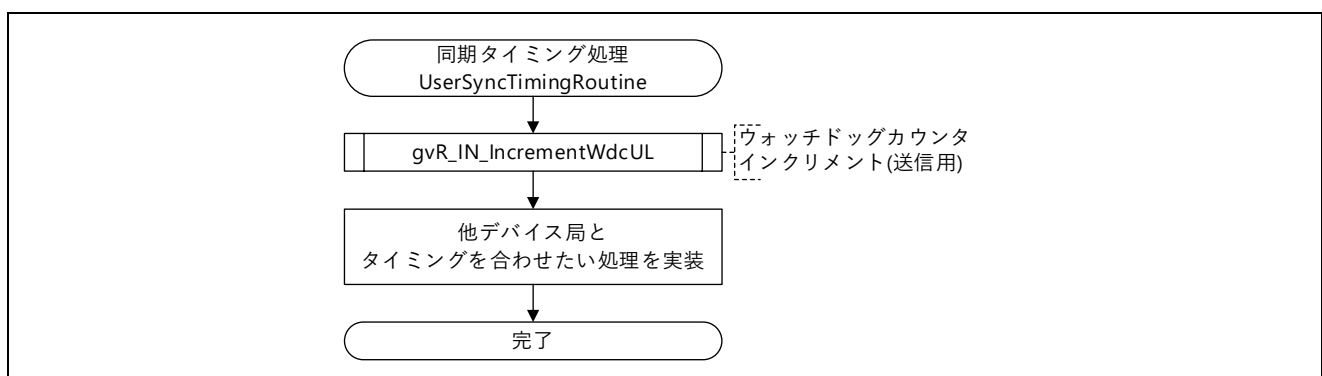
図 5.8 同期タイミング処理フロー図
