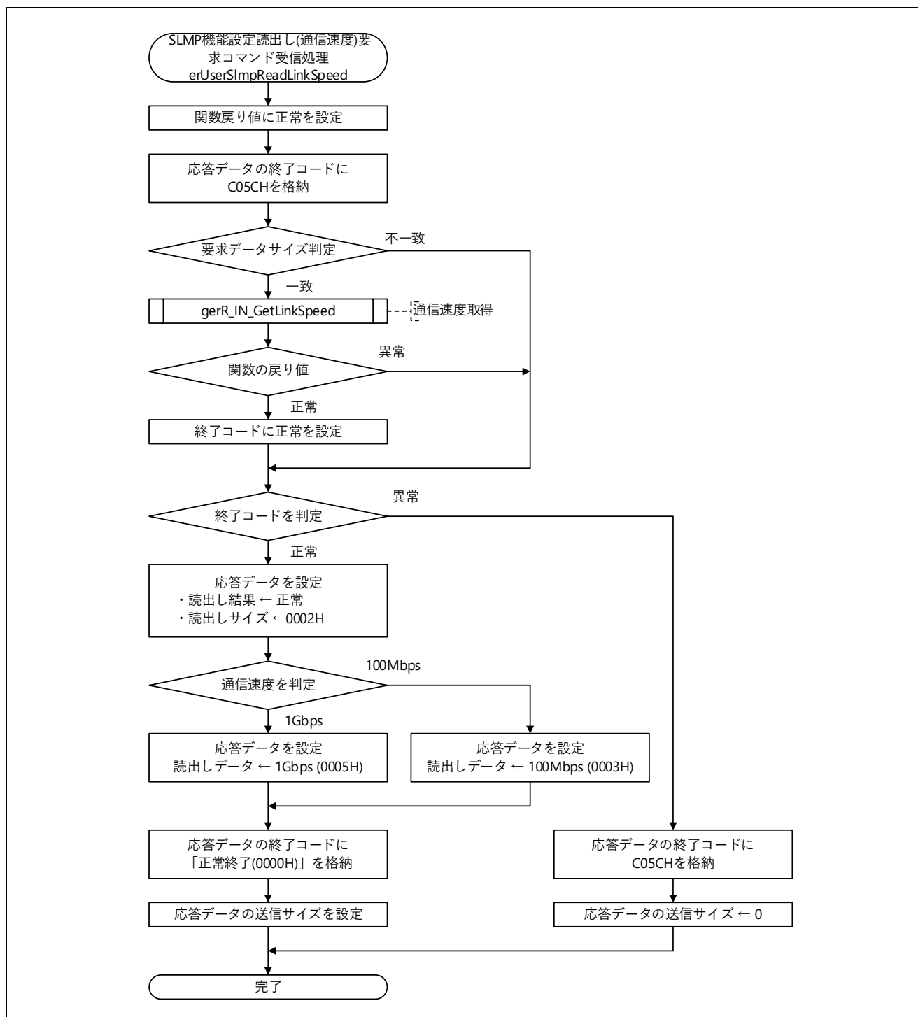
図 5.66 SLMP 機能設定読出し(通信速度)要求コマンド受信処理フロー図
