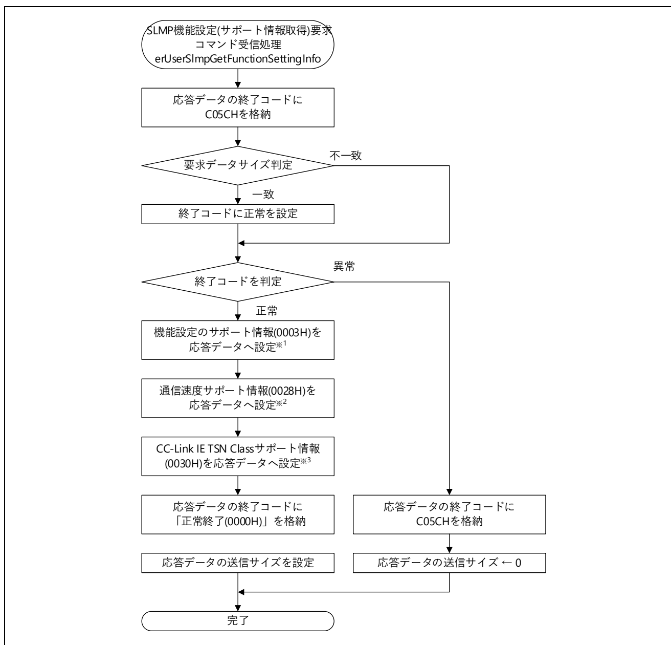
図 5.65 SLMP 機能設定(サポート情報取得)要求コマンド受信処理フロー図
