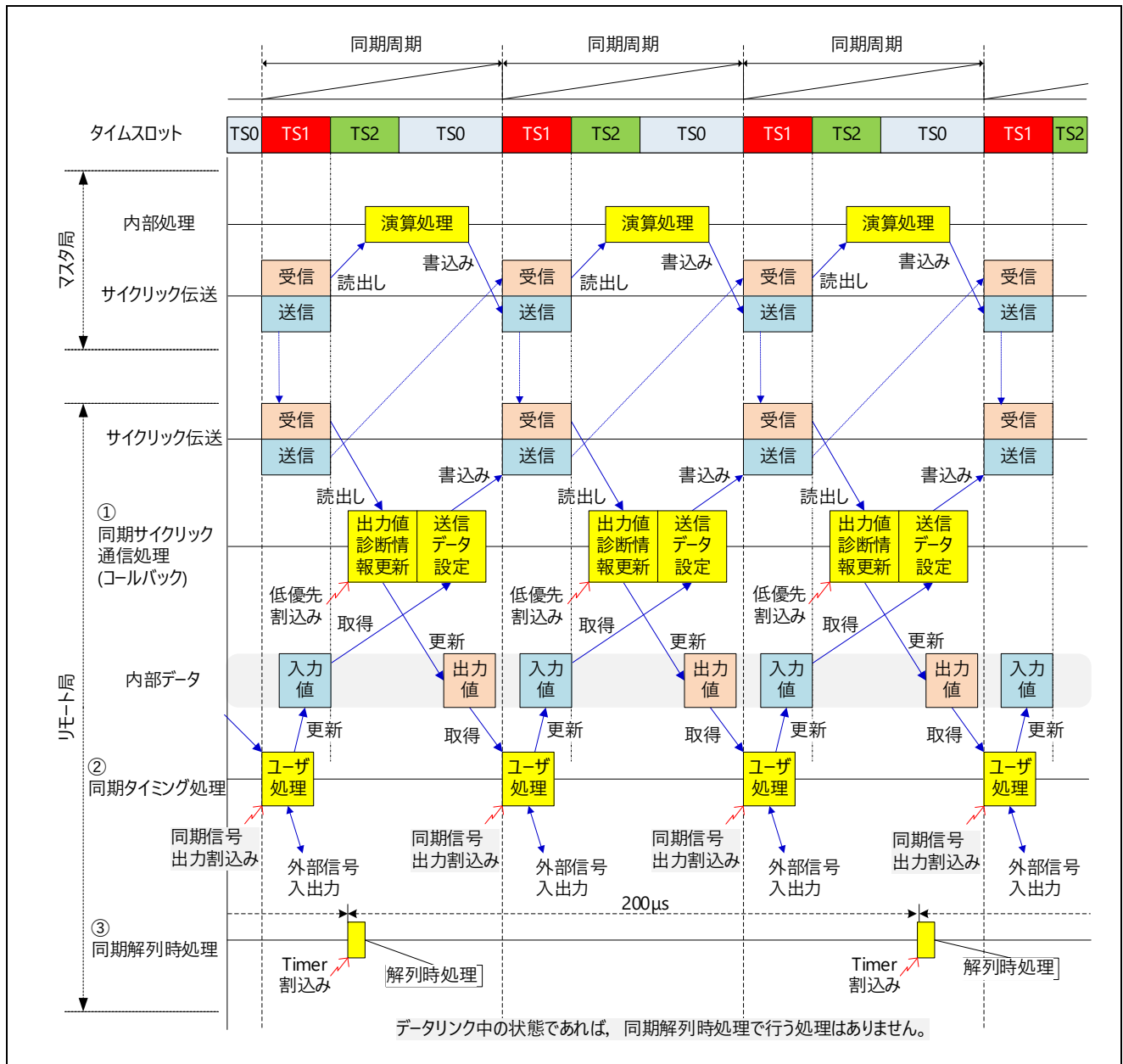
図 4.9 同期通信のタスク/処理タイミングチャート(データリンク中)
