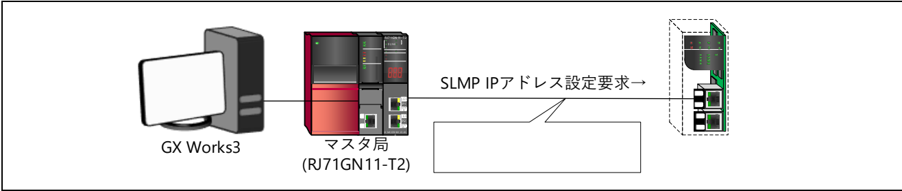
図 4.15 デバイス局の IP アドレス設定イメージ
