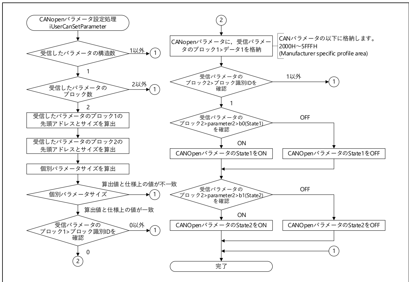
図 5.83 CANopen パラメータ設定処理フロー図
