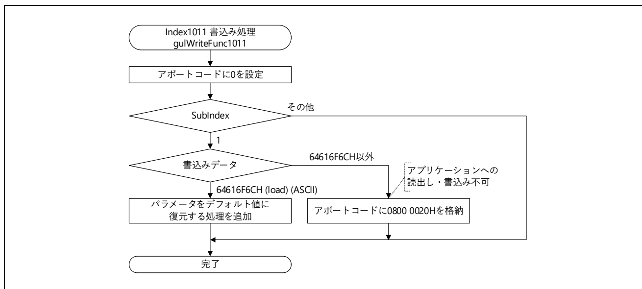
図 5.85 Index1011 書込み処理フロー図
