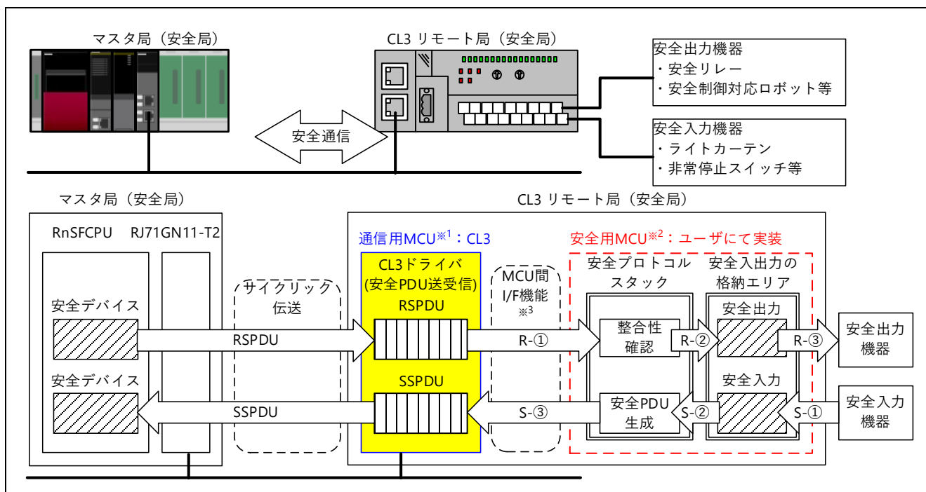
図 4.13 安全通信イメージ
