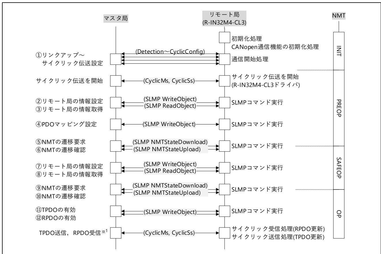
図 5.72 CANopen 通信時の初期化シーケンス(概略)
