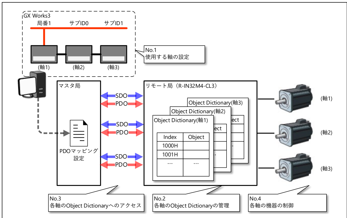
図 4.12 CANopen 通信における増設ユニットのイメージ
