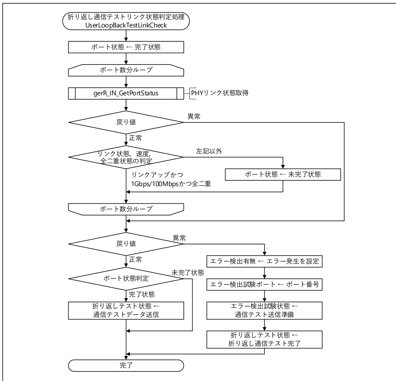
図 5.104 折り返し通信テストリンク状態判定処理フロー図
