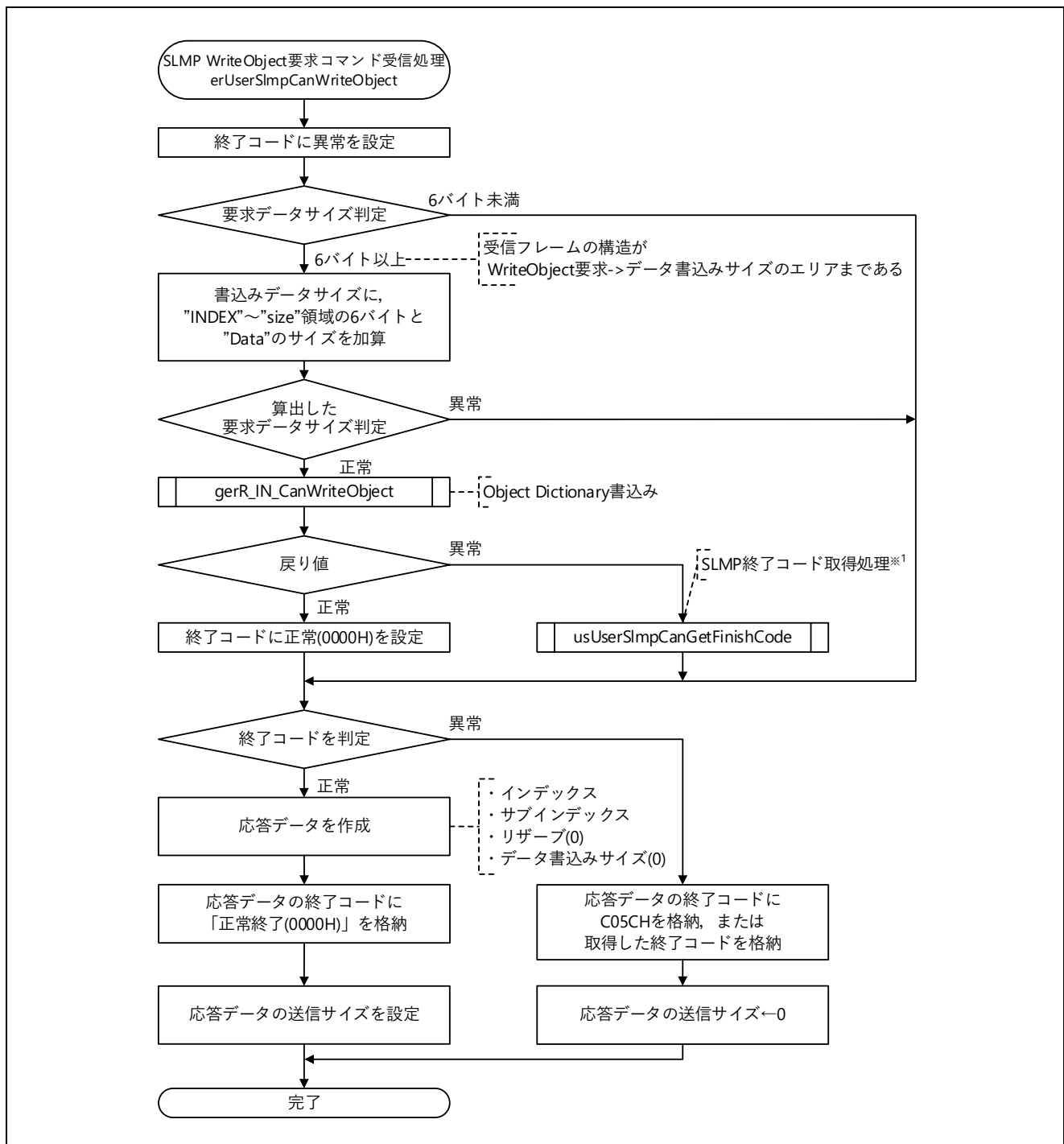
図 5.77 SLMP WriteObject 要求コマンド受信処理フロー図
