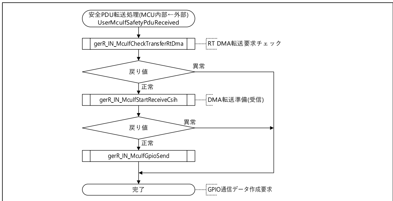
図 5.97 安全 PDU 転送処理(MCU 内部←外部)フロー図
