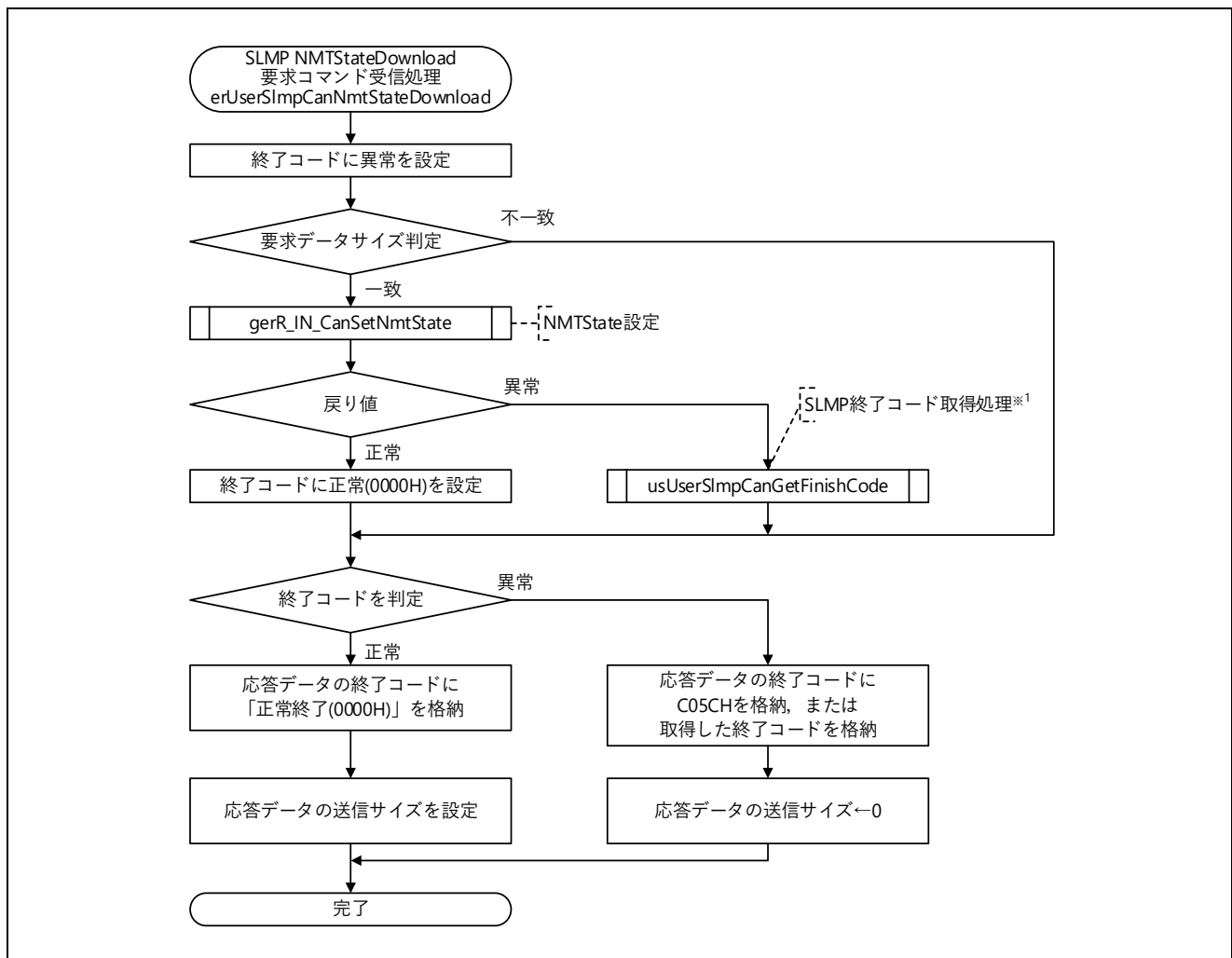
図 5.81 SLMP NMTStateDownload 要求コマンド受信処理フロー図
