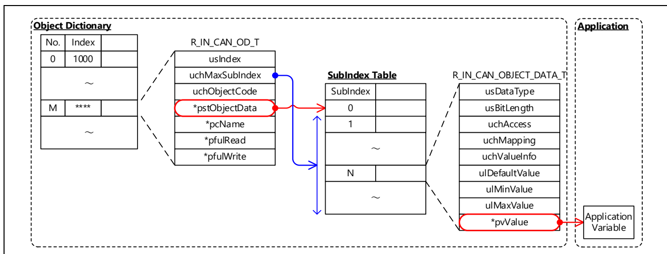
図 5.70 Object Dictionary のデータ構造イメージ
