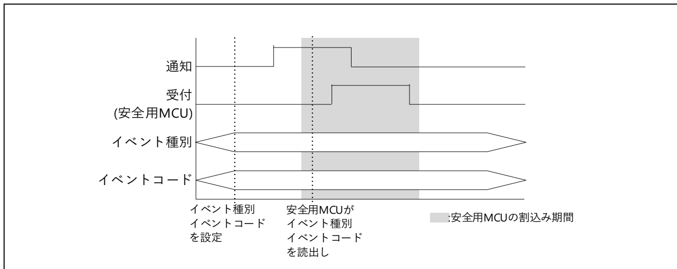
図 5.88 GPIO 通信のタイミング
