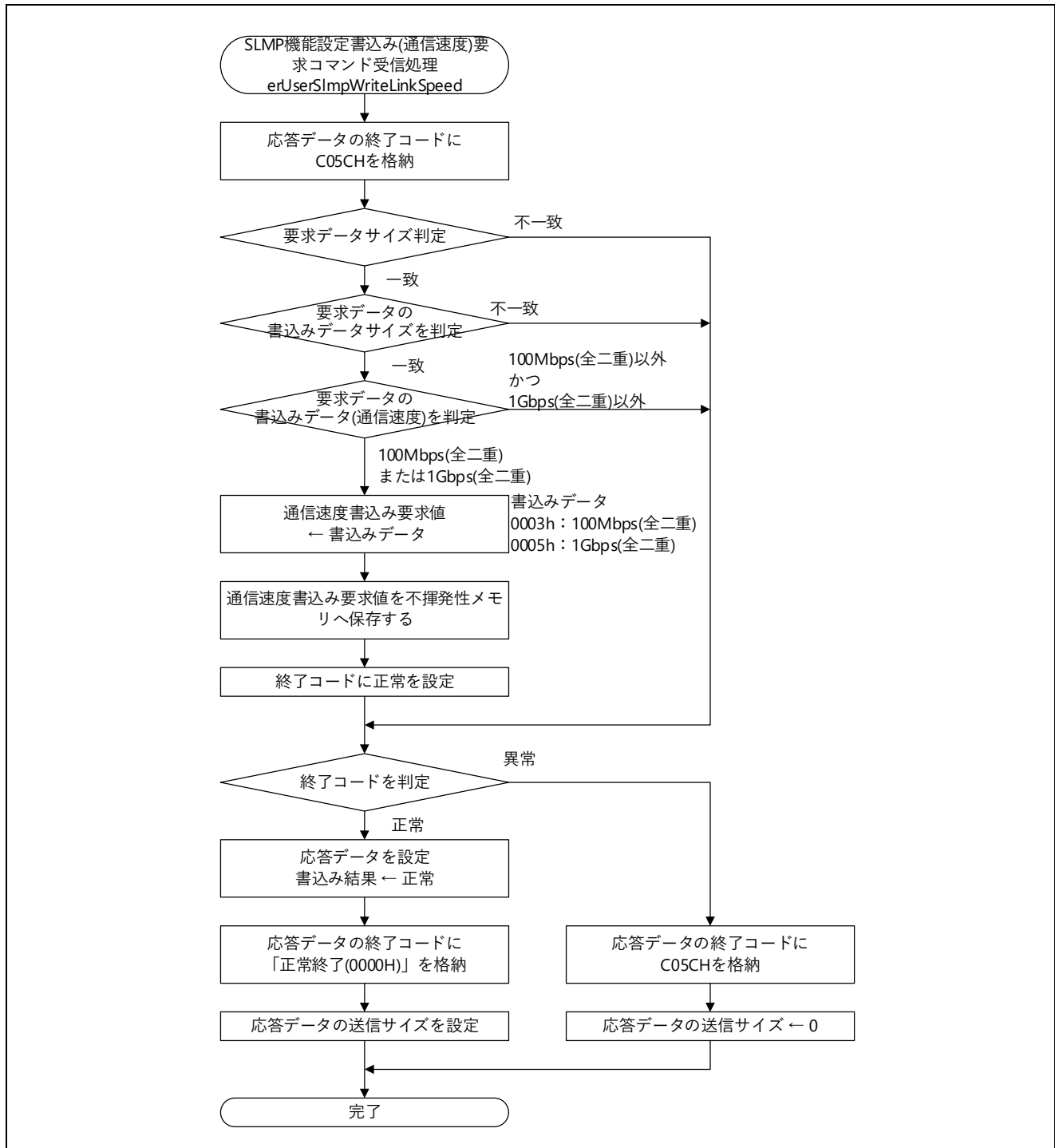
図 5.67 SLMP 機能設定書込み(通信速度)要求コマンド受信処理フロー図
