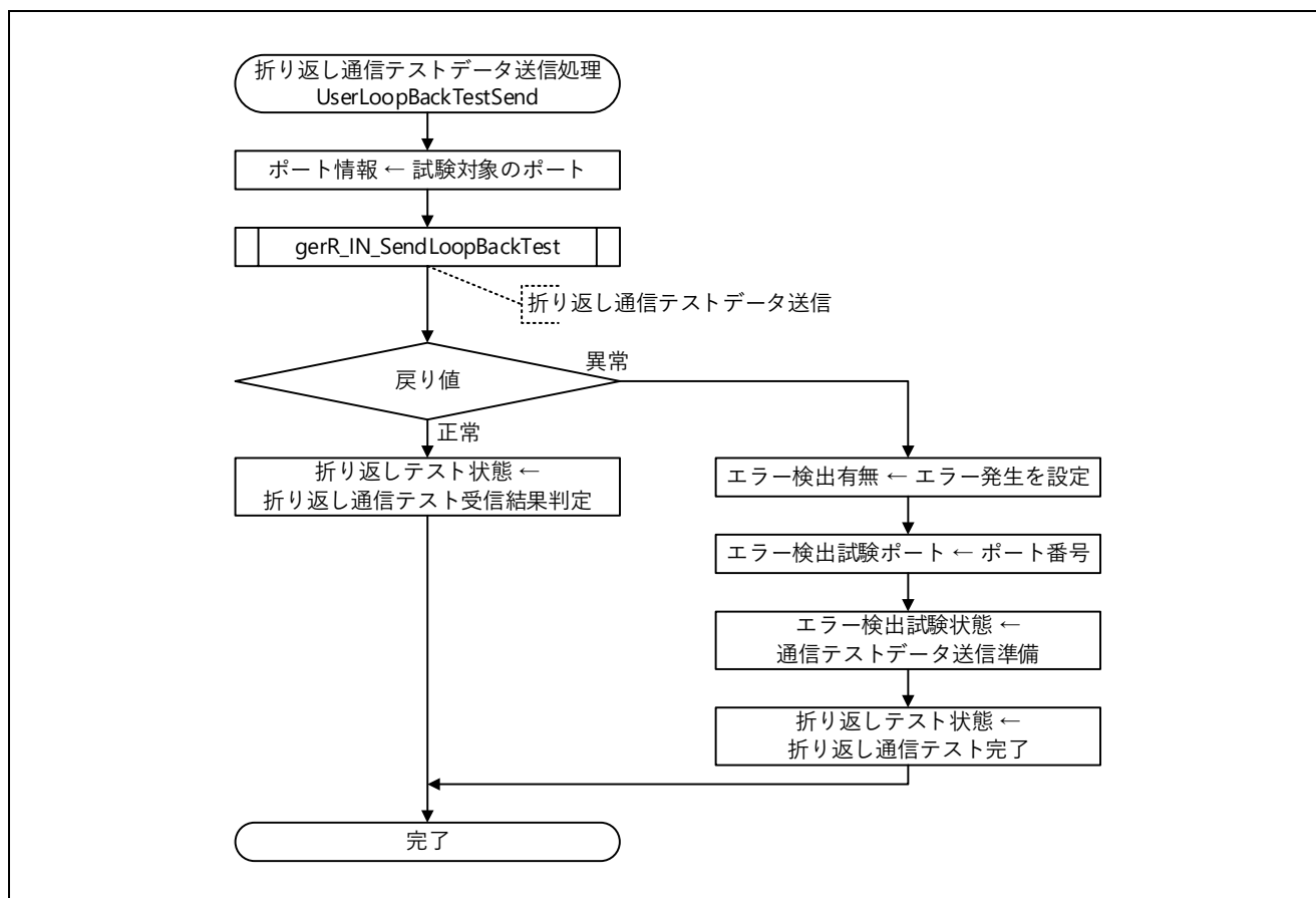
図 5.105 折り返し通信テストデータ送信処理フロー図
