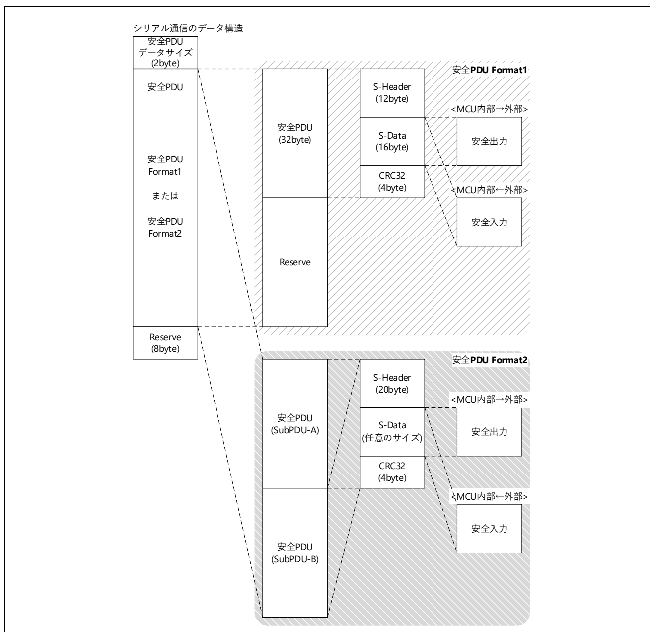
図 5.89 シリアル通信(RT DMA 転送)の安全 PDU 構造(概要)
