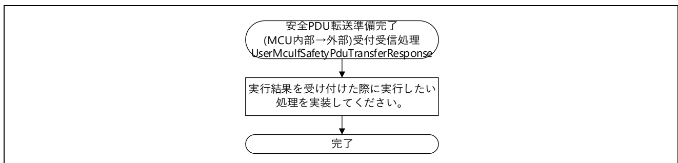
図 5.98 安全 PDU 転送準備完了(MCU 内部→外部)受付受信処理フロー図
