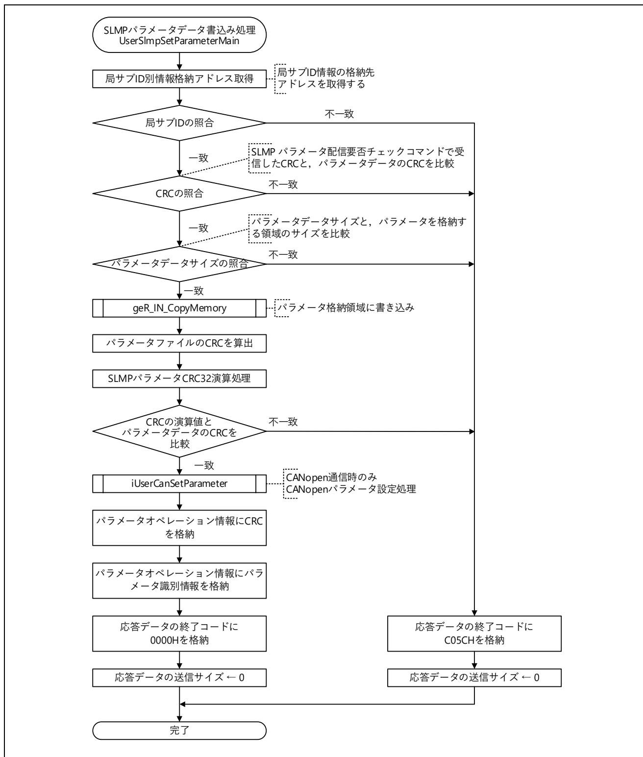
図 5.62 SLMP パラメータデータ書き込み処理フロー図
