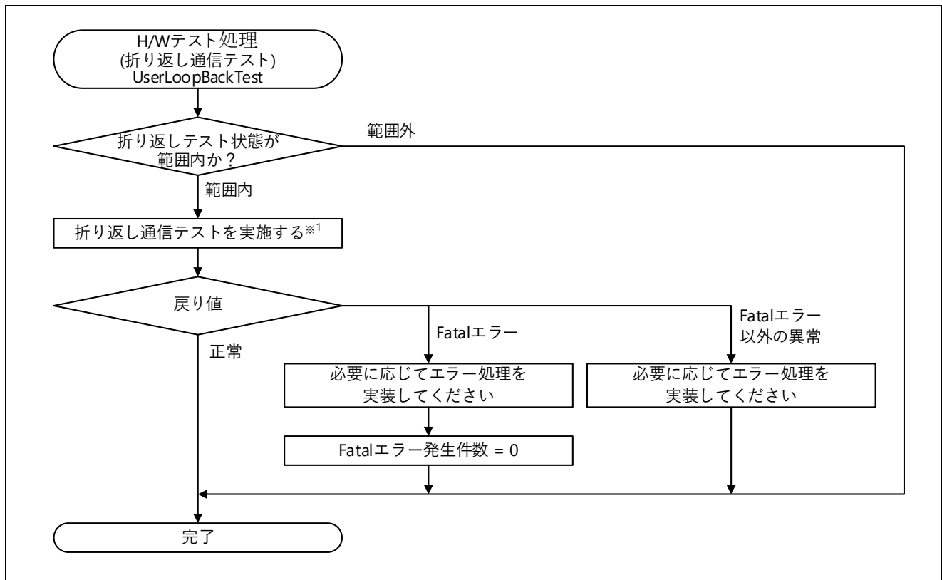
図 5.102 H/W テスト処理(折り返し通信テスト)処理フロー図
