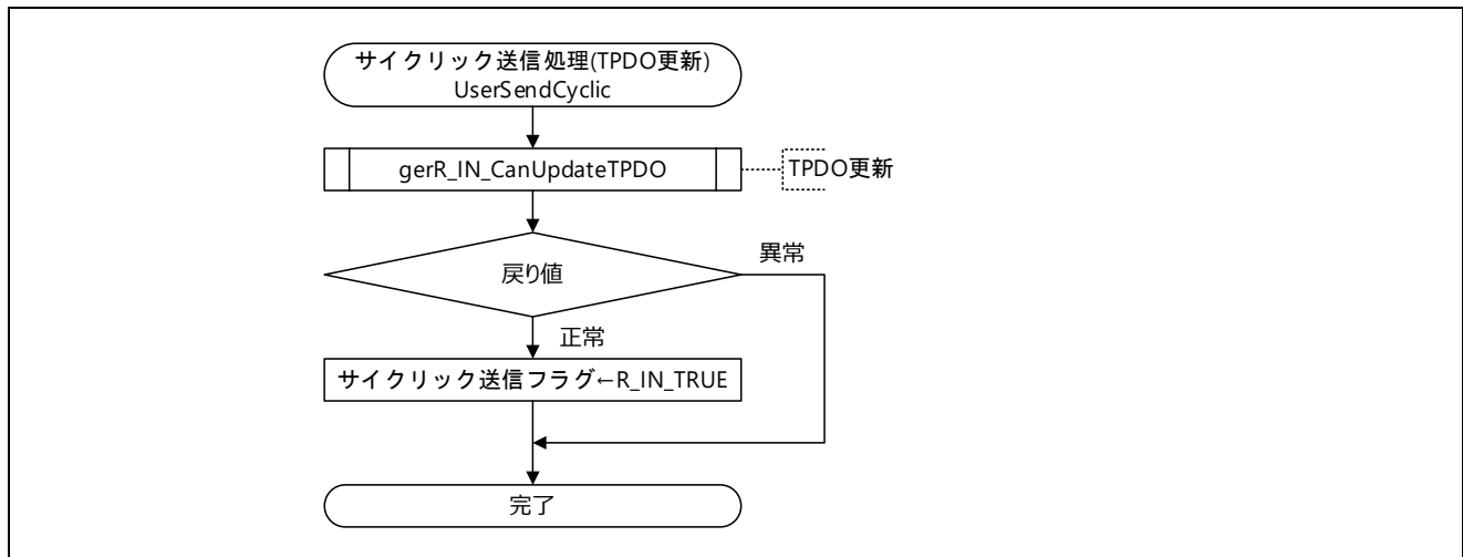
図 5.75 サイクリック送信処理(TPDO 更新)フロー図
