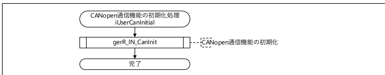
図 5.71 CANopen 通信機能の初期化処理フロー図
