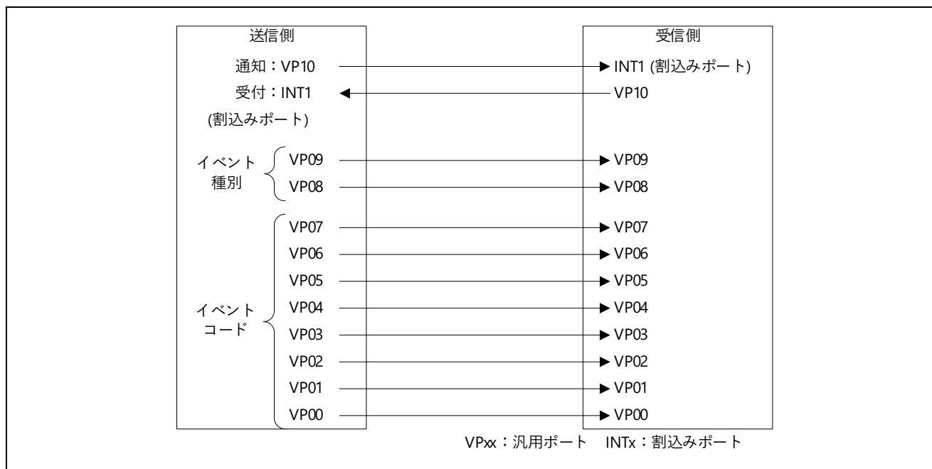
図 5.87 GPIO 通信の構成イメージ
