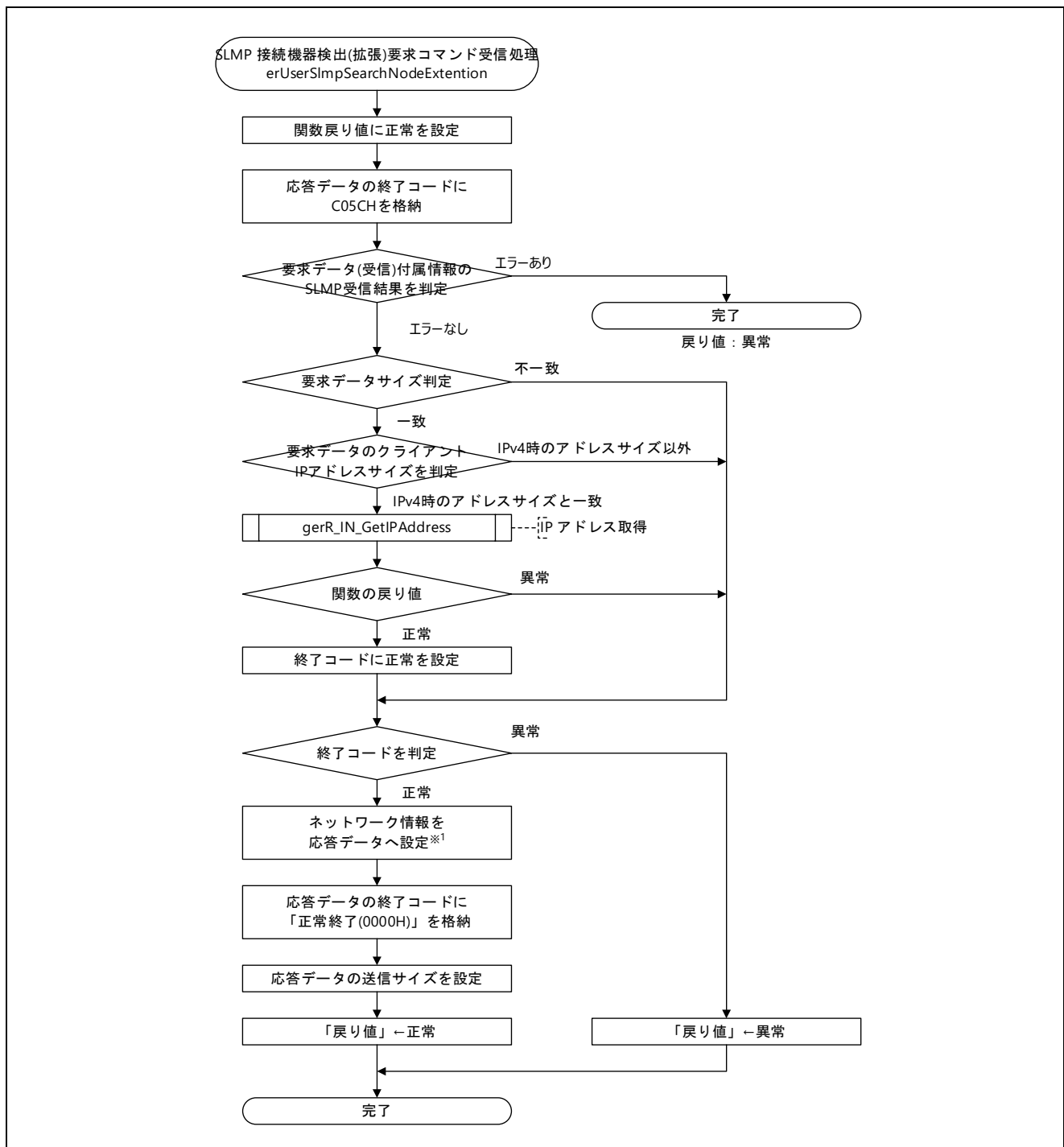
図 5.64 SLMP 接続機器検出(拡張)要求コマンド受信処理フロー図
