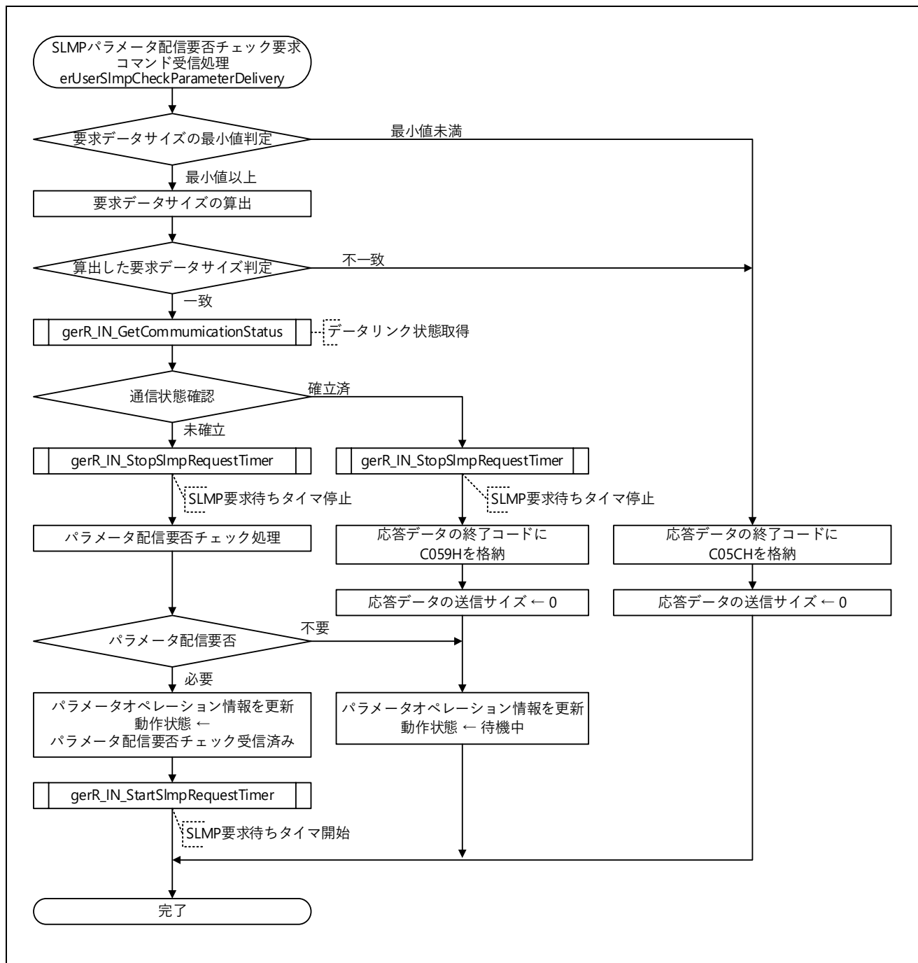
図 5.57 SLMP パラメータ配信可否チェック要求コマンド受信処理フロー図
