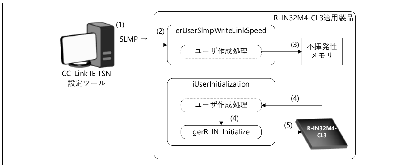
図 5.63 SLMP 経由の通信速度設定イメージ
