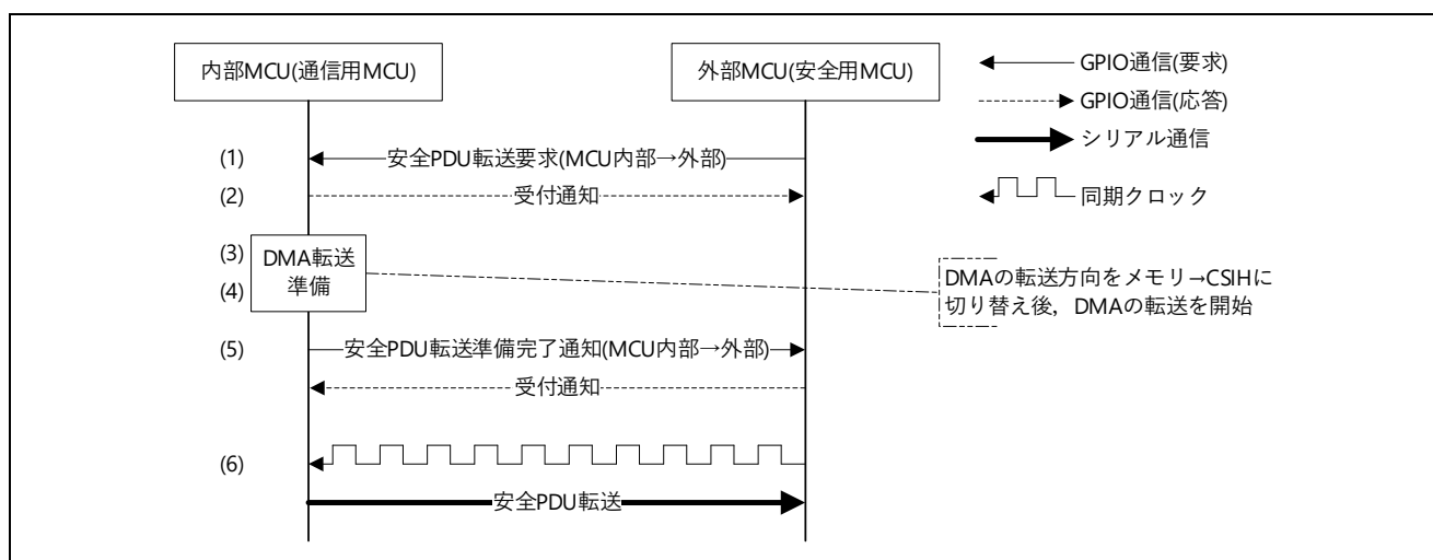
図 5.90 内部 MCU から外部 MCU へ安全 PDU を転送
