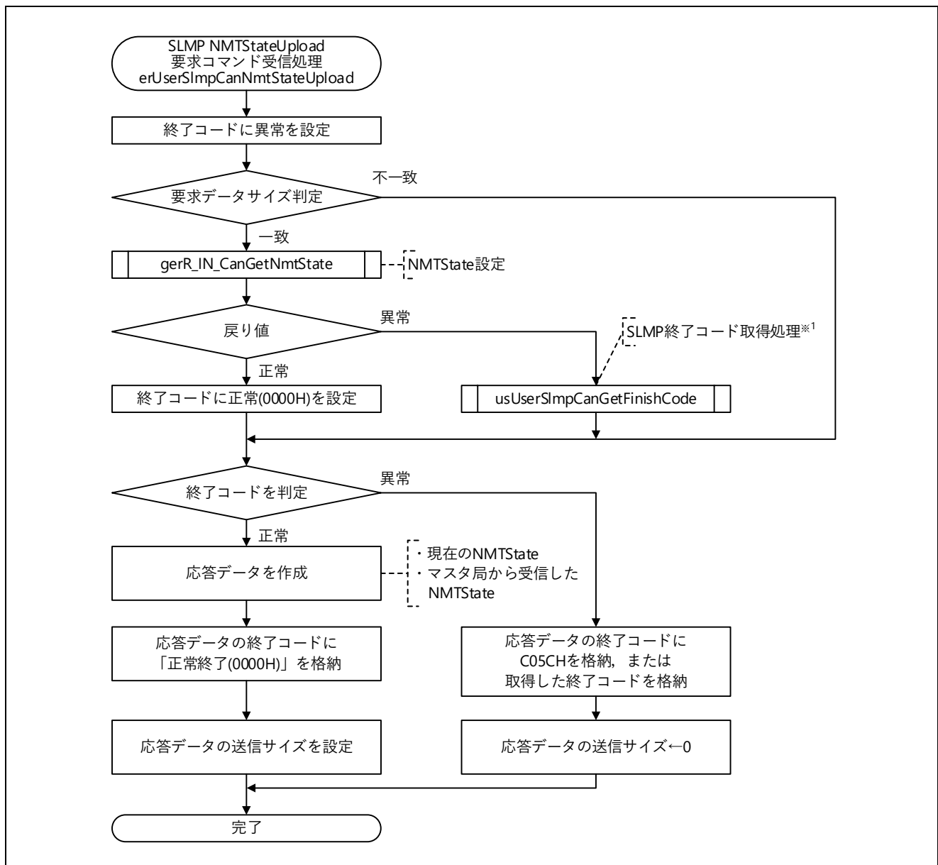
図 5.80 SLMP NMTStateUpload 要求コマンド受信処理フロー図
