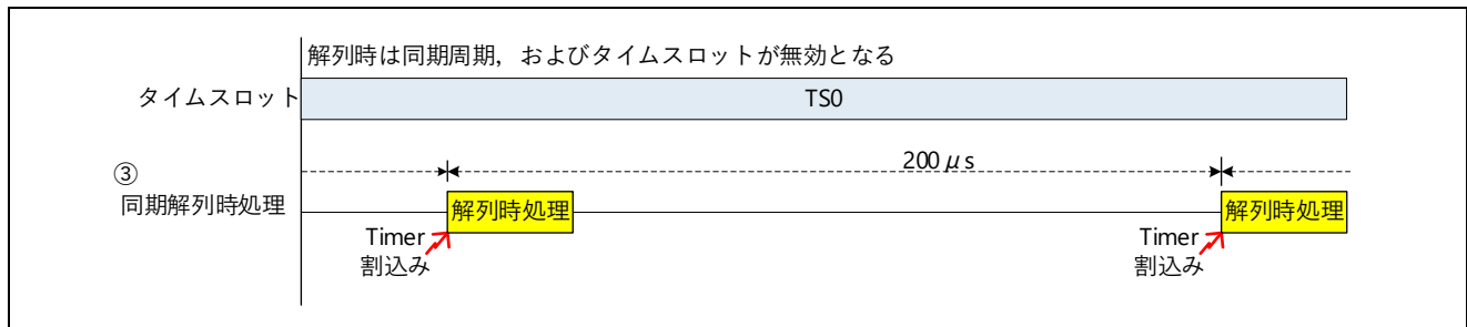
図 4.10 同期通信のタスク/処理タイミングチャート(データリンク未実施(解列状態))
