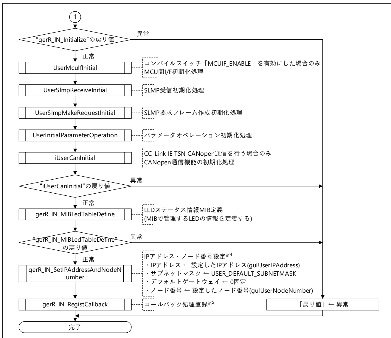
図 5.19 初期化処理フロー図
