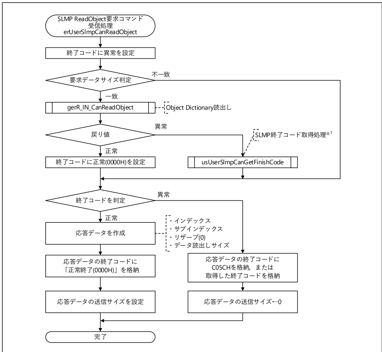
図 5.76 SLMP ReadObject 要求コマンド受信処理フロー図
