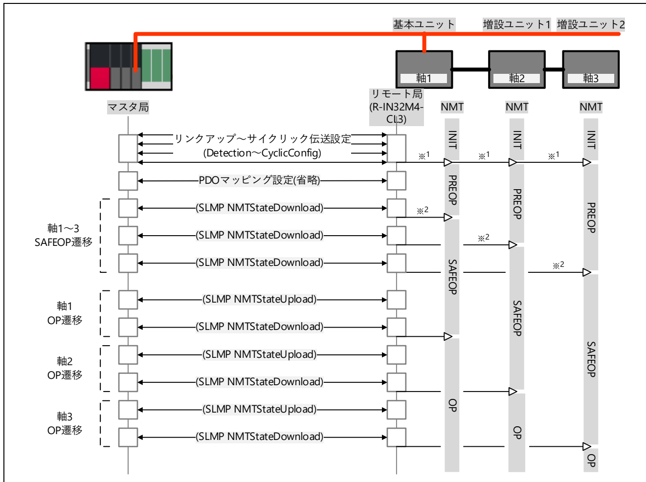
図 5.73 NMT の遷移イメージ(増設ユニット装着時)
