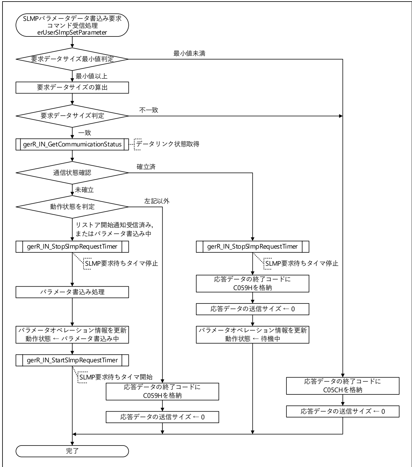
図 5.61 SLMP パラメータデータ書き込み要求コマンド受信処理フロー図
