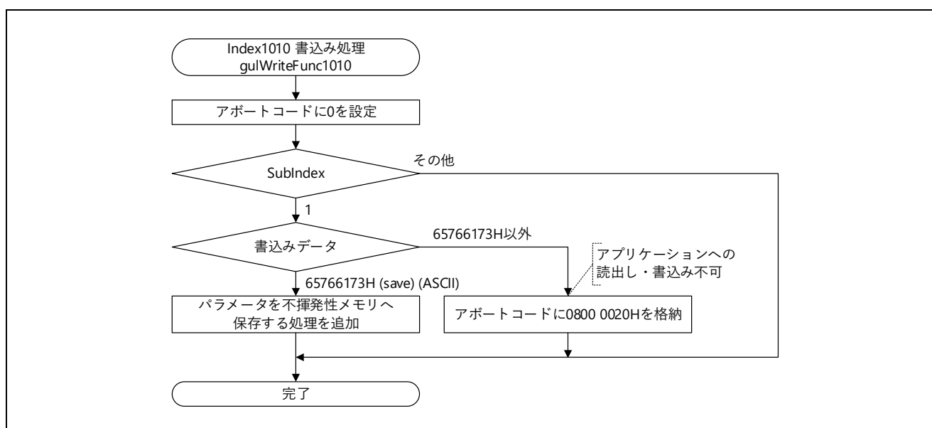
図 5.84 Index1010 書込み処理フロー図
