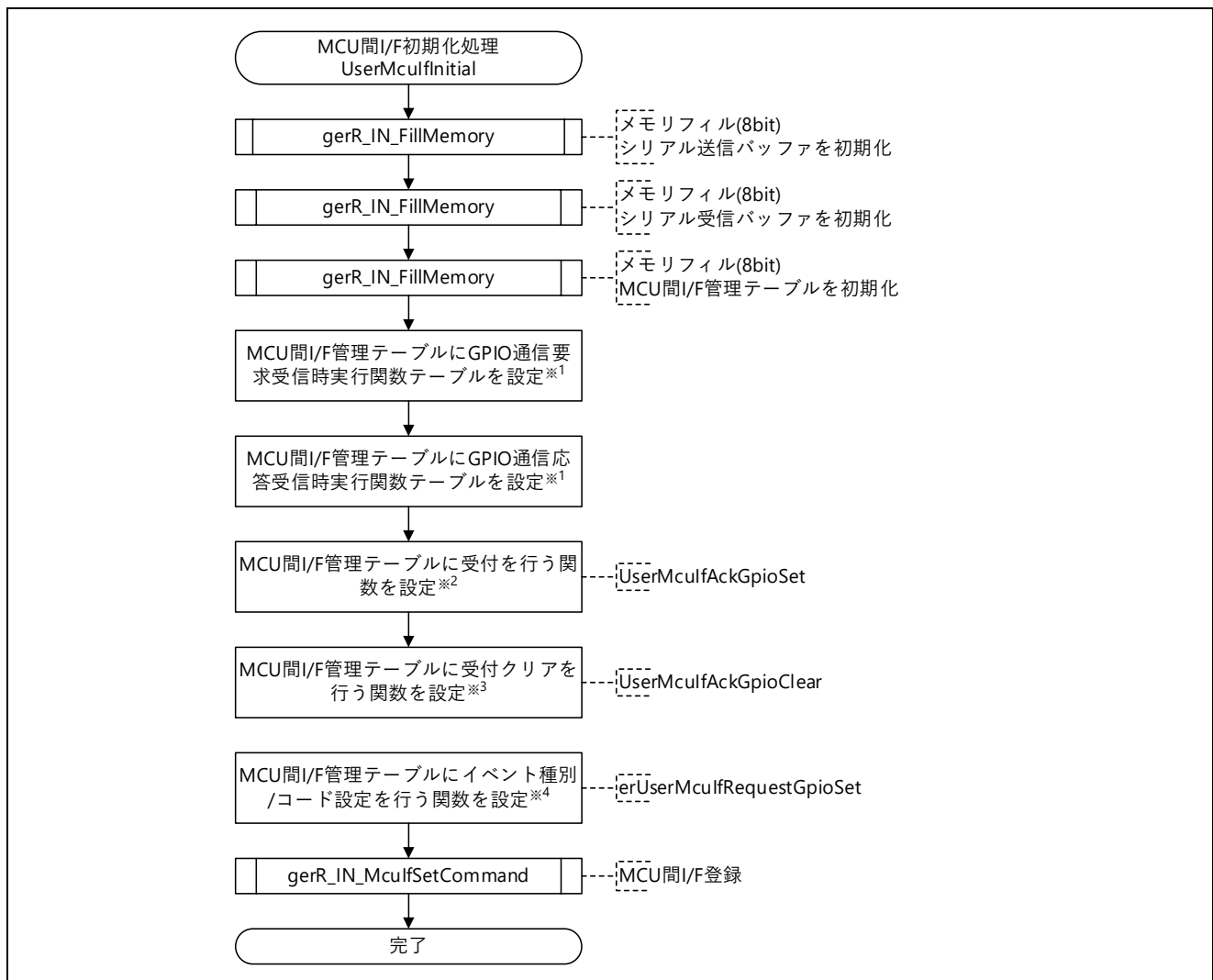
図 5.92 MCU 間 I/F 初期化処理フロー図
