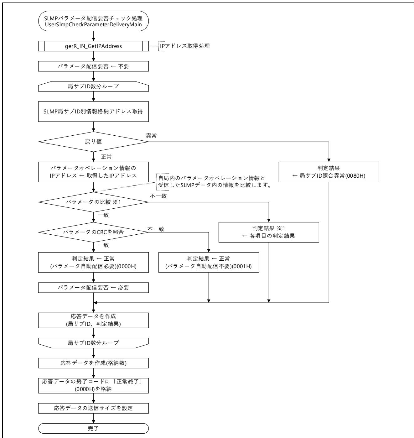
図 5.58 SLMP パラメータ配信要否チェック処理フロー図
