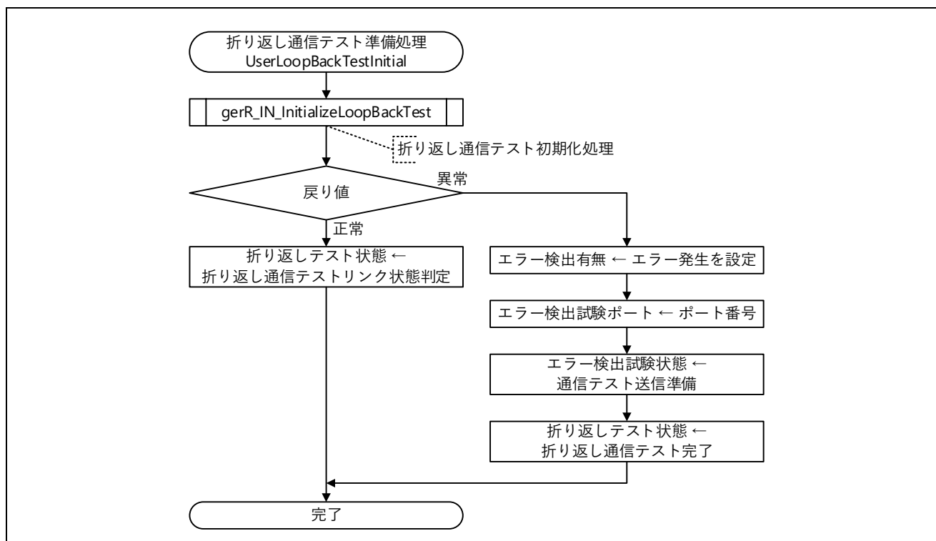
図 5.103 折り返し通信テスト準備処理フロー図
