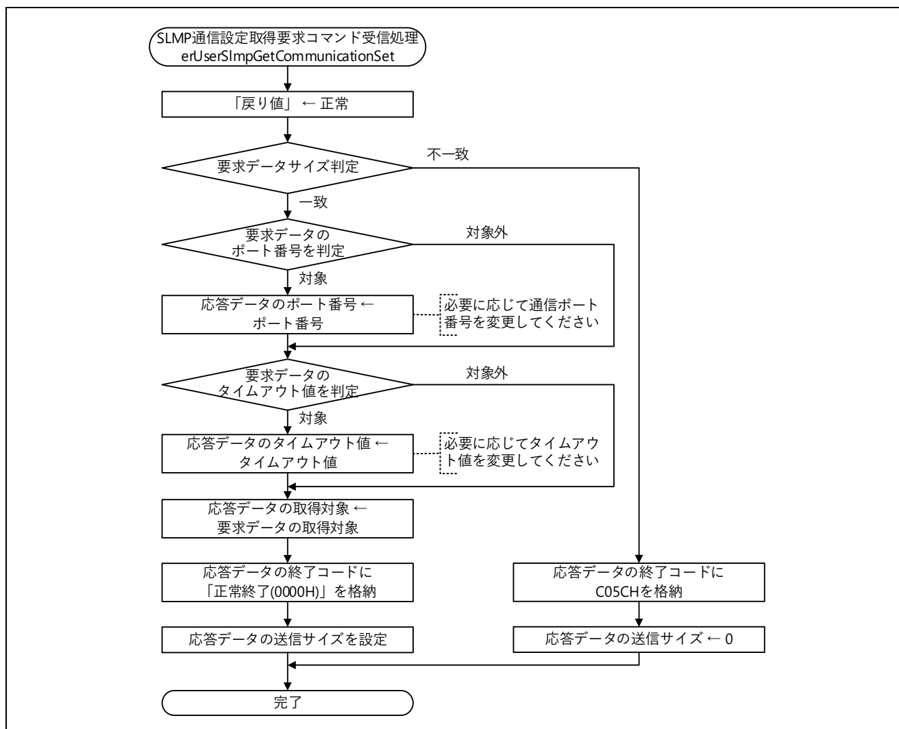
図 5.56 SLMP 通信設定取得要求コマンド受信処理フロー図
