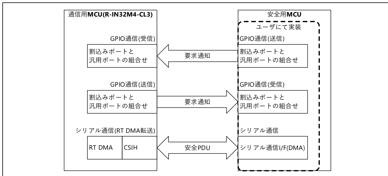
図 5.86 MCU 間 I/F のイメージ
