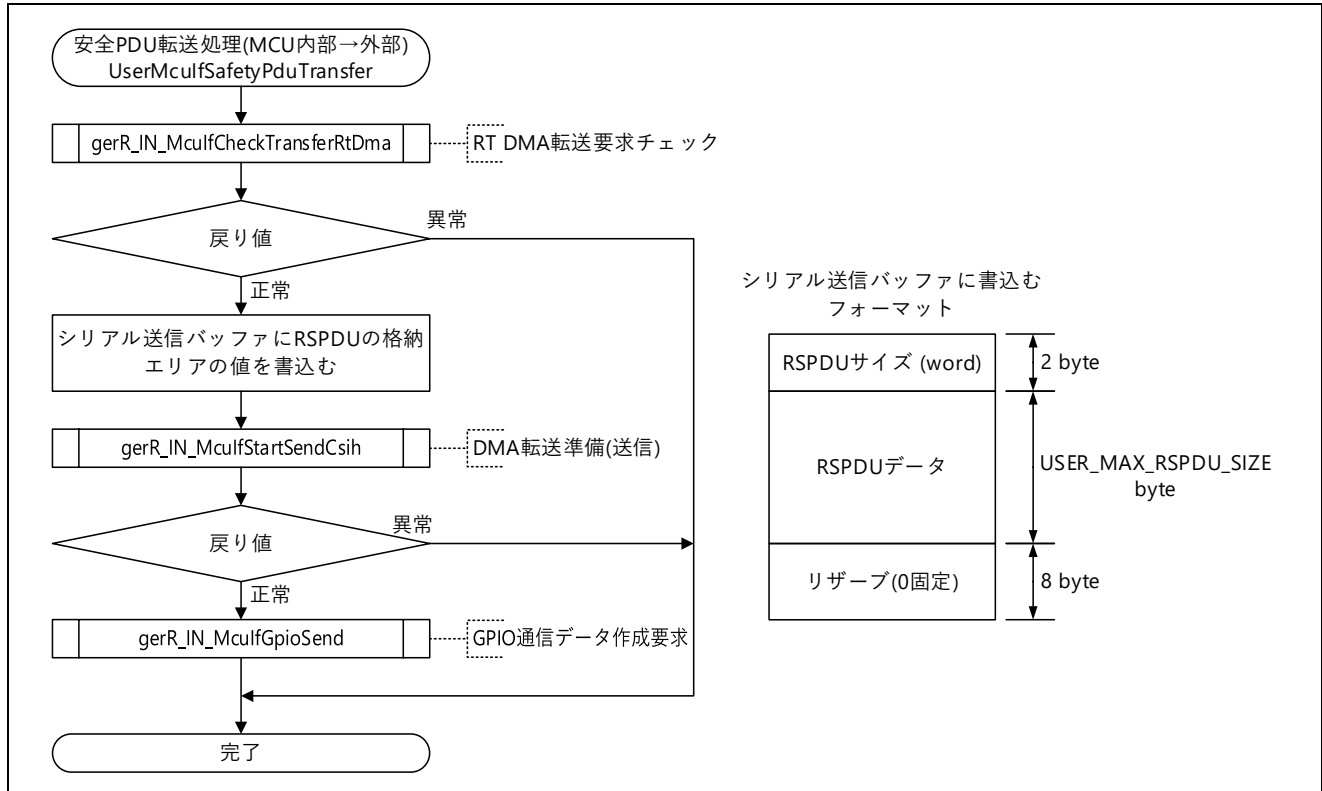
図 5.96 安全 PDU 転送処理(MCU 内部→外部)フロー図
