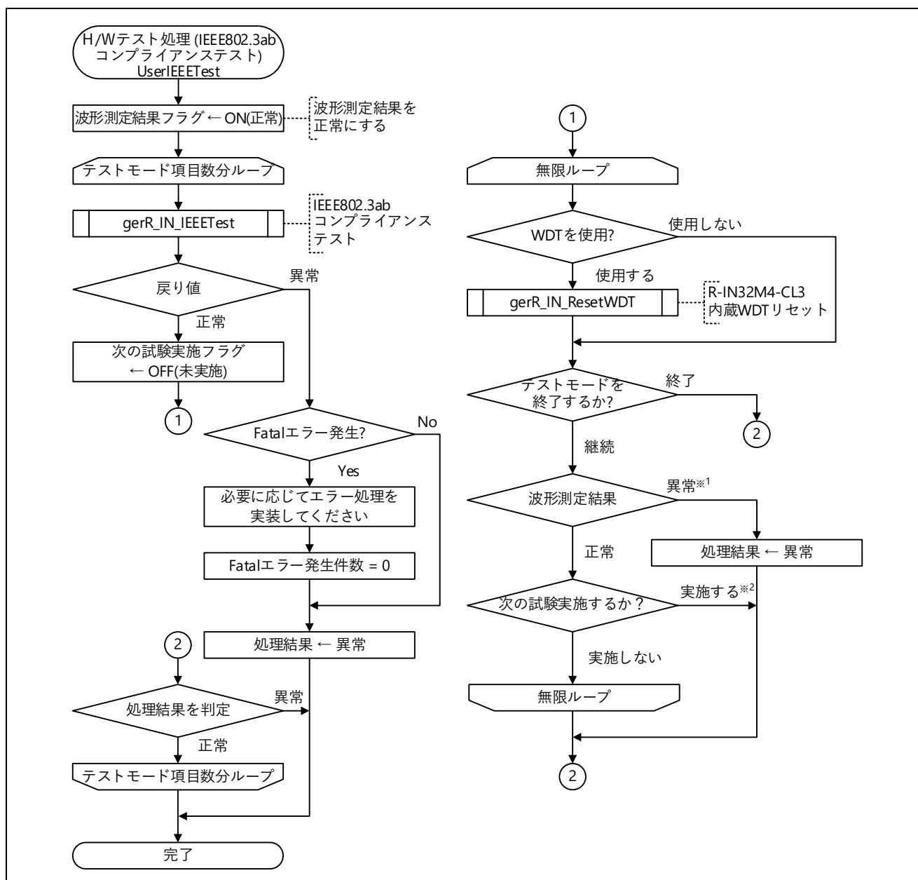
図 5.101 H/W テスト処理(IEEE802.3ab コンプライアンステスト)処理フロー図
