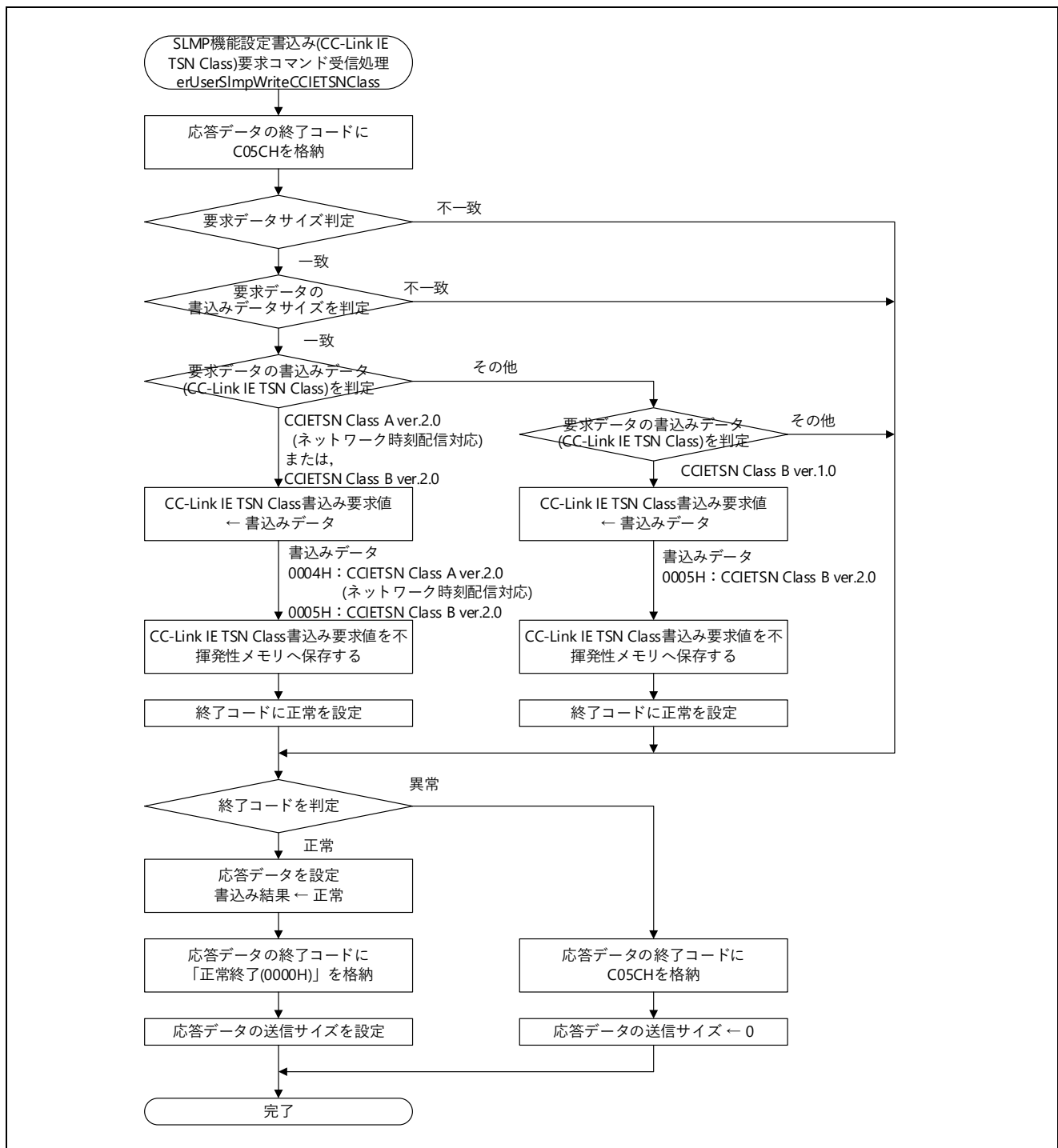
図 5.69 SLMP 機能設定書込み(CC-Link IE TSN Class)要求コマンド受信処理フロー図
