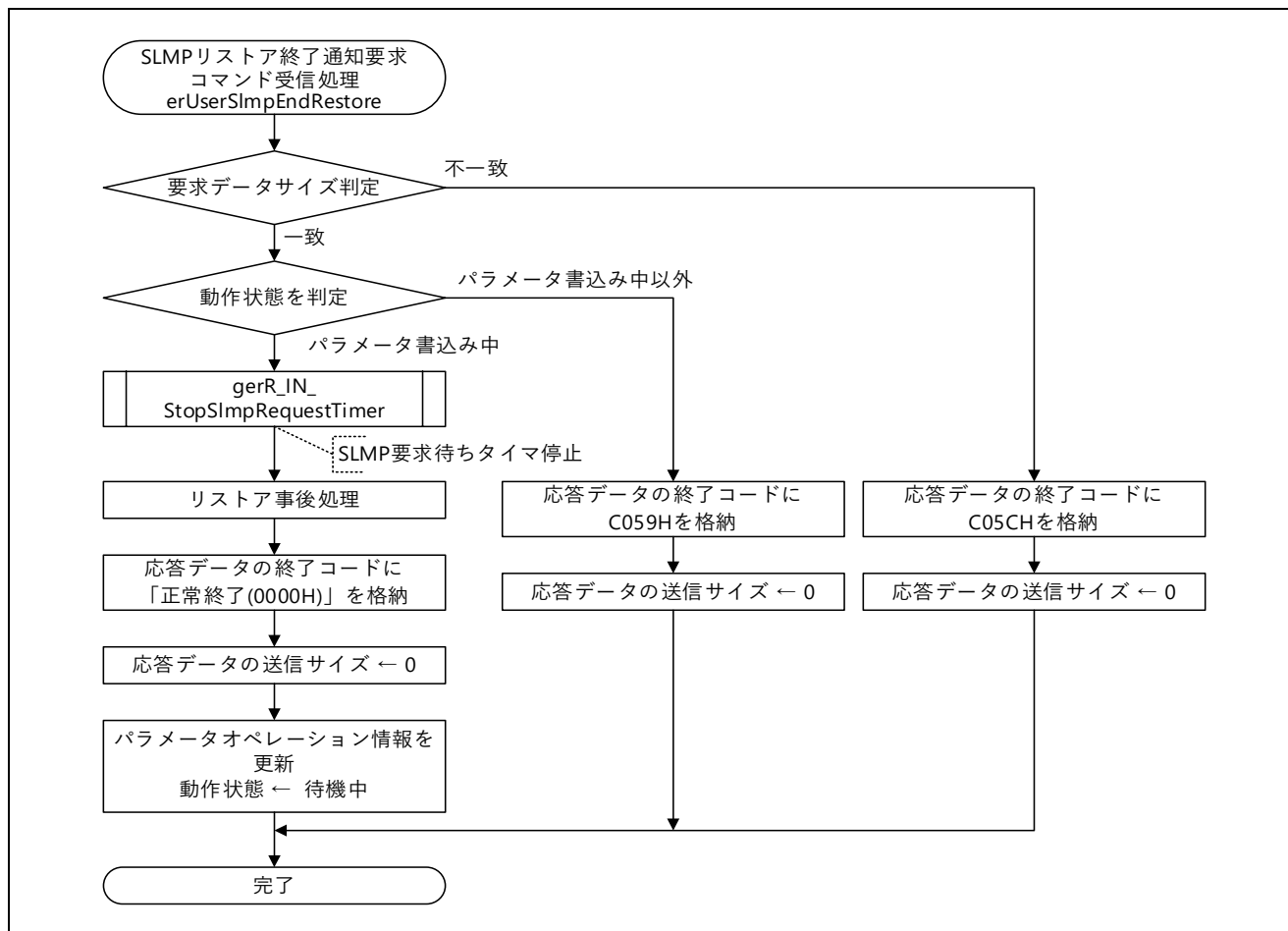
図 5.60 SLMP リストア終了通知要求コマンド受信処理フロー図
