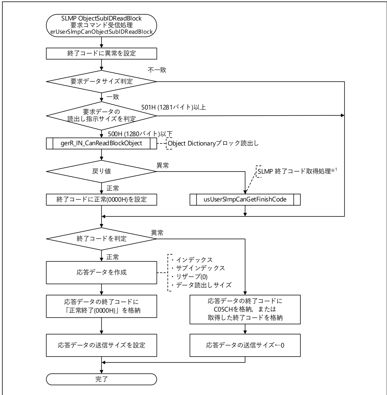
図 5.78 SLMP ObjectSubIDReadBlock 要求コマンド受信処理フロー図
