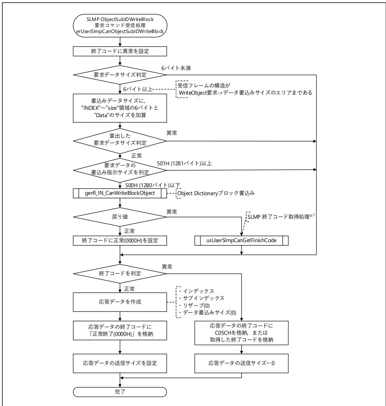
図 5.79 SLMP ObjectSubIDWriteBlock 要求コマンド受信処理フロー図
