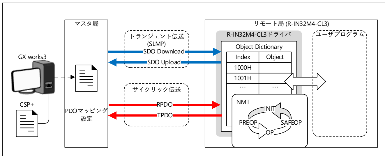
図 4.11 CC-Link IE TSN における CANopen 通信のイメージ
