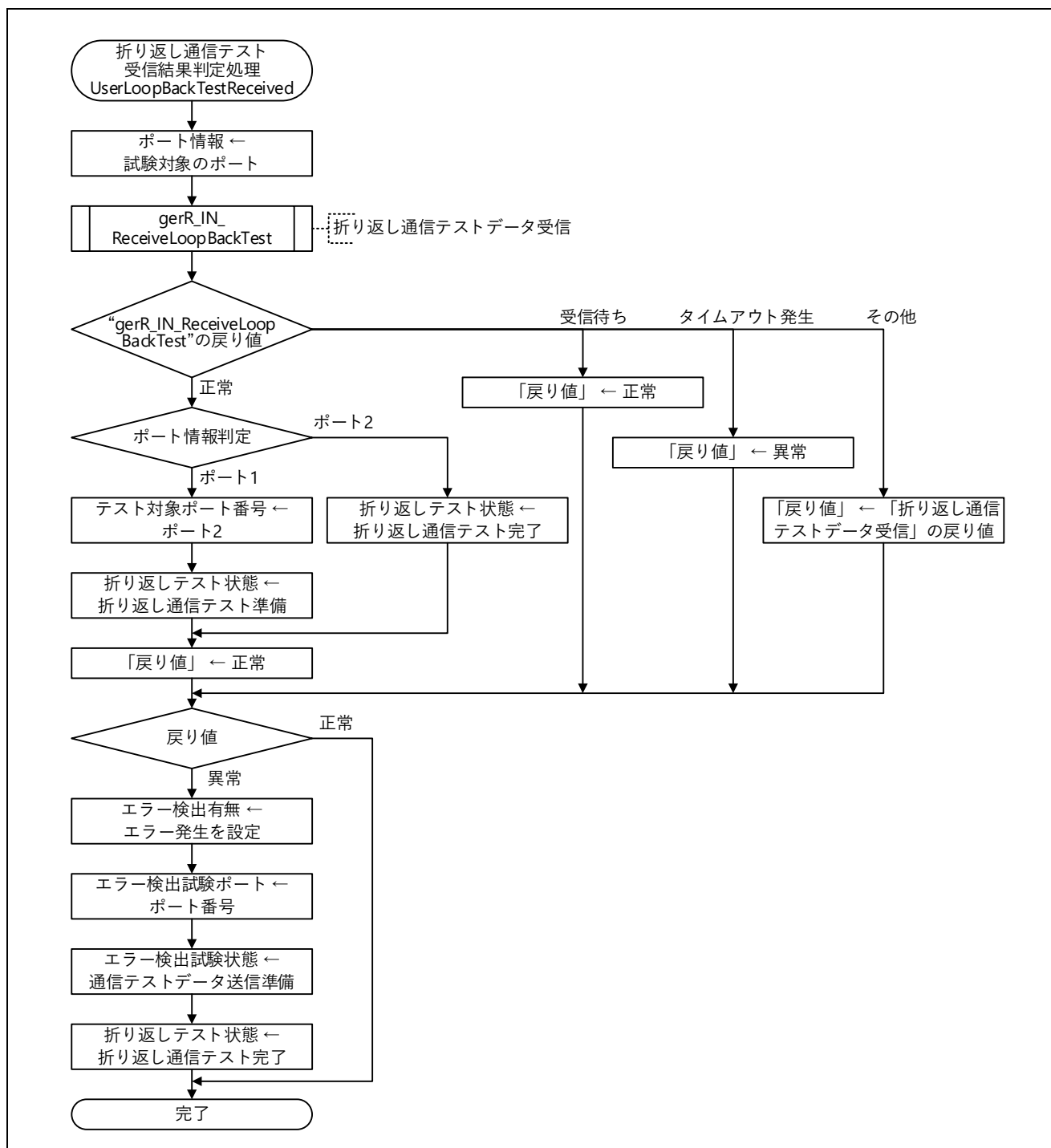
図 5.106 折り返し通信テスト受信結果判定処理フロー図
