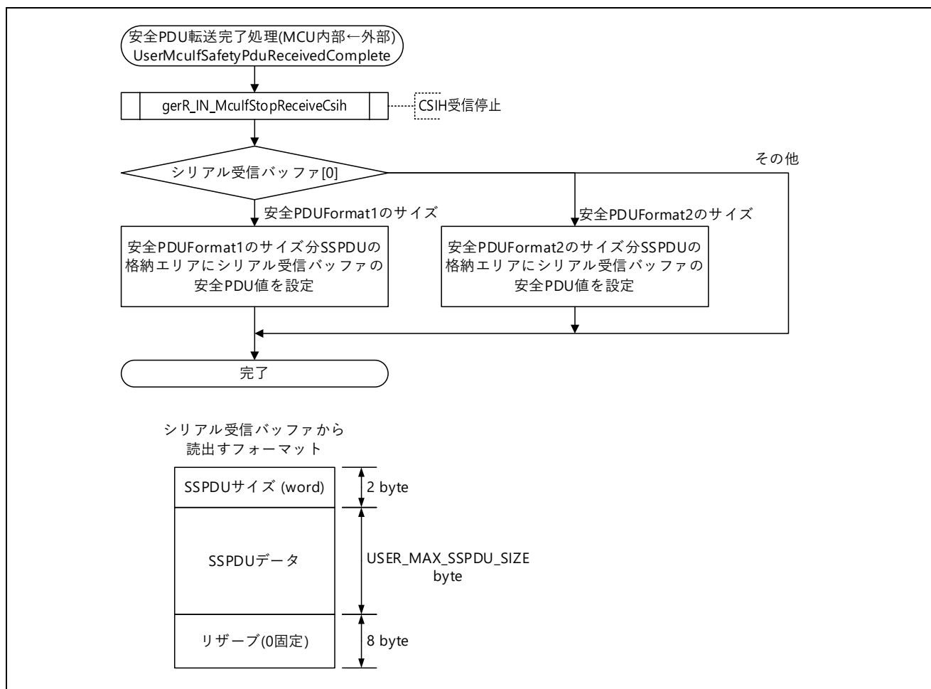
図 5.100 安全 PDU 転送完了処理(MCU 内部←外部)フロー図
