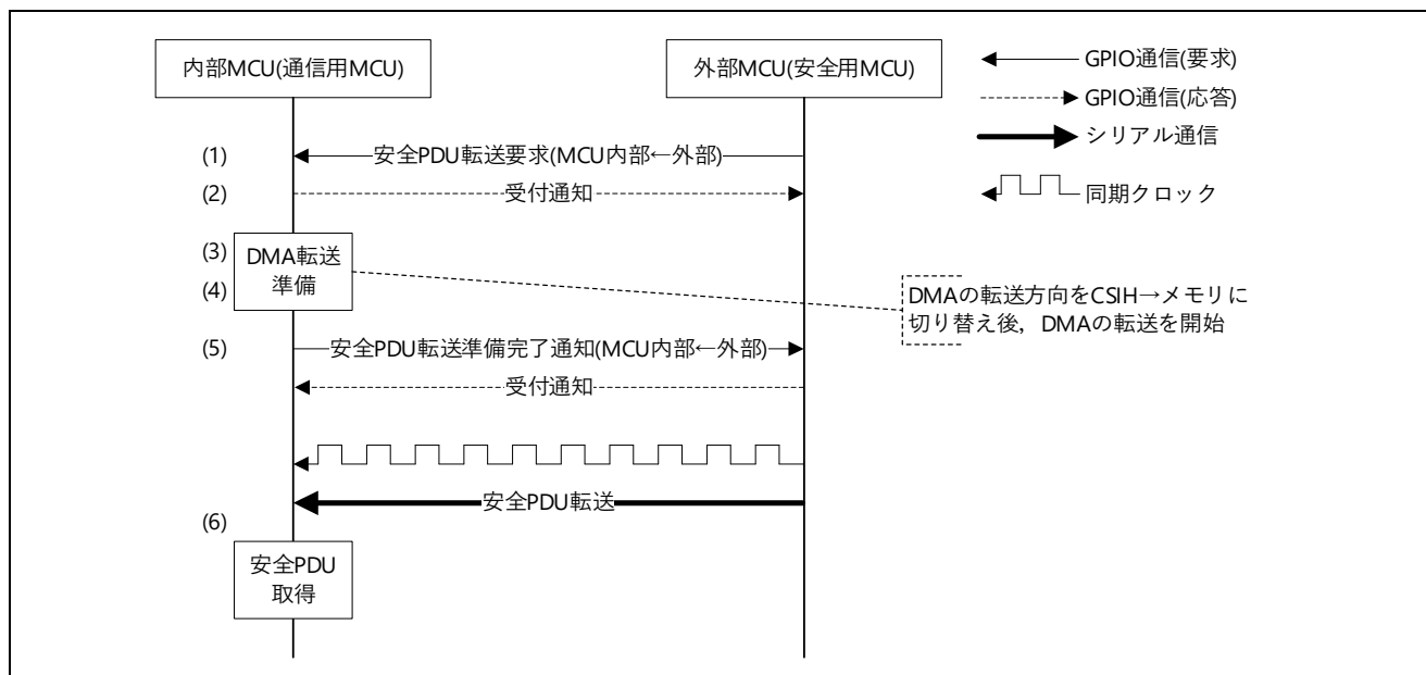
図 5.91 外部 MCU から内部 MCU へ安全 PDU を転送
