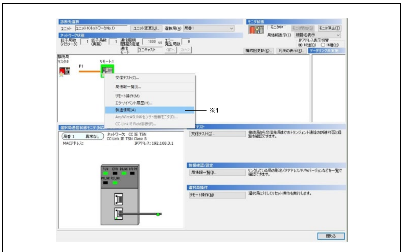
図 4.7 診断画面 (GX works3 の場合)
