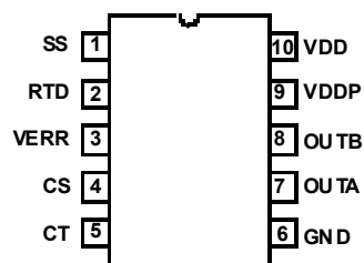
ISL6745 (MSOP)
