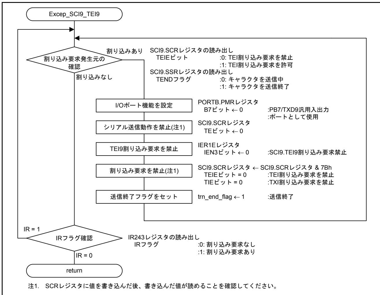
図 5.13 SCI9 送信終了割り込み処理
