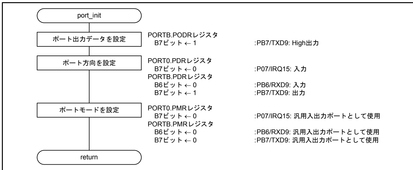
図 5.4 ポート初期設定
