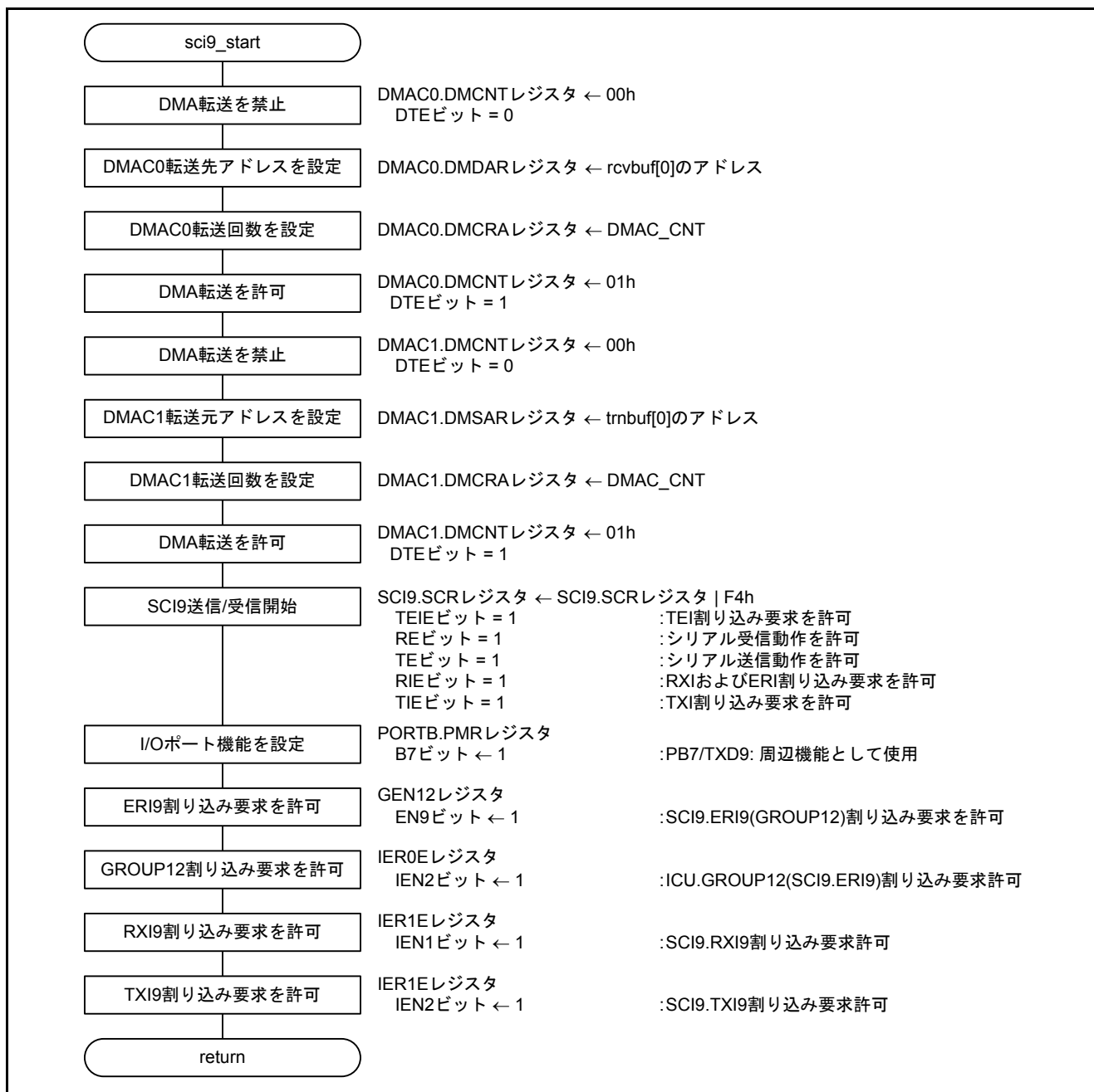
図 5.10 SCI9 送受信開始
