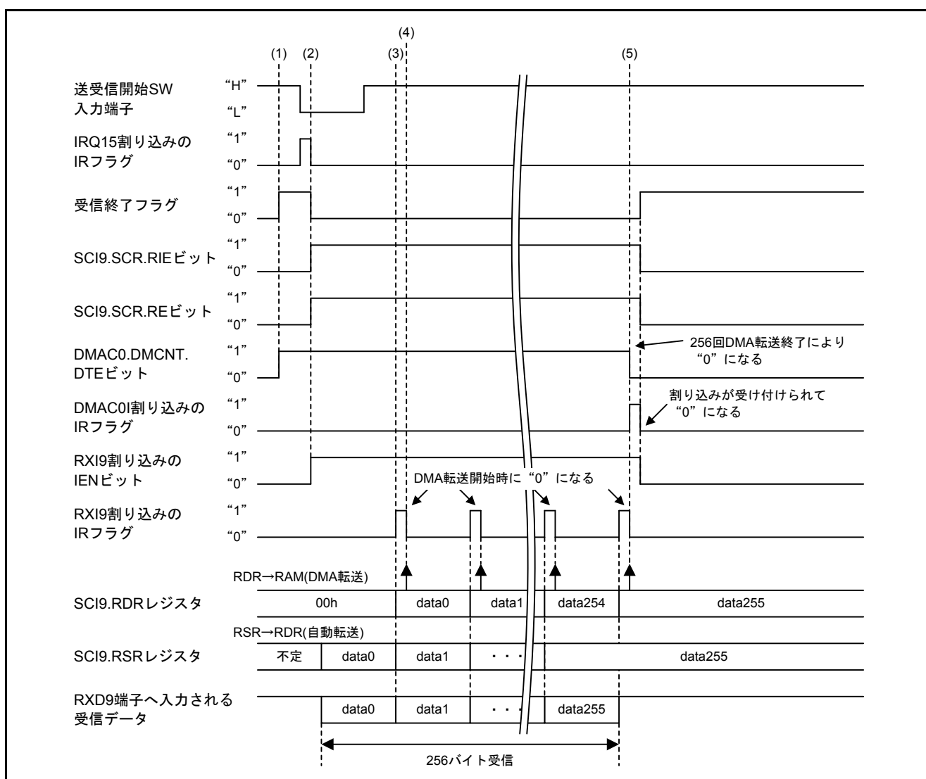
図 5.2 受信動作のタイミング図
