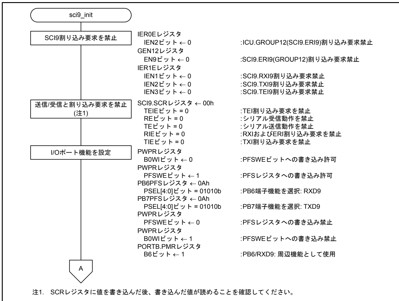
図 5.6 SCI9 初期設定(1/2)
