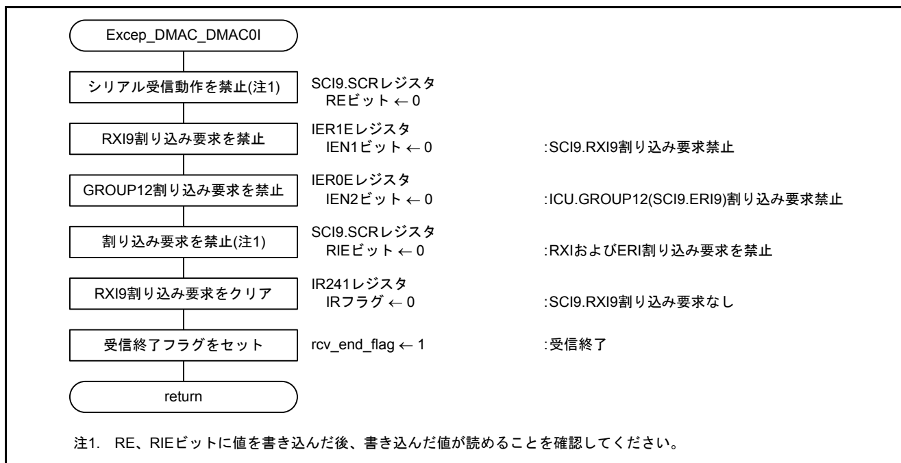
図 5.11 DMAC0 転送終了割り込み処理
