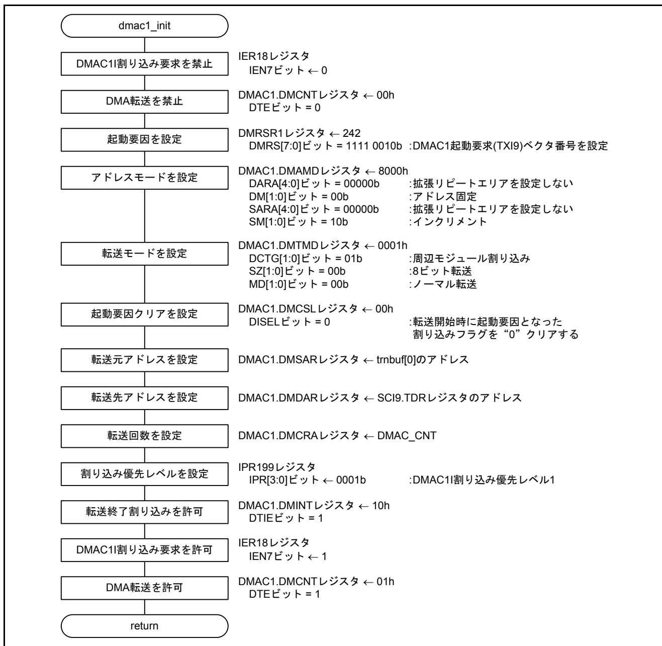
図 5.9 DMAC1 初期設定
