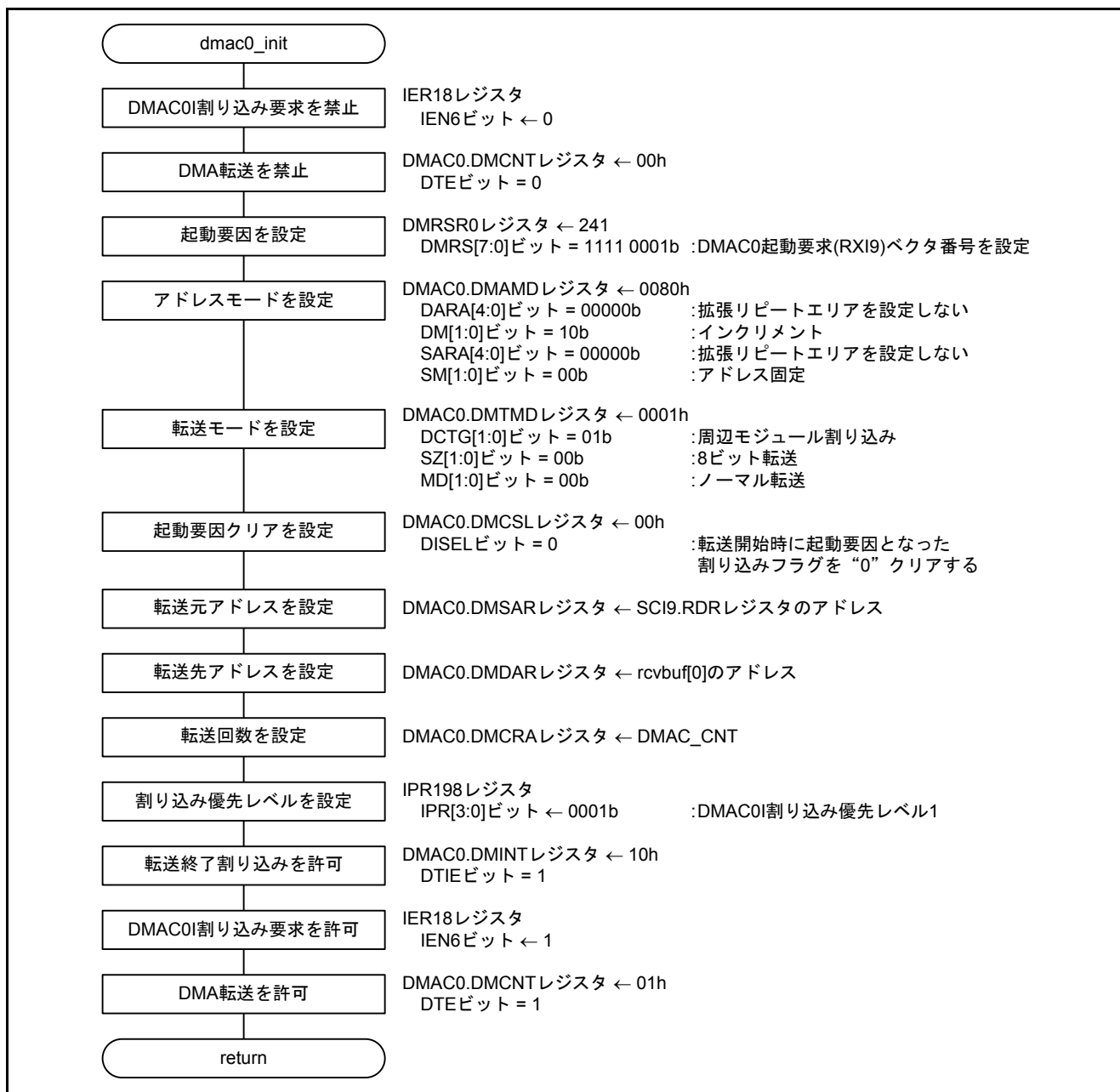
図 5.8 DMAC0 初期設定
