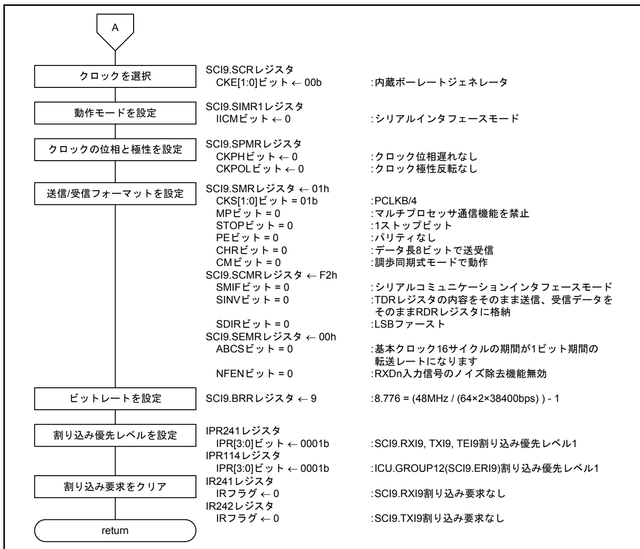
図 5.7 SCI9 初期設定(2/2)
