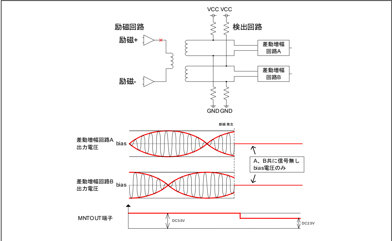
図 10.6 励磁側断線
