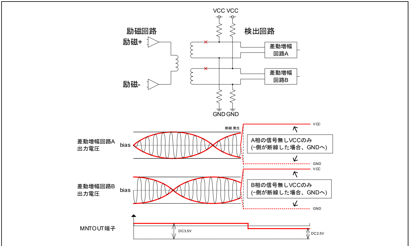
図 10.8 SIN+、COS+側断線
