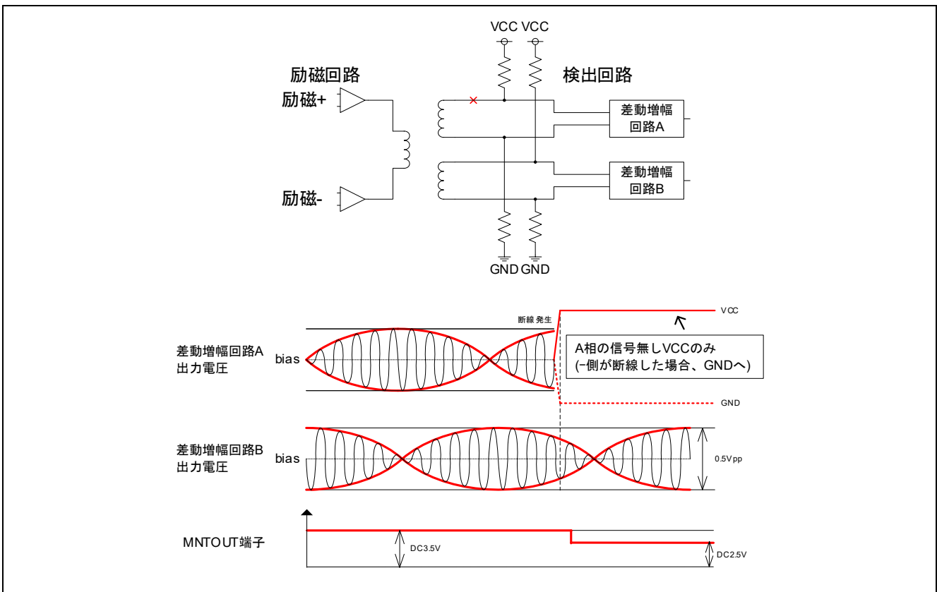
図 10.7 SIN+側断線
