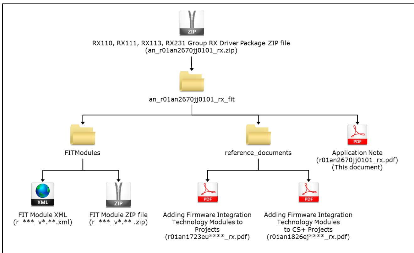
図 3-1 RX110、RX111、RX113、RX231 グループ用 RX Driver Package フォルダ構成
