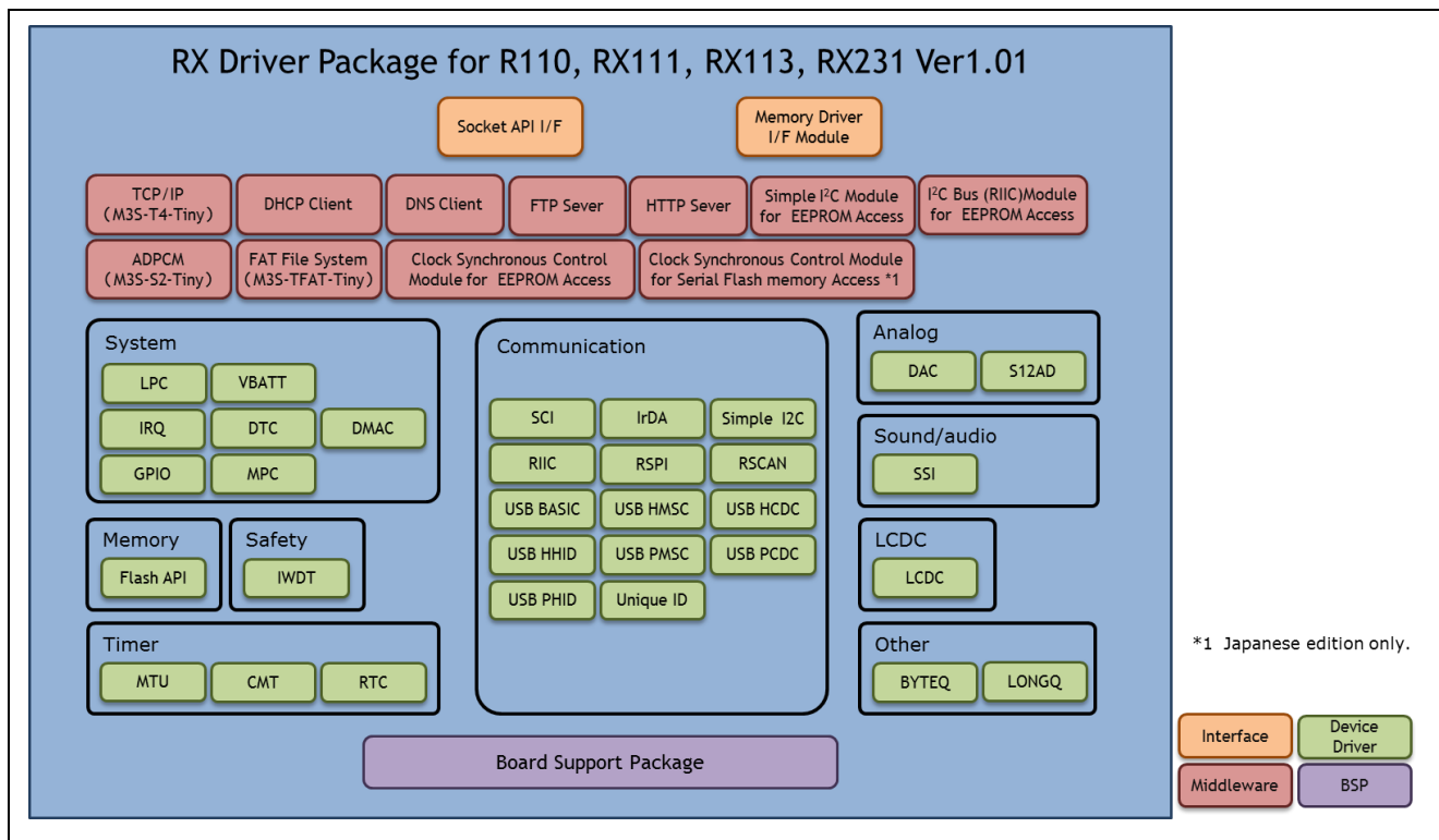
図 3-2 RX110、RX111、RX113、RX231 グループ用 RX Driver Package FIT モジュール構成イメージ
