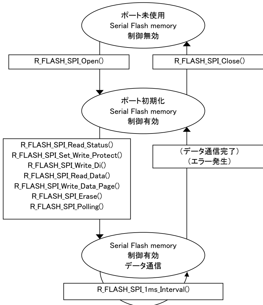
図 1-11 状態遷移図
