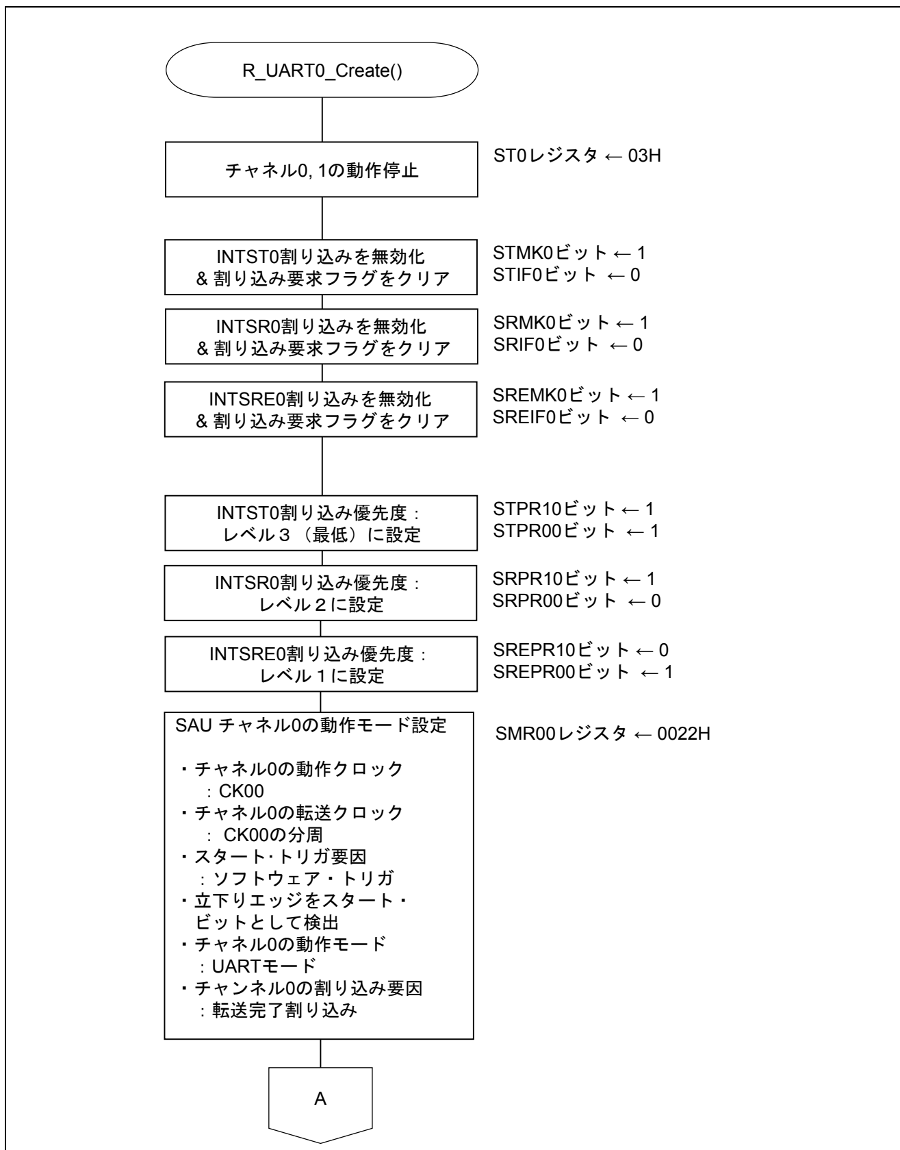
図 5.7 UART0 の設定 (1/3)
