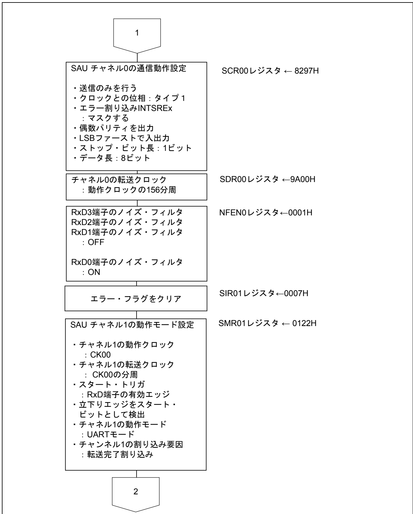
図 5.8 UART0 の設定 (2/3)
