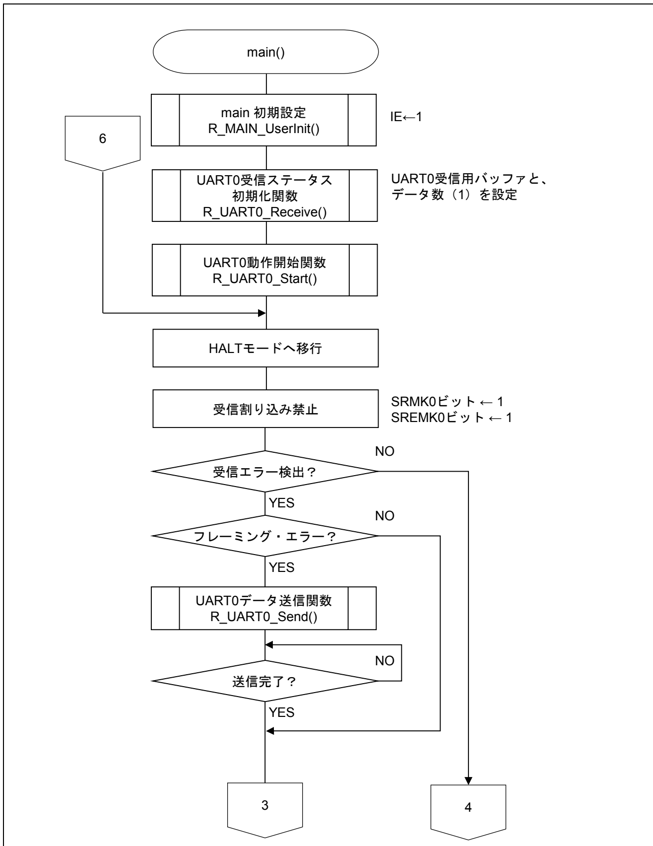
図 5.10 メイン関数 (1/3)
