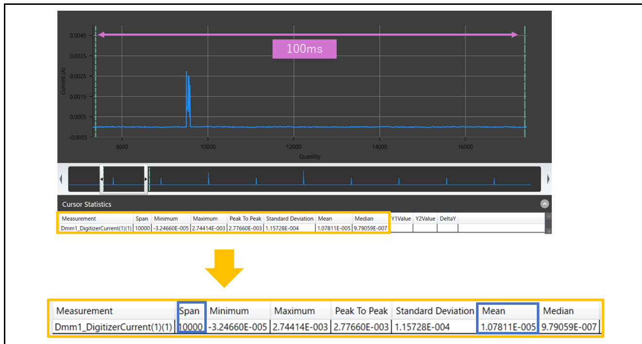
図 10-3 消費電流結果(SMS を使用したタッチ計測)
