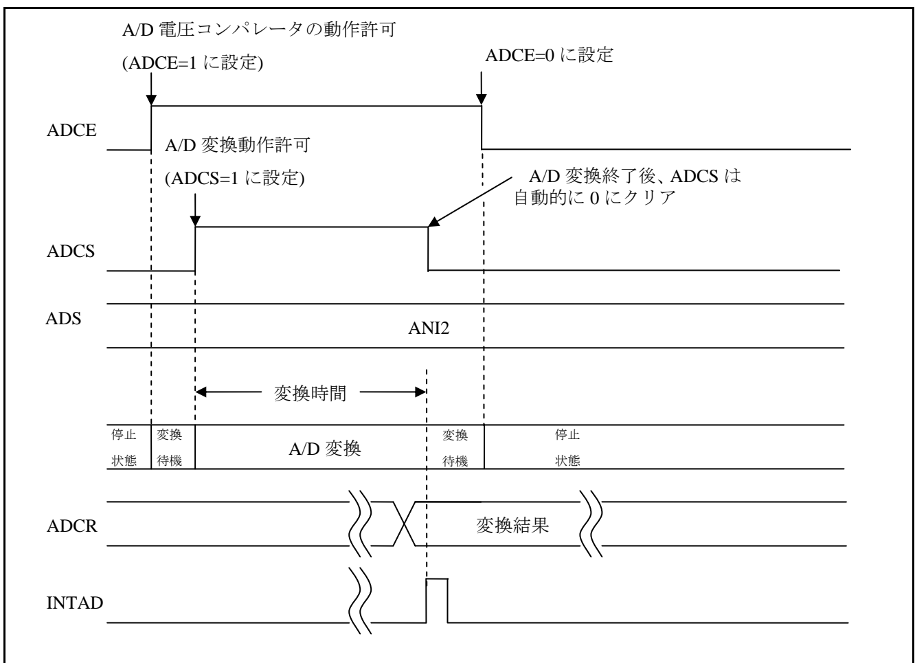
図1.1 A/D コンバータの変換概要
