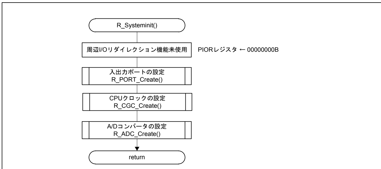
図 5.3 システム関数
