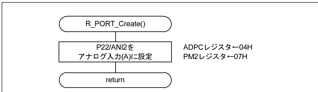
図 5.4 入出力ポートの設定
