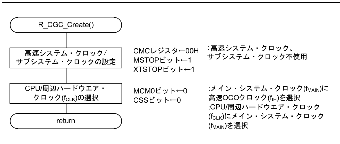
図 5.5 CPU クロックの設定
