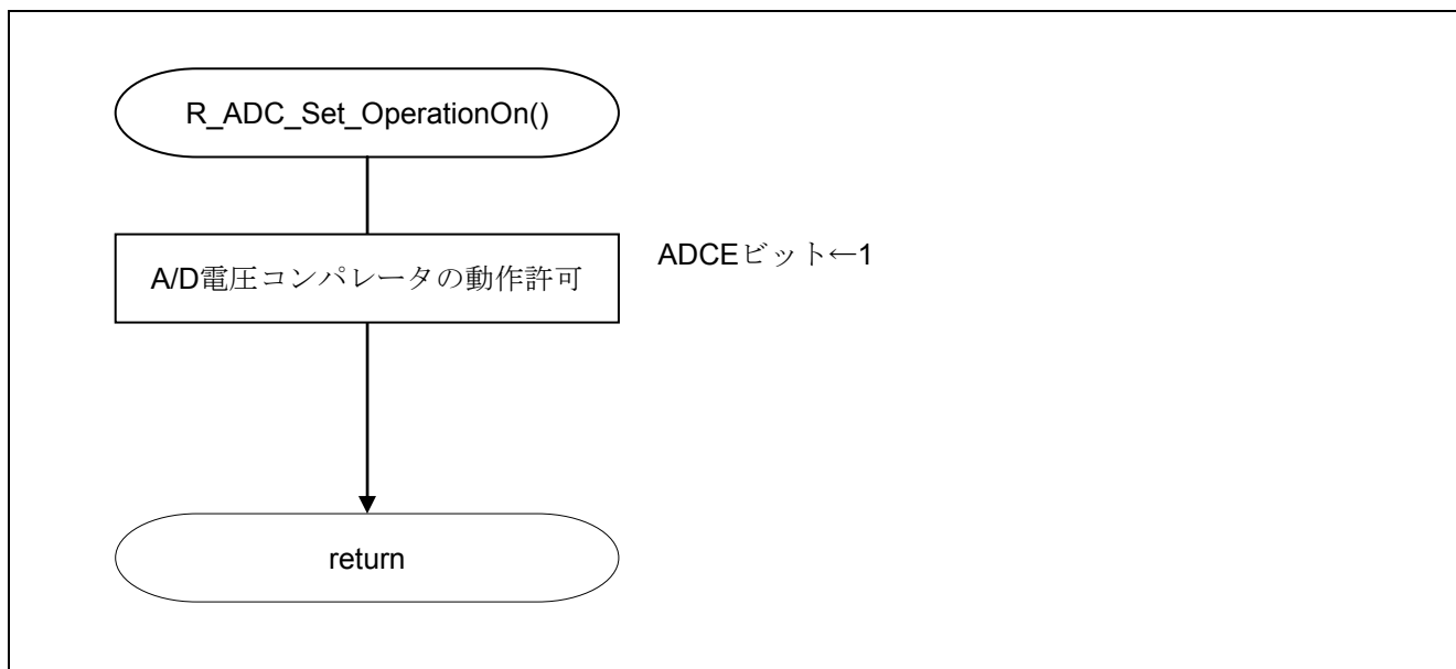
図 5.8 A/D 電圧コンパレータ動作許可
