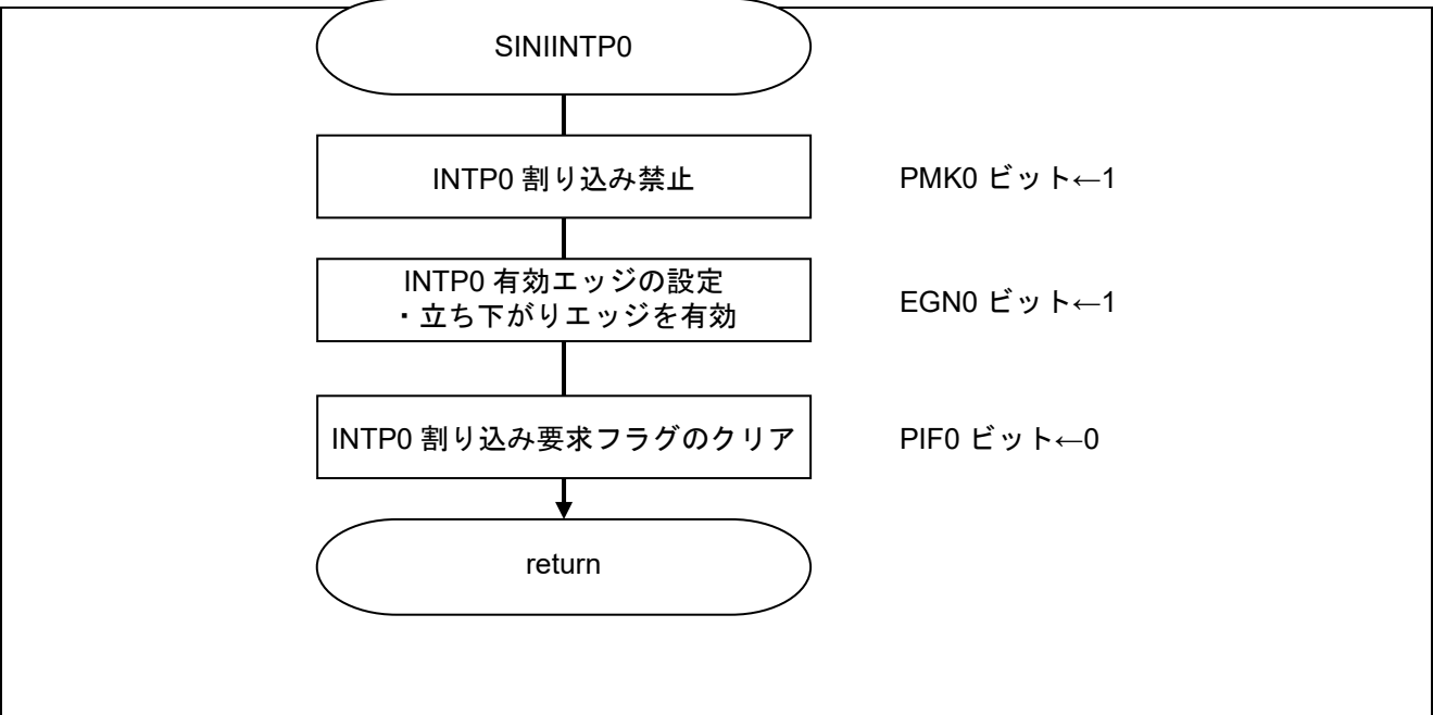
図 5.6 INTC モジュールの設定
