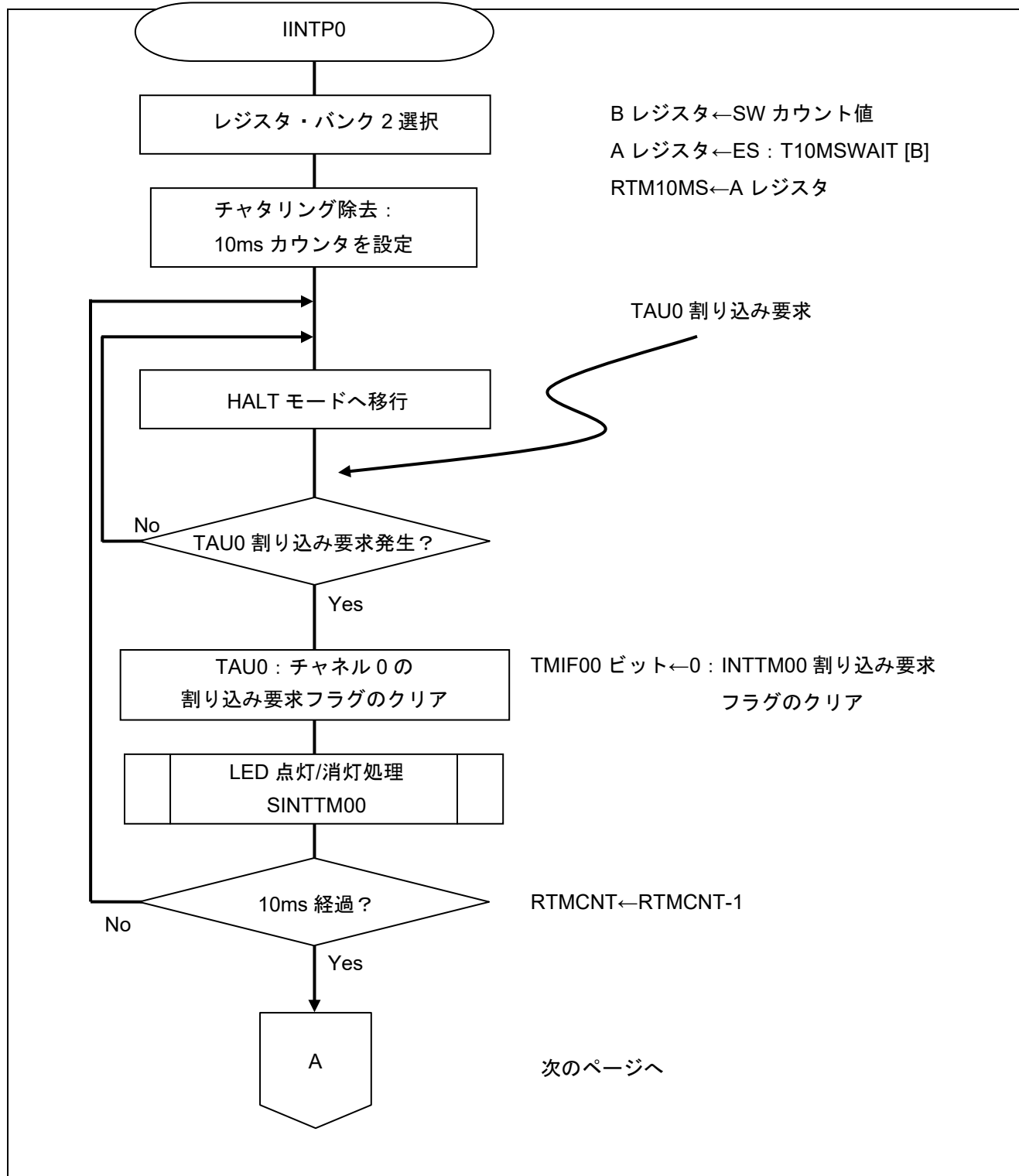
図 5.11 INTP0 割り込み処理 (1/2)
