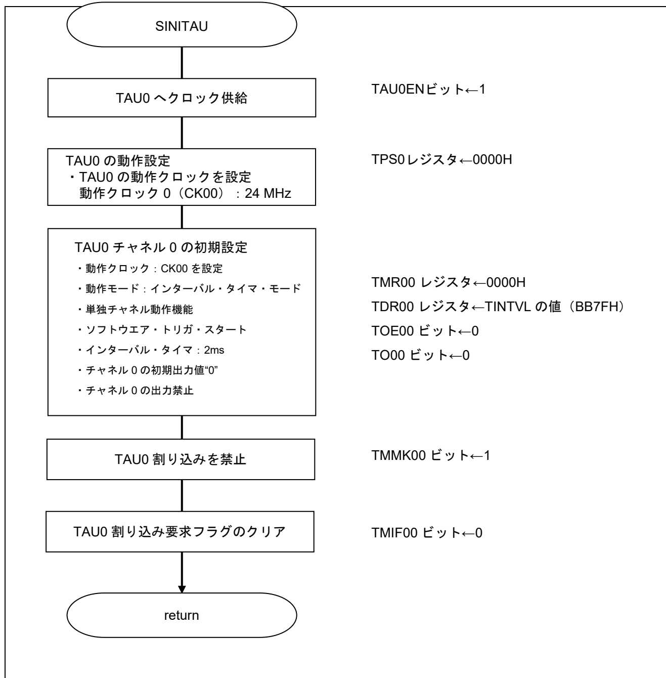
図 5.5 タイマ・アレイ・ユニットの設定
