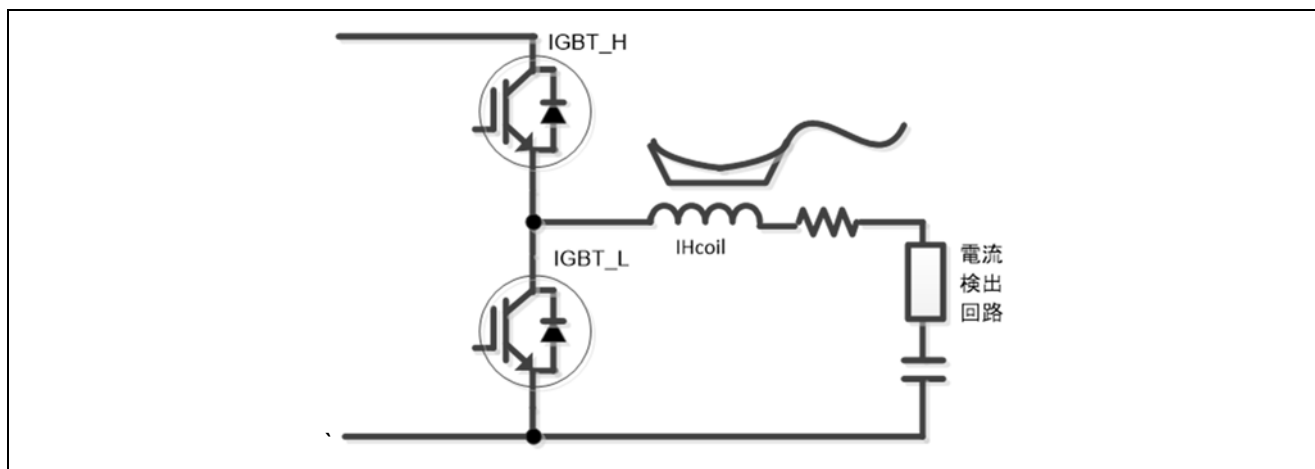
図 1.1 LC 共振型ハーフブリッジ等価回路
