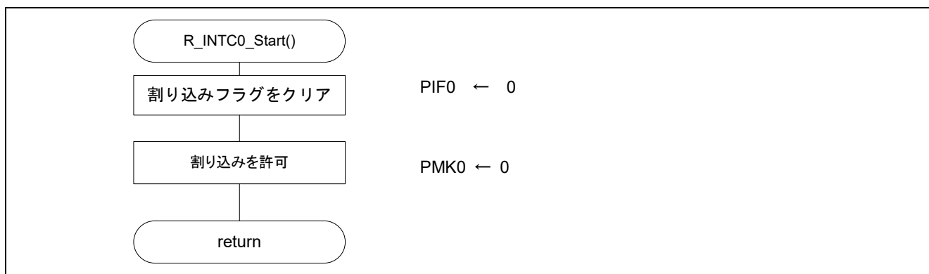
図 4.10 割り込み許可設定
