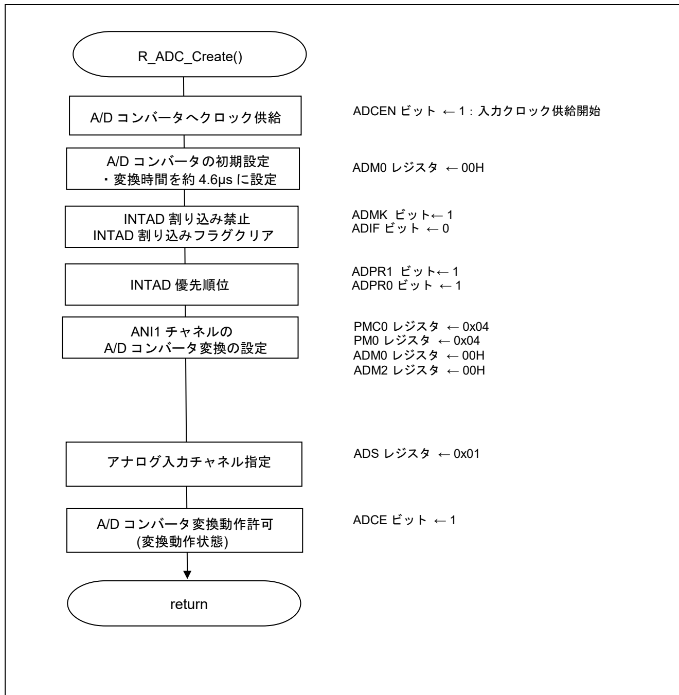
図 4.6 A/D コンバータの設定
