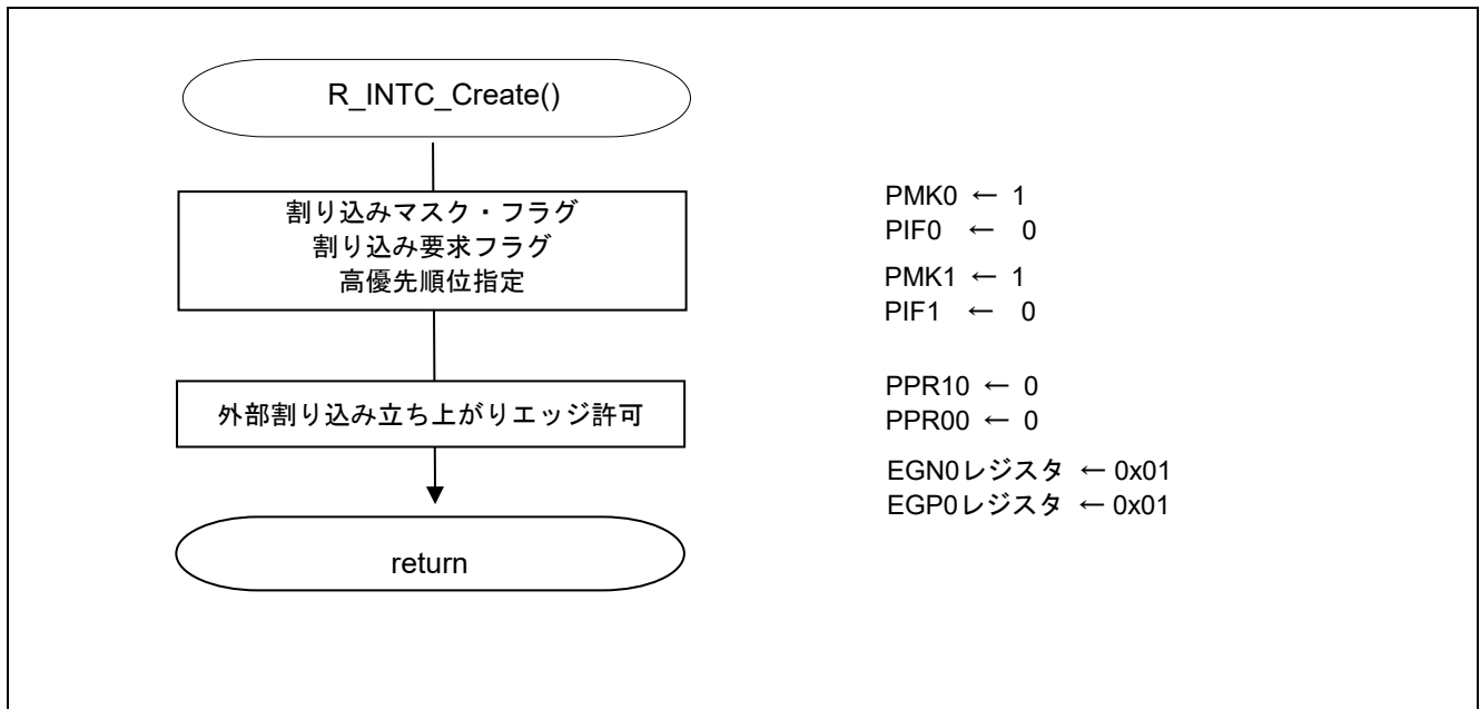
図 4.7 外部割り込みの設定
