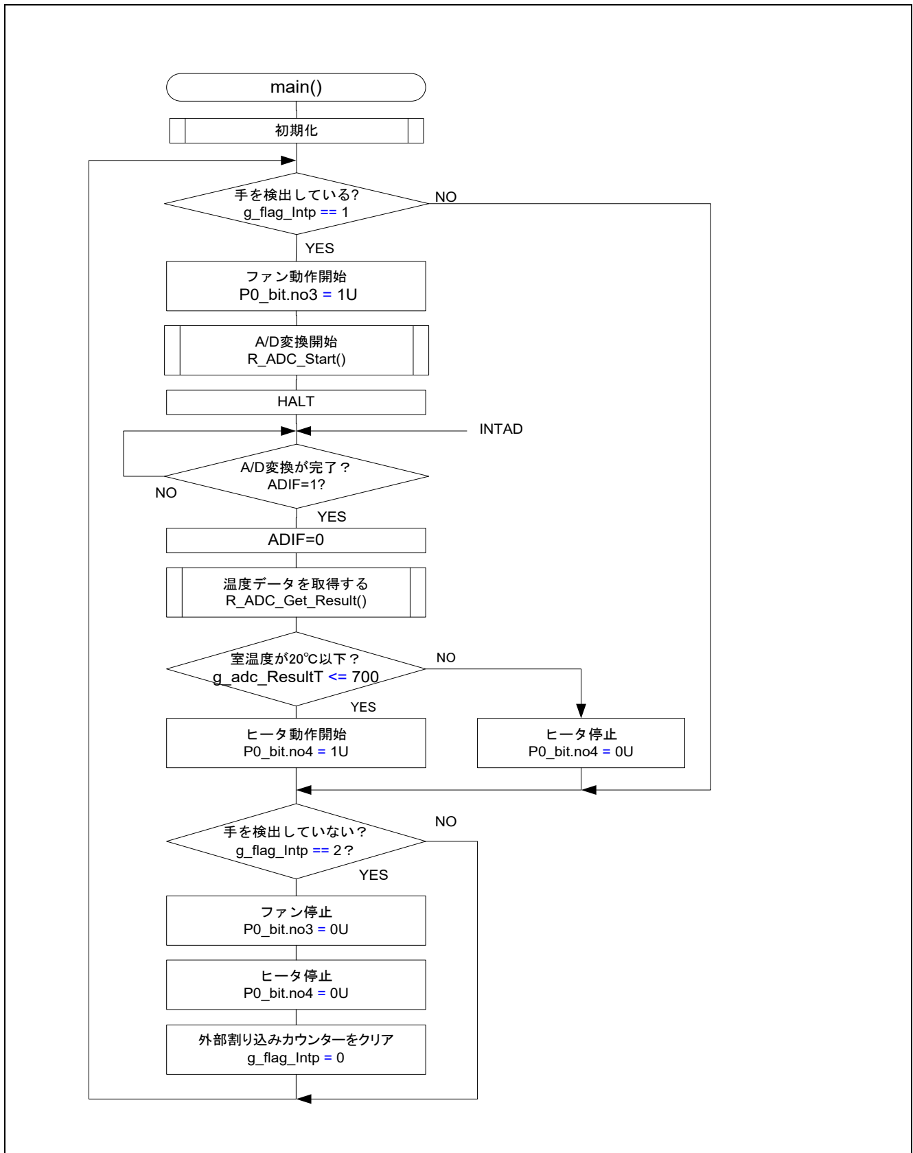
図 4.8 メイン処理のフローチャート
