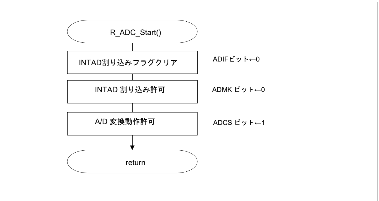
図 4.11 A/D コンバータ動作開始設定
