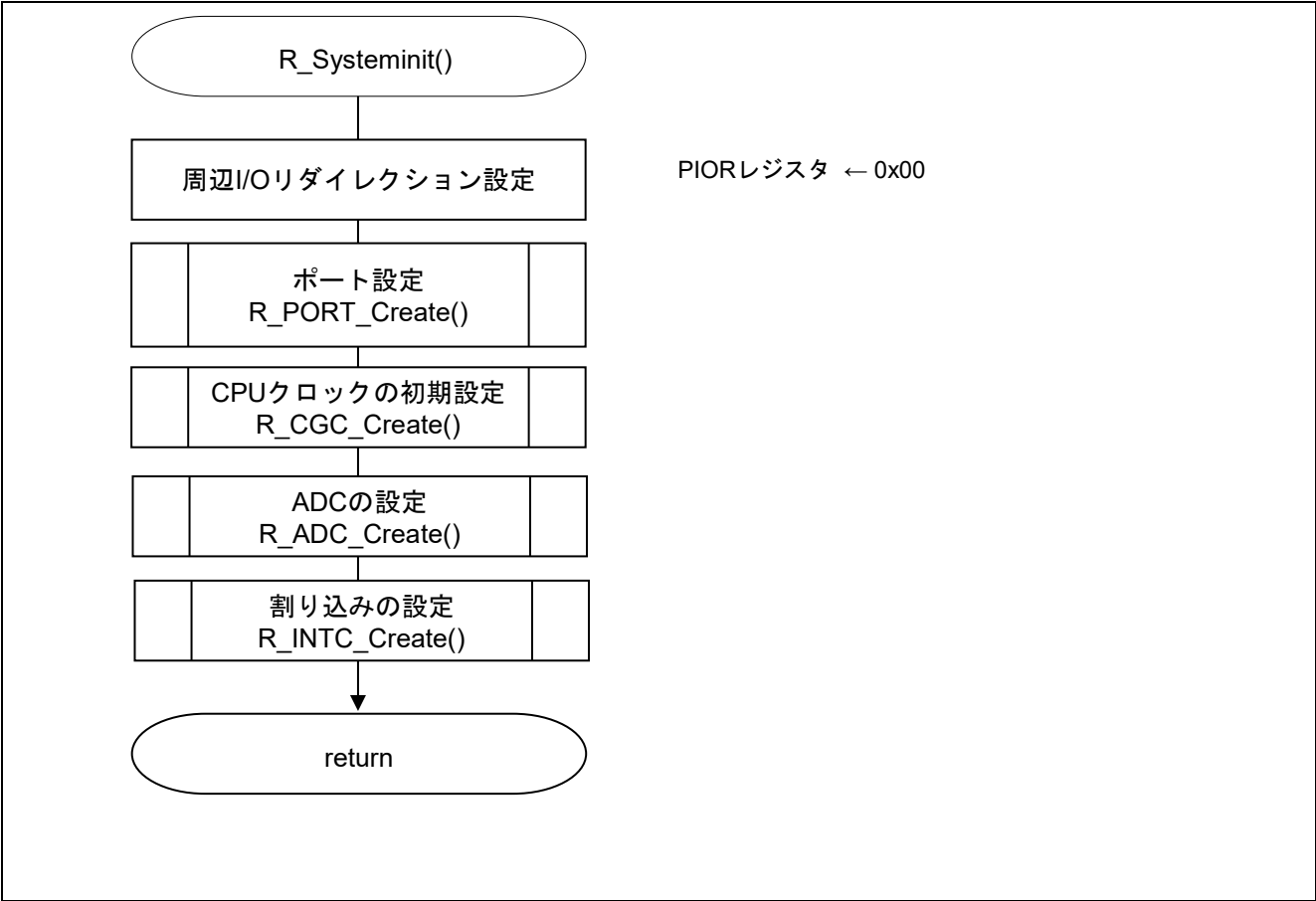
図 4.3 システム関数
