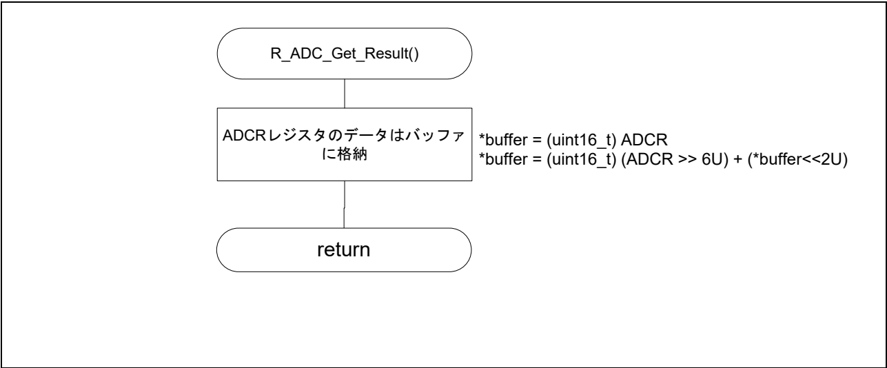
図 4.12 温度データを取得するフローチャート
