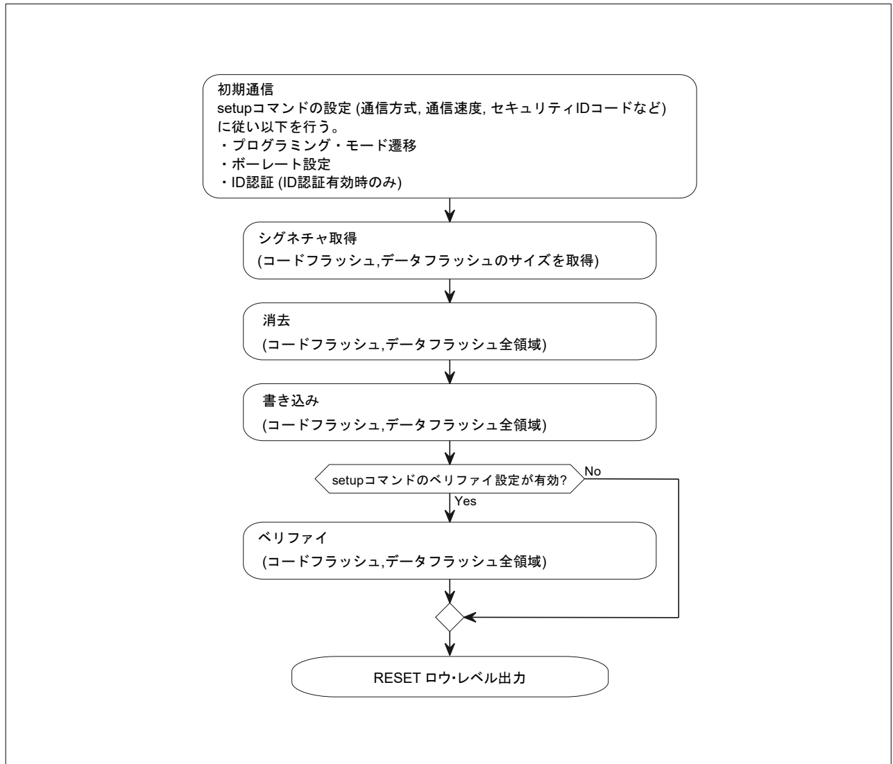
図 3-6 オフライン・モード
