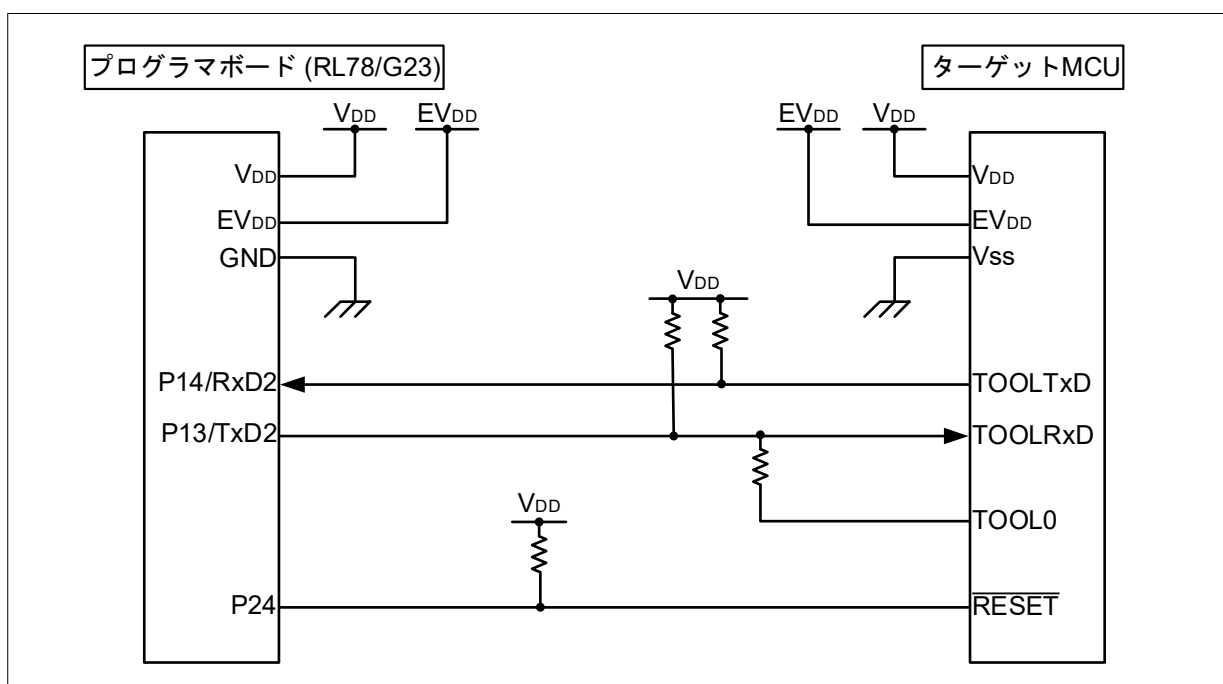
図 4-3 2 線 UART
