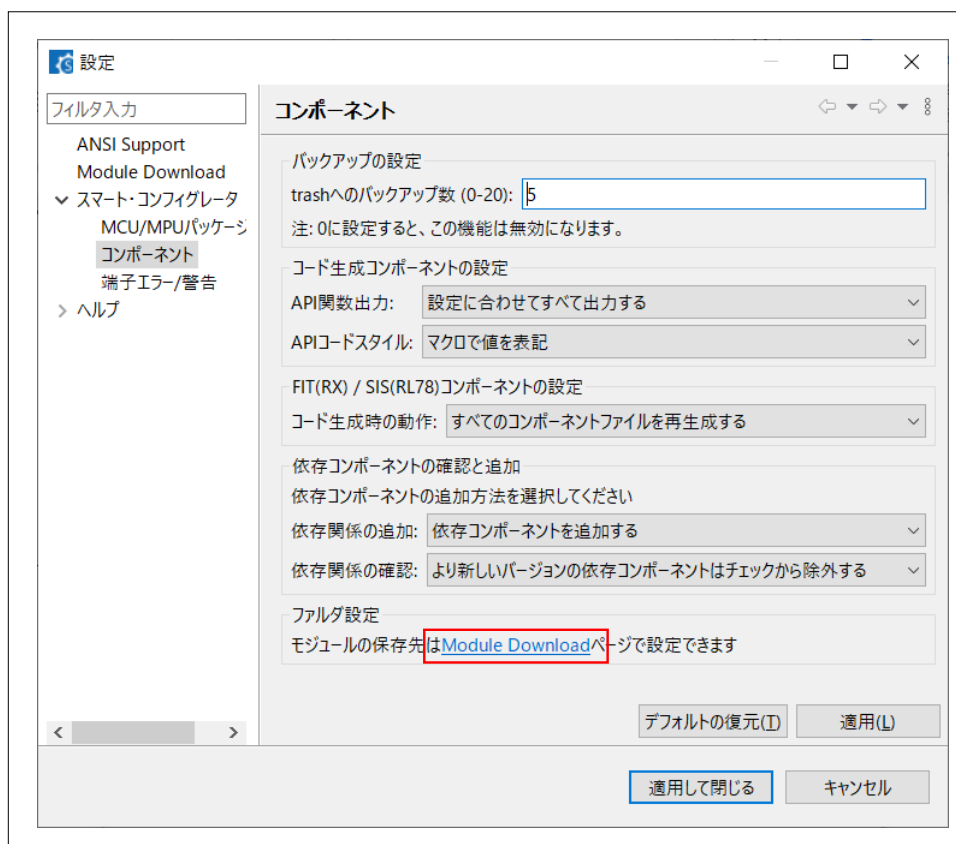
図 5-5 スマート・コンフィグレータ 「設定」ダイアログ (1/2)
