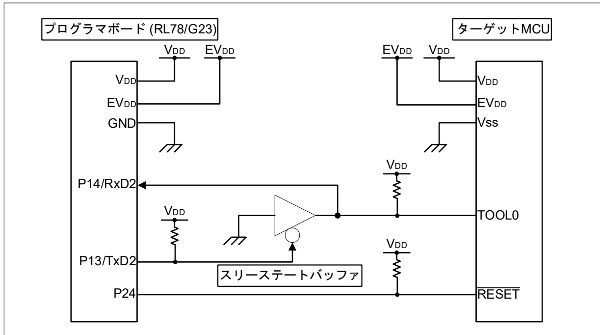
図 4-2 1 線 UART
