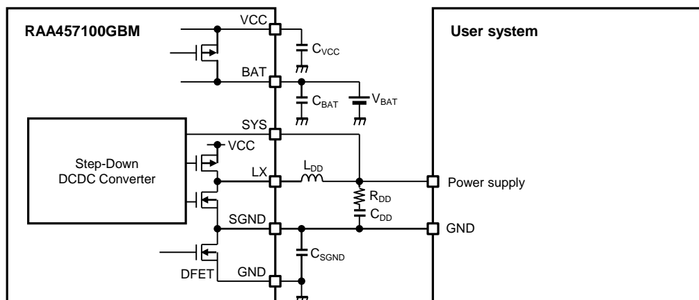
図1. DCDCコンバータ周辺回路図
