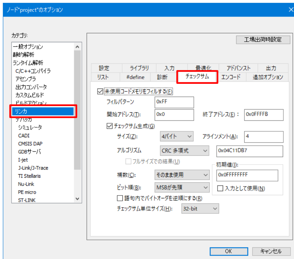
図 2.7 参照用 CRC の追加例（パラメータは MCU に合わせて設定してください）
