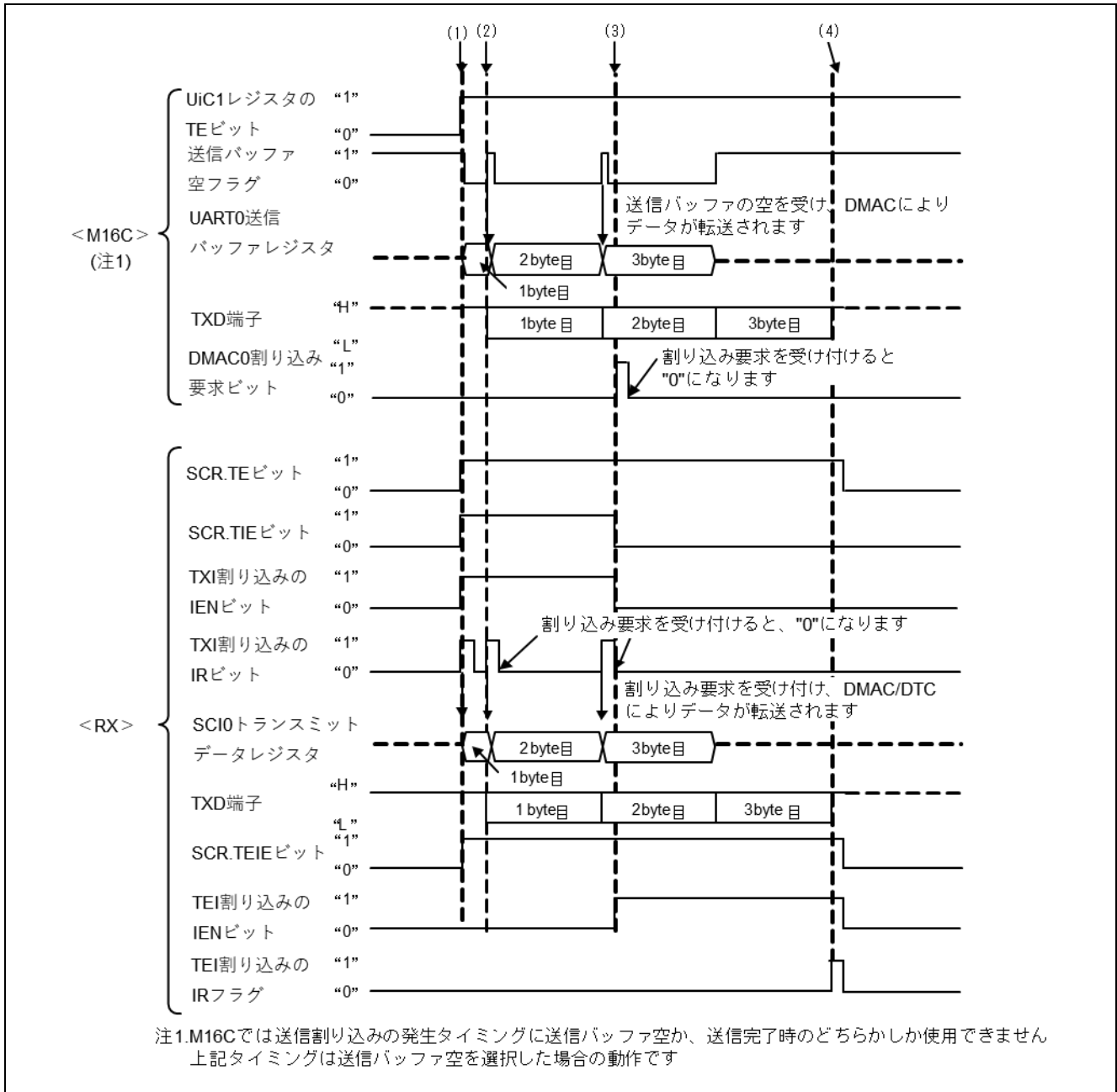
図 3.1 RX と M16C のタイミング相違点
