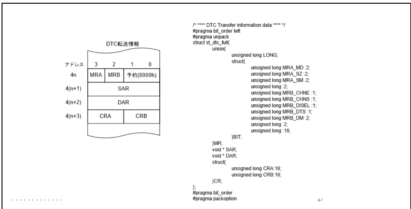
図 4.2 DTC 転送情報のメモリマップと構造体
