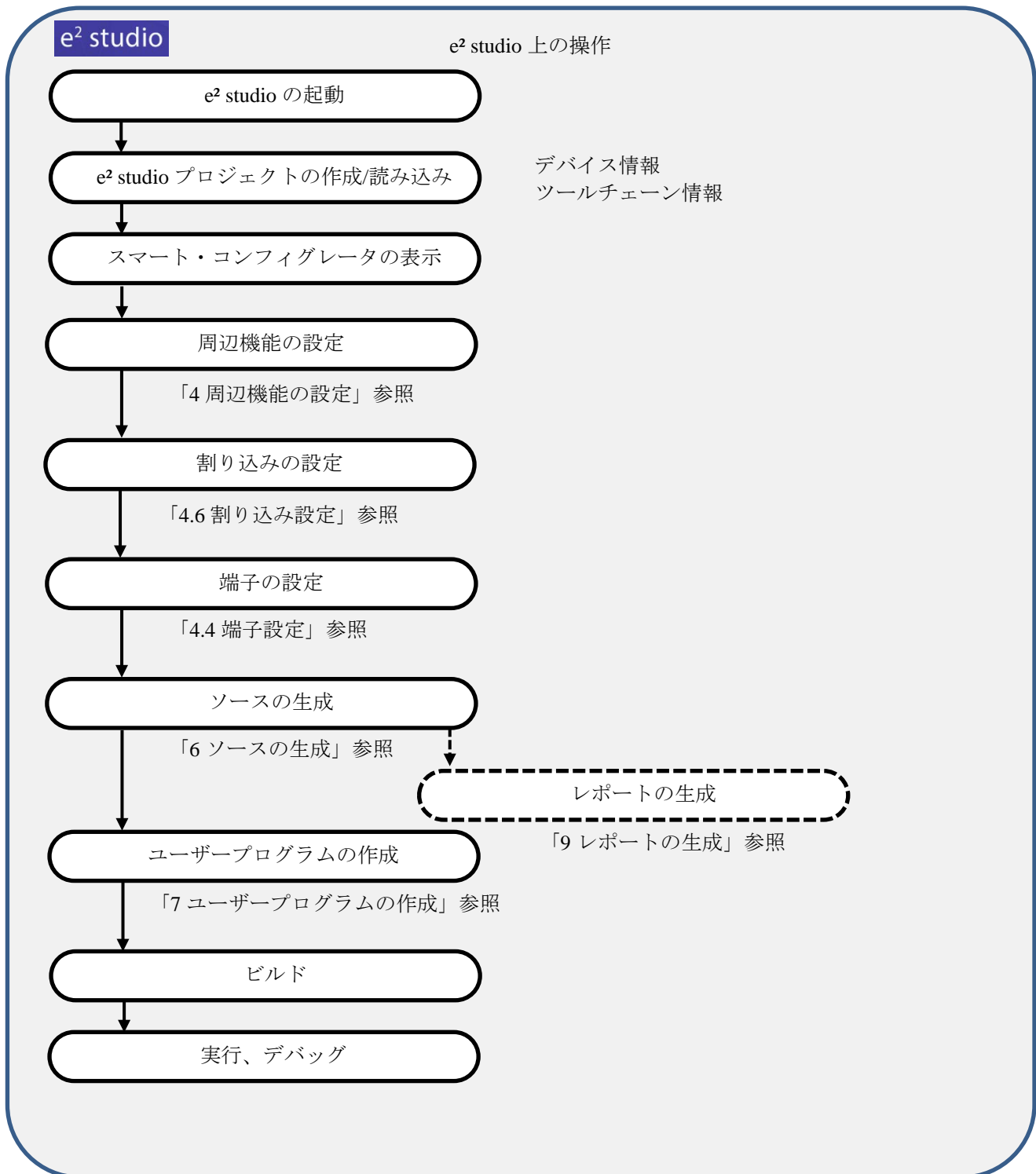
図 3-2 操作手順
