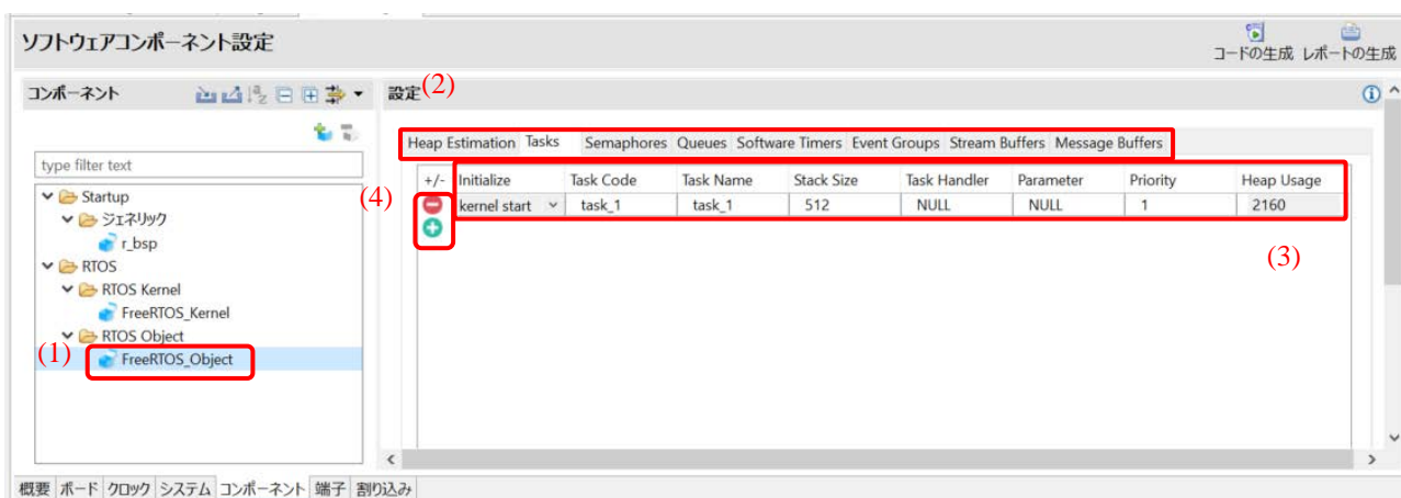
図 4-39 FreeRTOS_Object の設定
