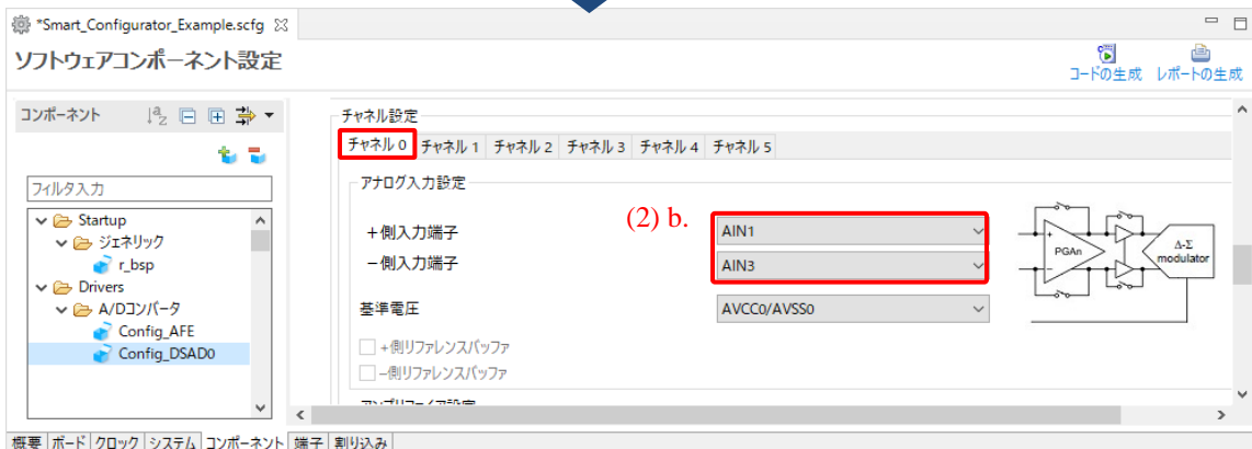
図 4-41 Config_DSAD0 の設定
