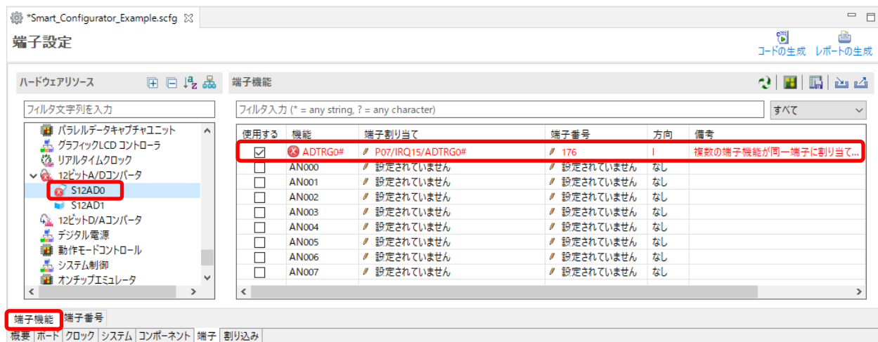
図 5-2 端子の競合
