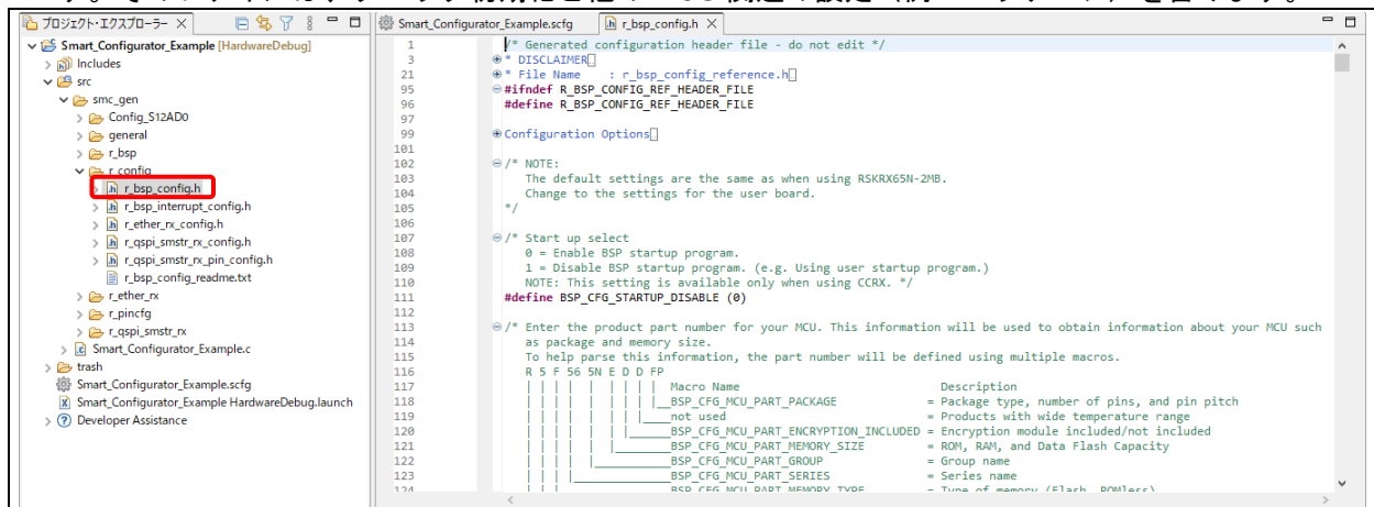
図 6-12 r_bsp_config.h
