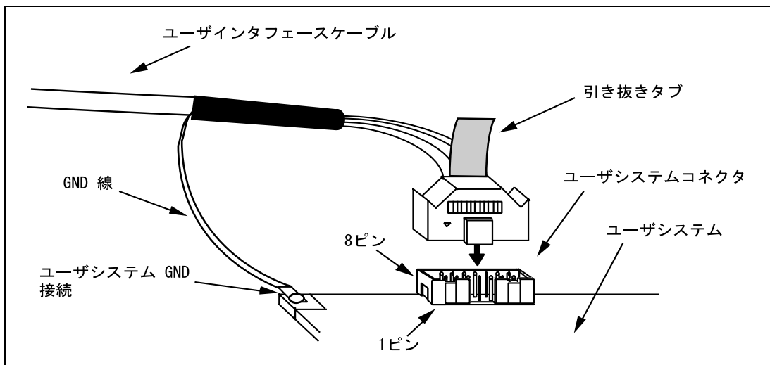
図 1.1 14 ピンストレータイプコネクタ使用時のユーザシステム側のユーザインタフェースケーブル接続方法
