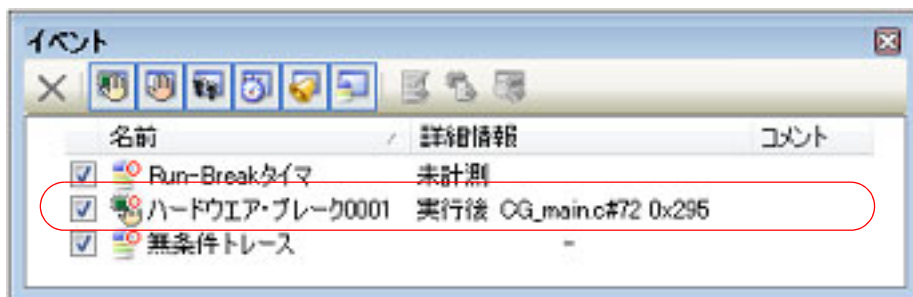
図 2.38 イベントパネルのハードウェア・ブレーク・イベント（実行系）の設定例
