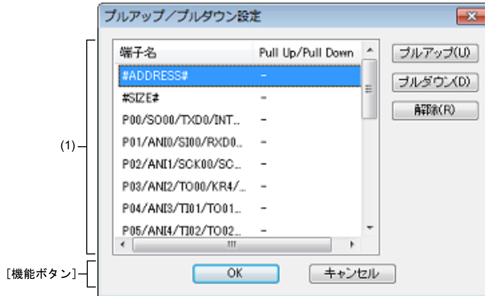
図 A.87 プルアップ／プルダウン設定 ダイアログ
