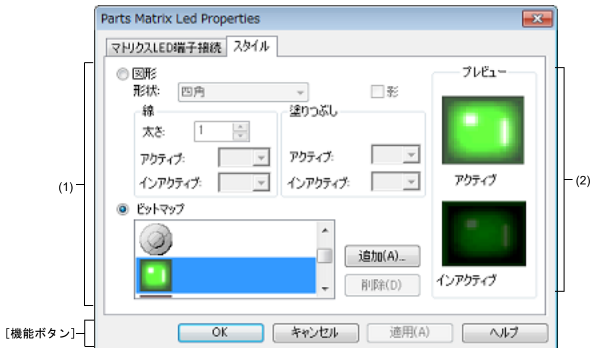
図 A.82 Parts Matrix Led Properties ダイアログ : [スタイル] タブ
