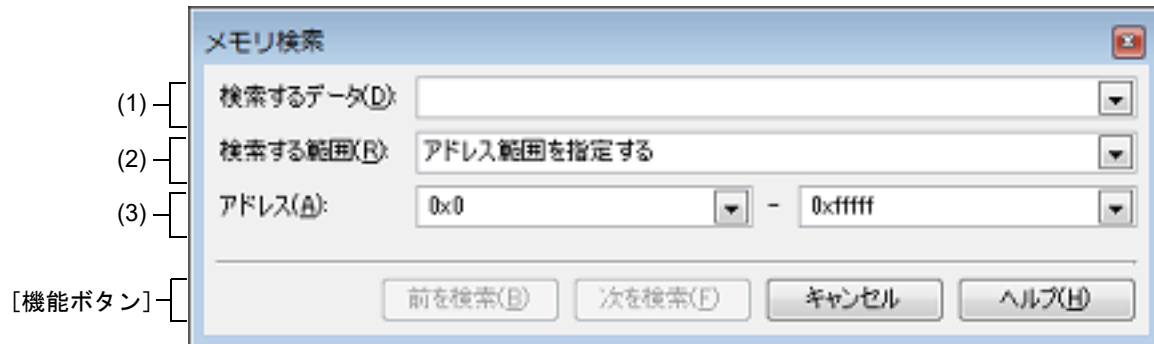
図 A.28 メモリ検索 ダイアログ
