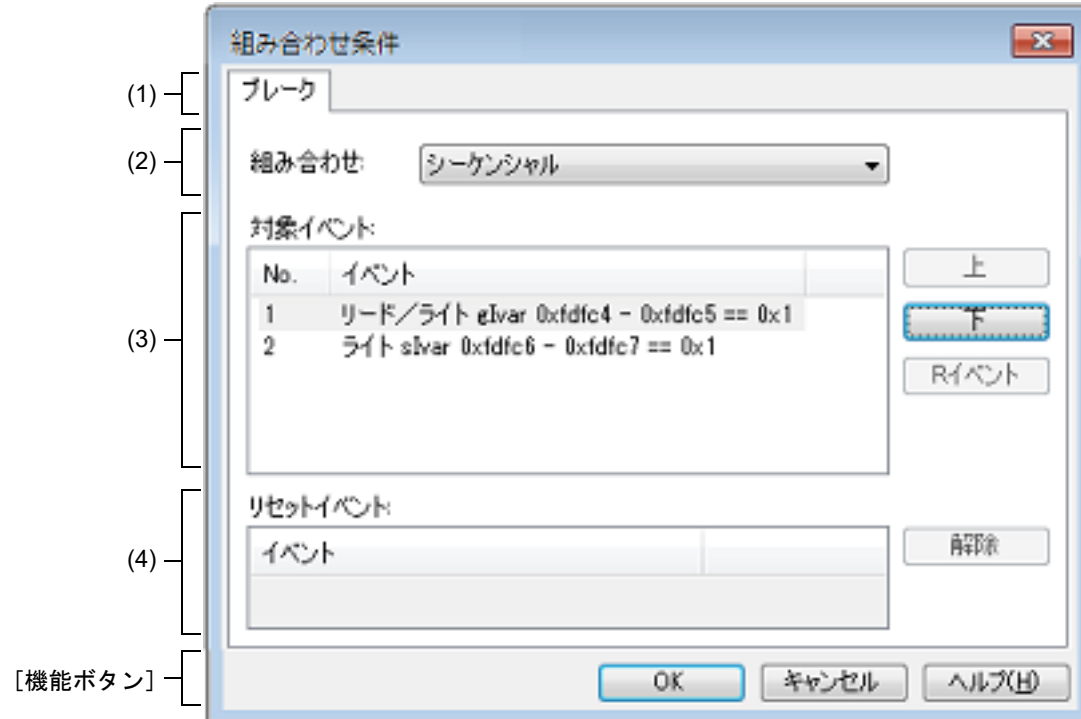
図 A.33 組み合わせ条件 ダイアログ
