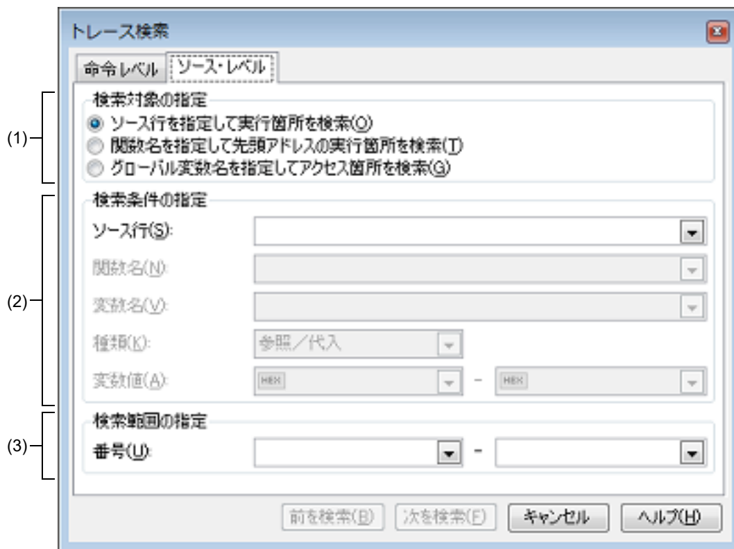
図 A.32 トレース検索 ダイアログ : [ソース・レベル] タブ
