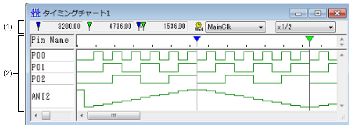
図 A.59 タイミングチャート ウィンドウ
