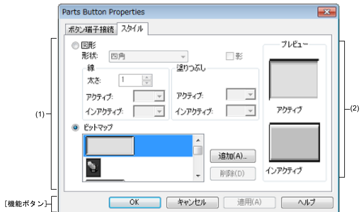
図 A.64 Parts Button Properties ダイアログ : [スタイル] タブ
