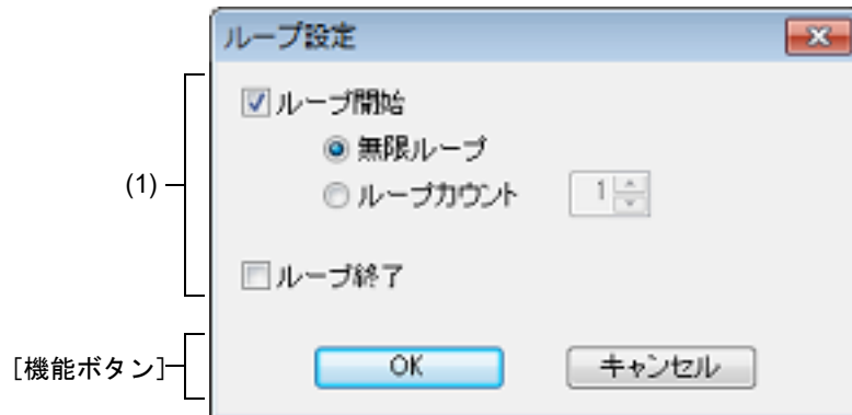
図 A.57 ループ設定 ダイアログ
