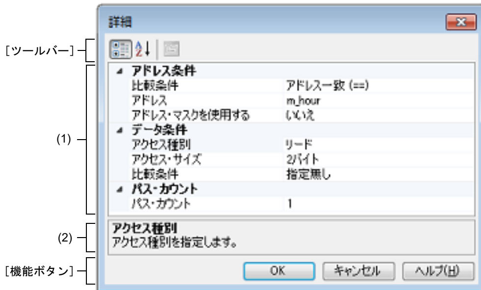
図 A.39 詳細 ダイアログ (アクセス・イベント) 【シミュレータ】
