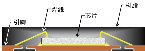
图1-8 剖面结构图
