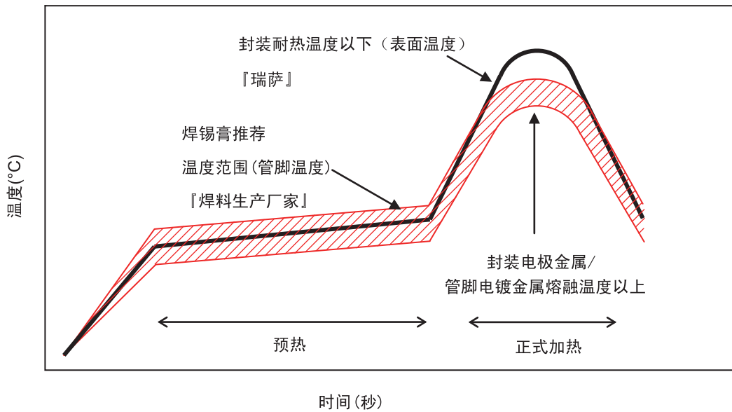
图5-2 焊接温度
