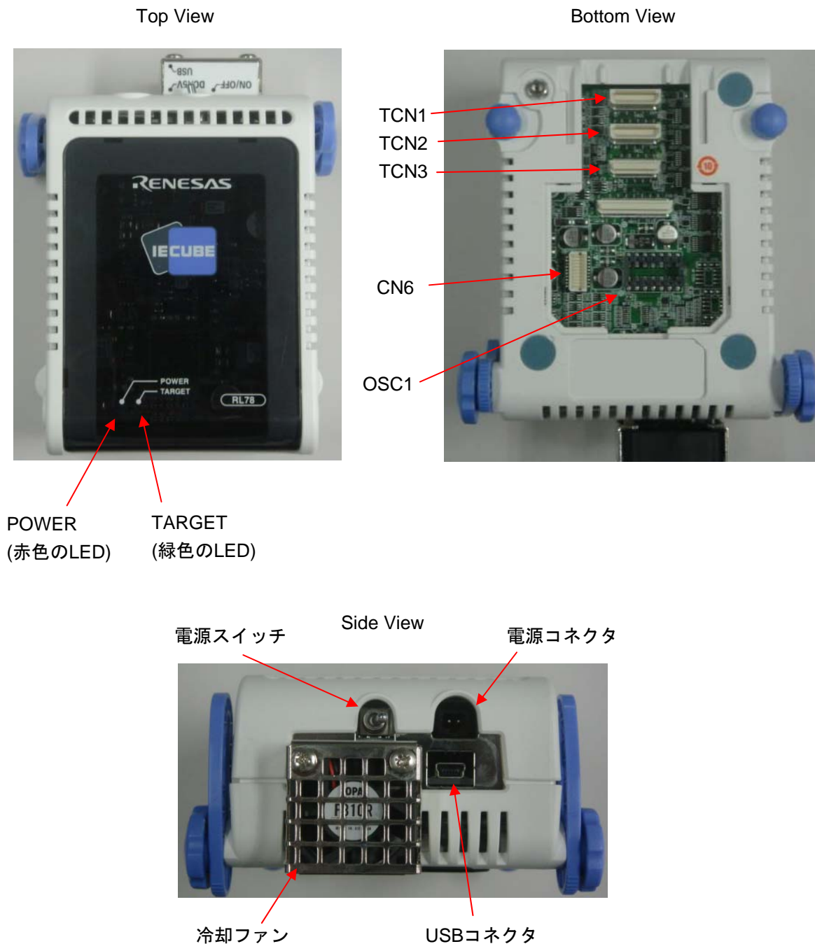
図1-1 QB-RL78I1Aの各部の名称
