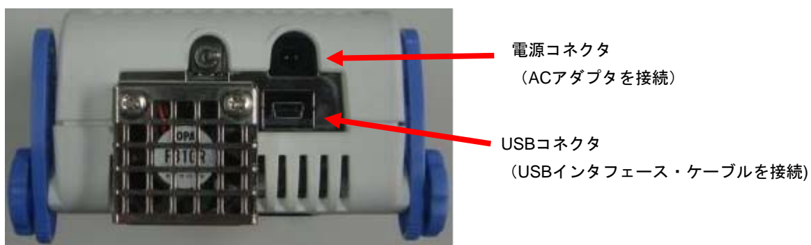
図2-8 コネクタ位置
