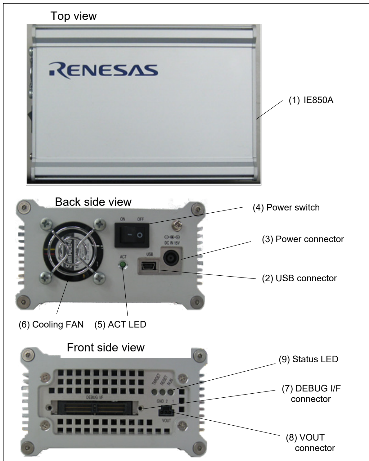
図 2-1 IE850A (RTE0T0850AKCT00000J) 各部の名称
