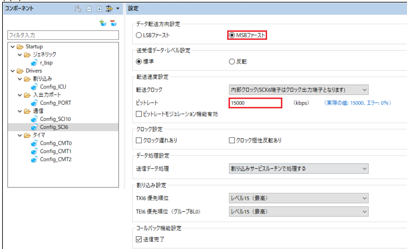
図 4-40 Config_SCI6 設定
