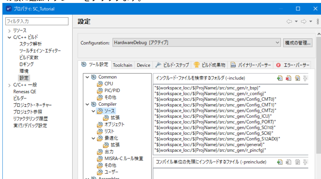
図 5-2 インクルードパス追加
