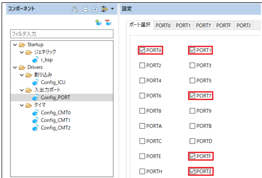
図 4-25 ポート選択
