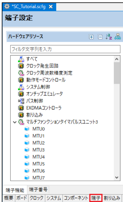
図 4-45 端子ページ
