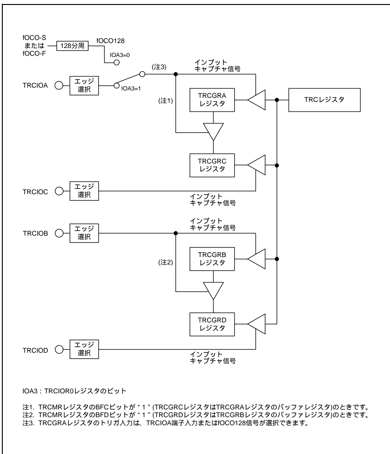
図 19.7 インputキャプチャ機能のブロック図
