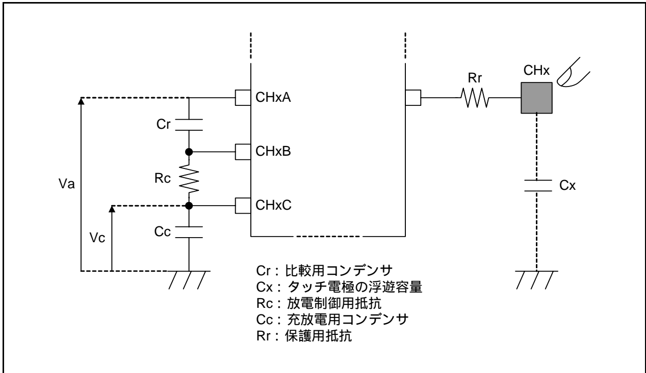
図27.5 計測部回路
