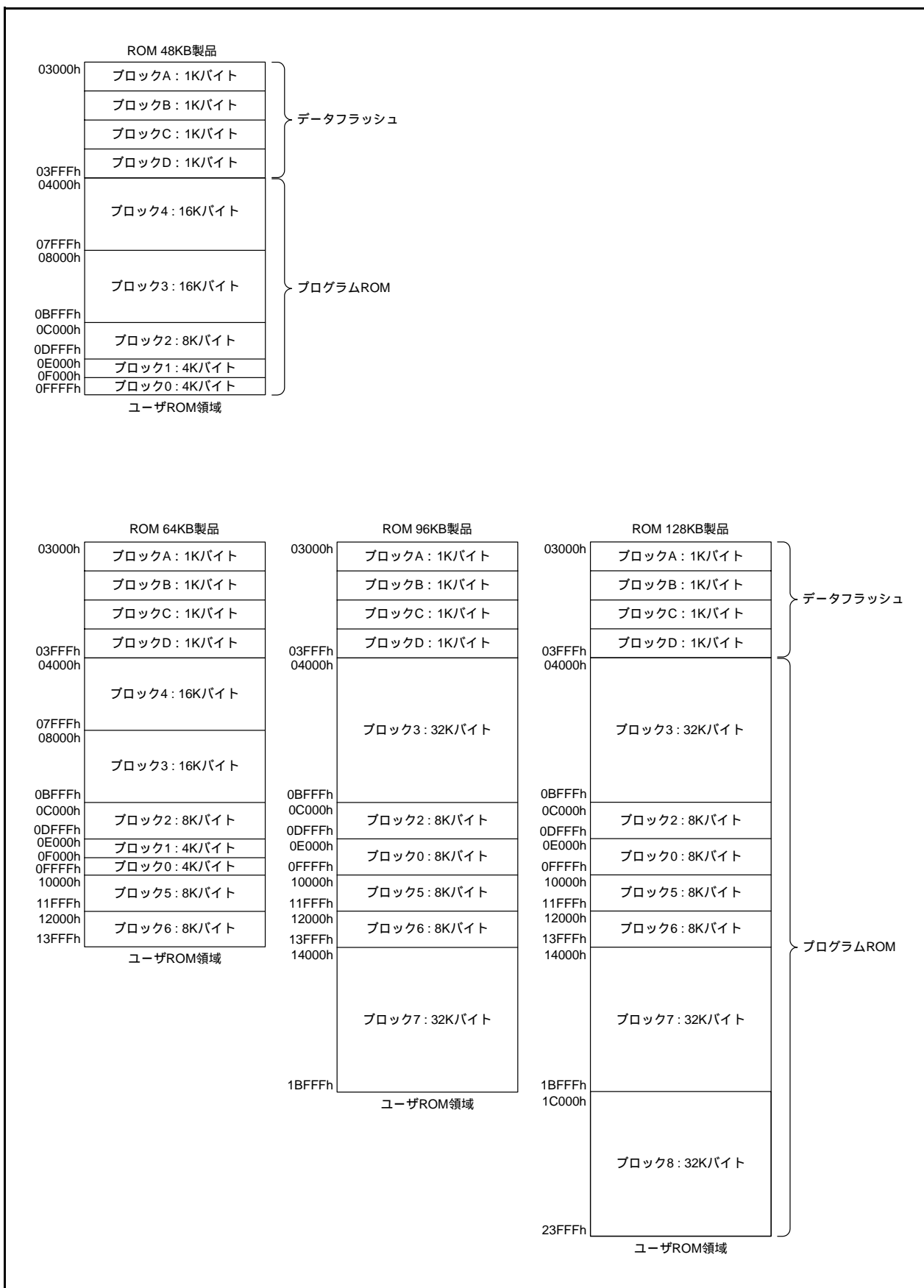
図28.1 R8C/3NTグループのフラッシュメモリのブロック図
