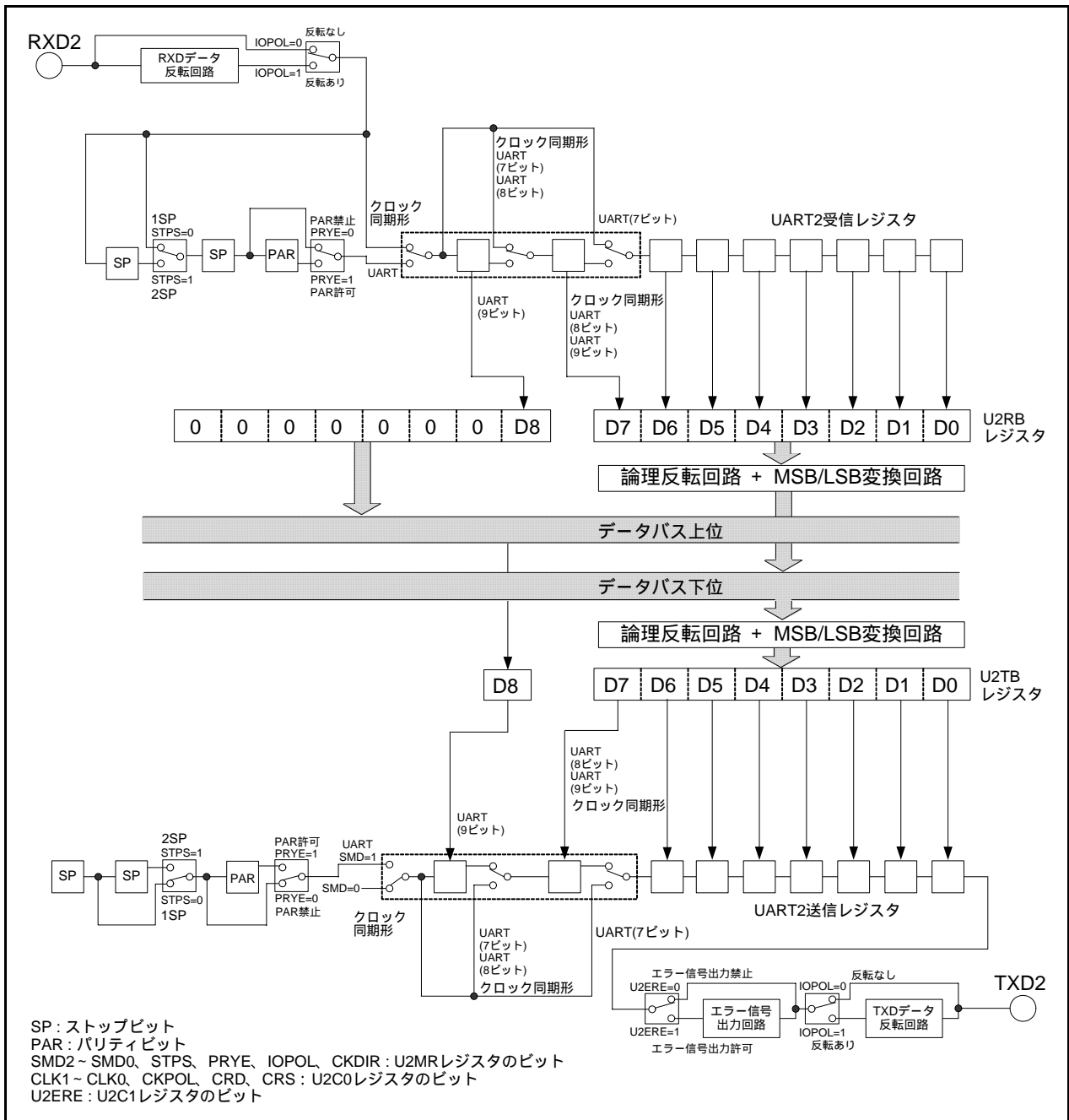
図22.2 UART2送受信部のブロック図
