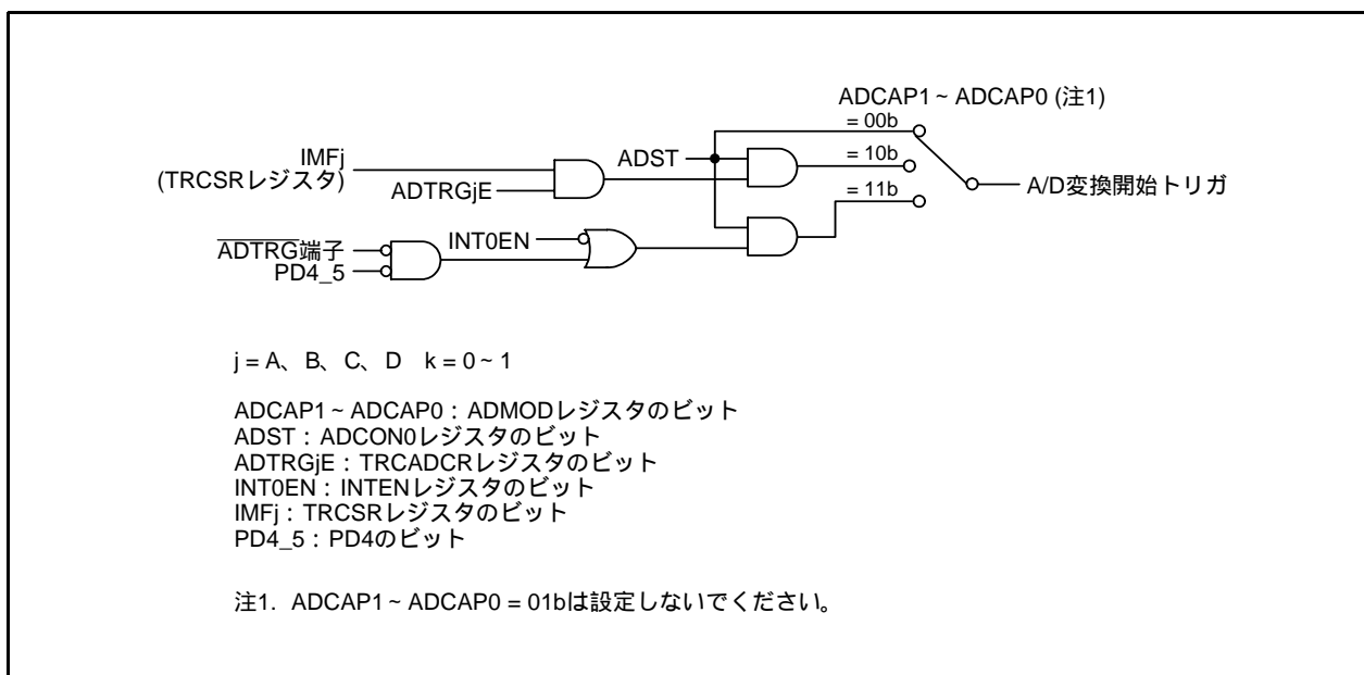
図26.4 A/D変換開始制御部のブロック図
