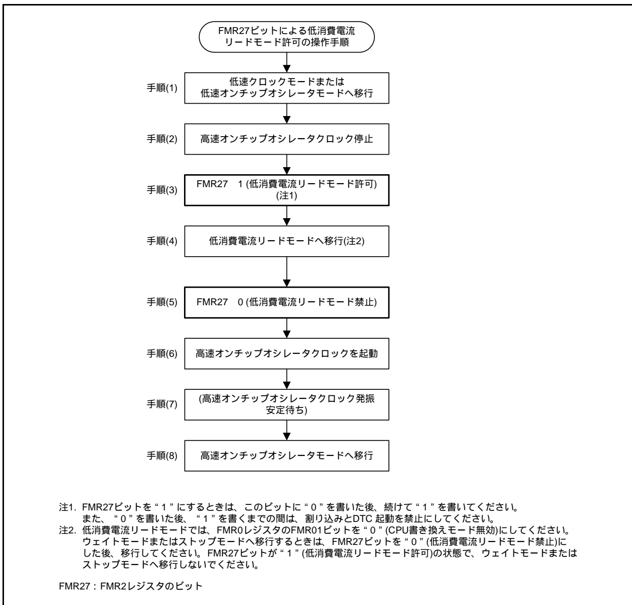
図29.3 低消費電流リードモードの操作手順例
