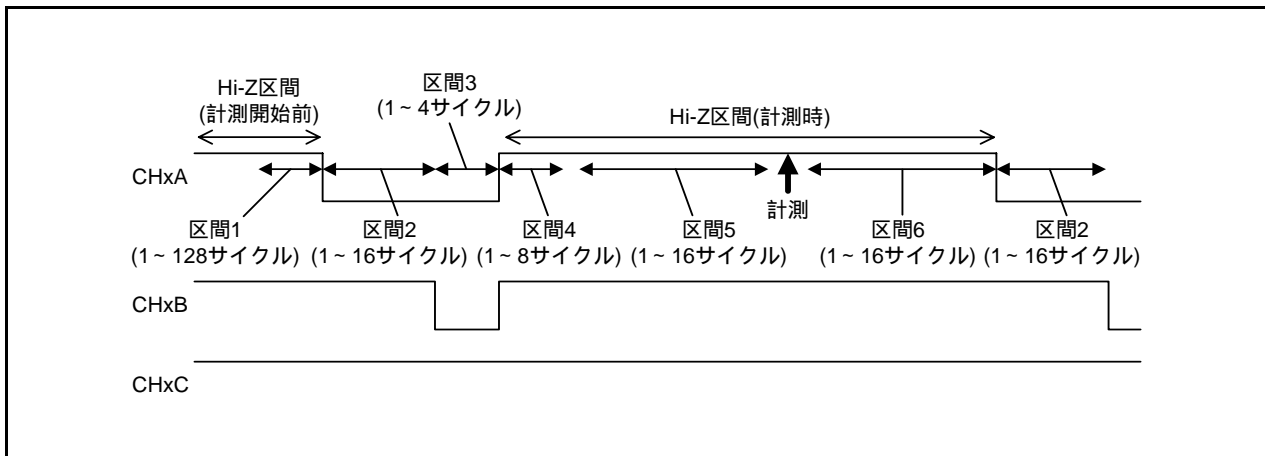
図27.3 ステータス区間調整
