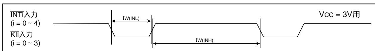
図30.15 VCC = 3V時の外部割り込み \overline{INTi} およびキー入力割り込み \overline{Kli} 入力タイミング
