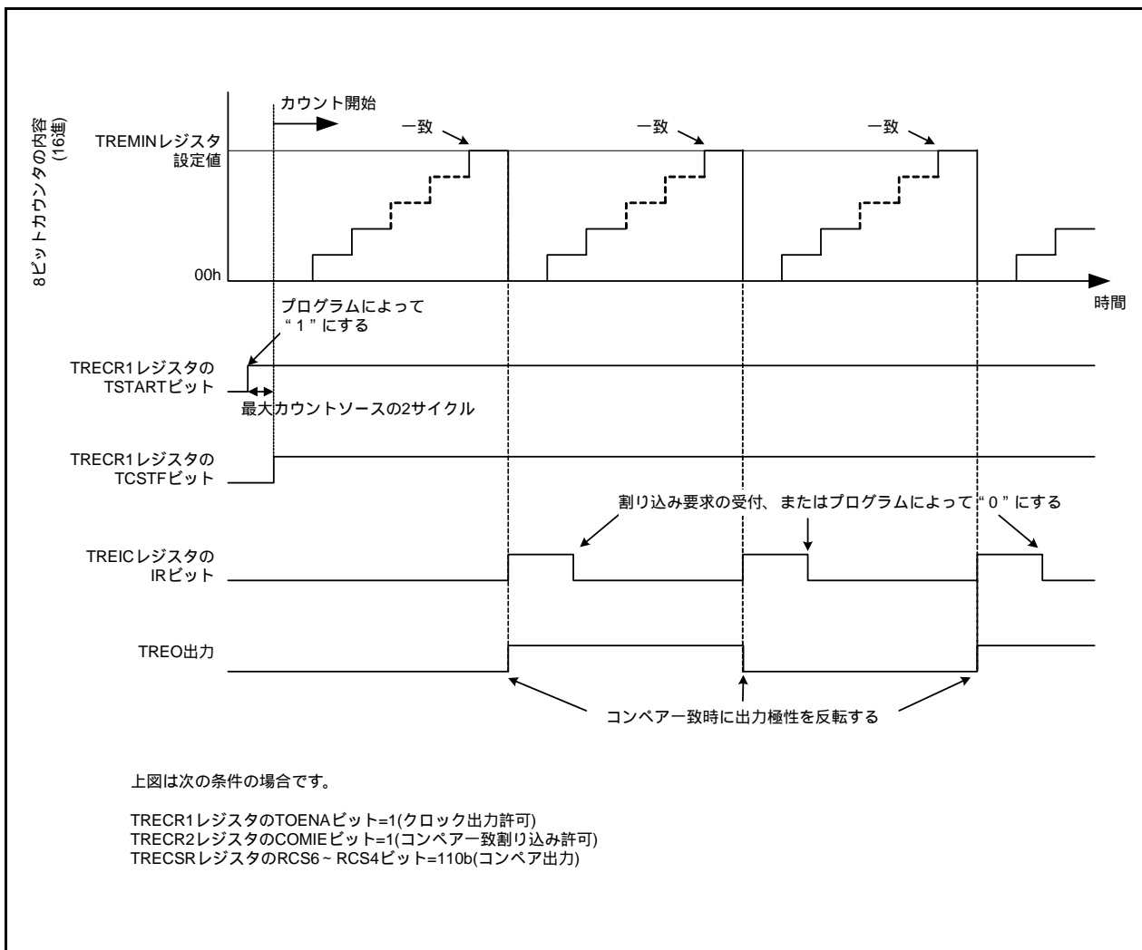
図20.5 アウトプットコンペアーモードの動作例
