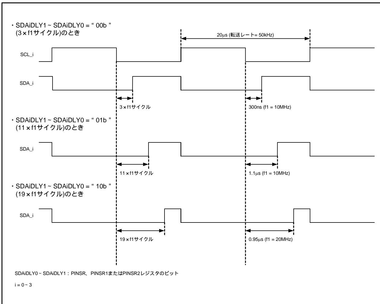
図25.3 SDA i (i = 0 ~ 3)端子のデジタル遅延の動作例
