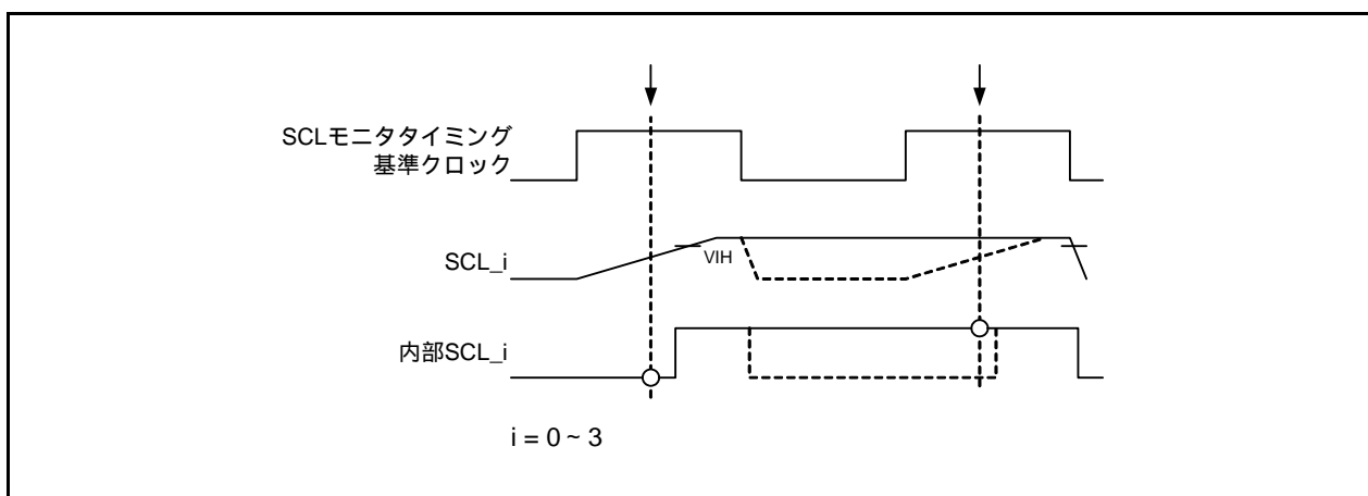
図25.21 ビット同期回路のタイミング
