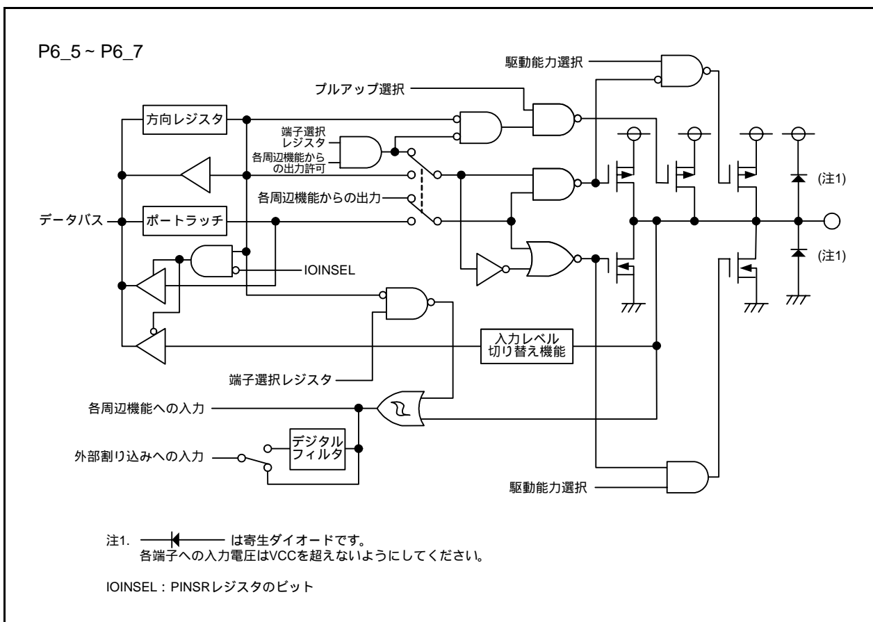
図7.14 I/Oポートの構成(14)
