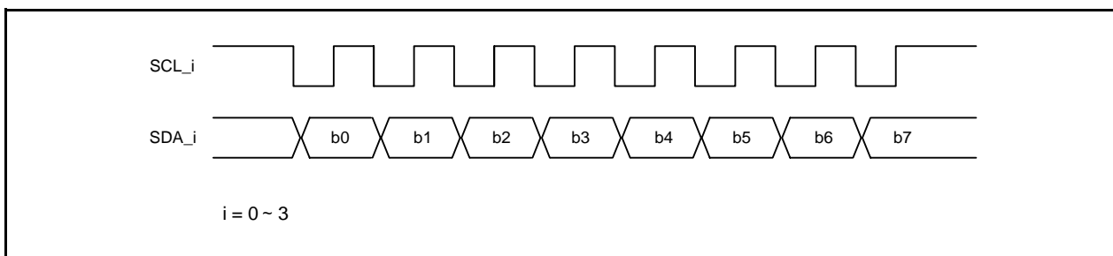
図25.13 クロック同期式シリアルフォーマットの転送フォーマット
