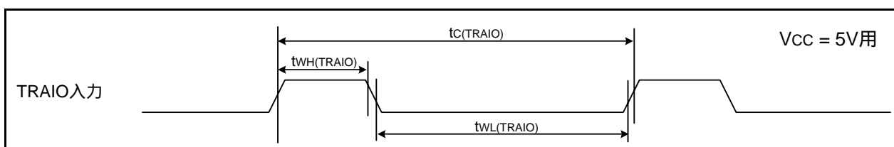
図30.9 V_{CC} = 5V 時のTRAIO入力タイミング
