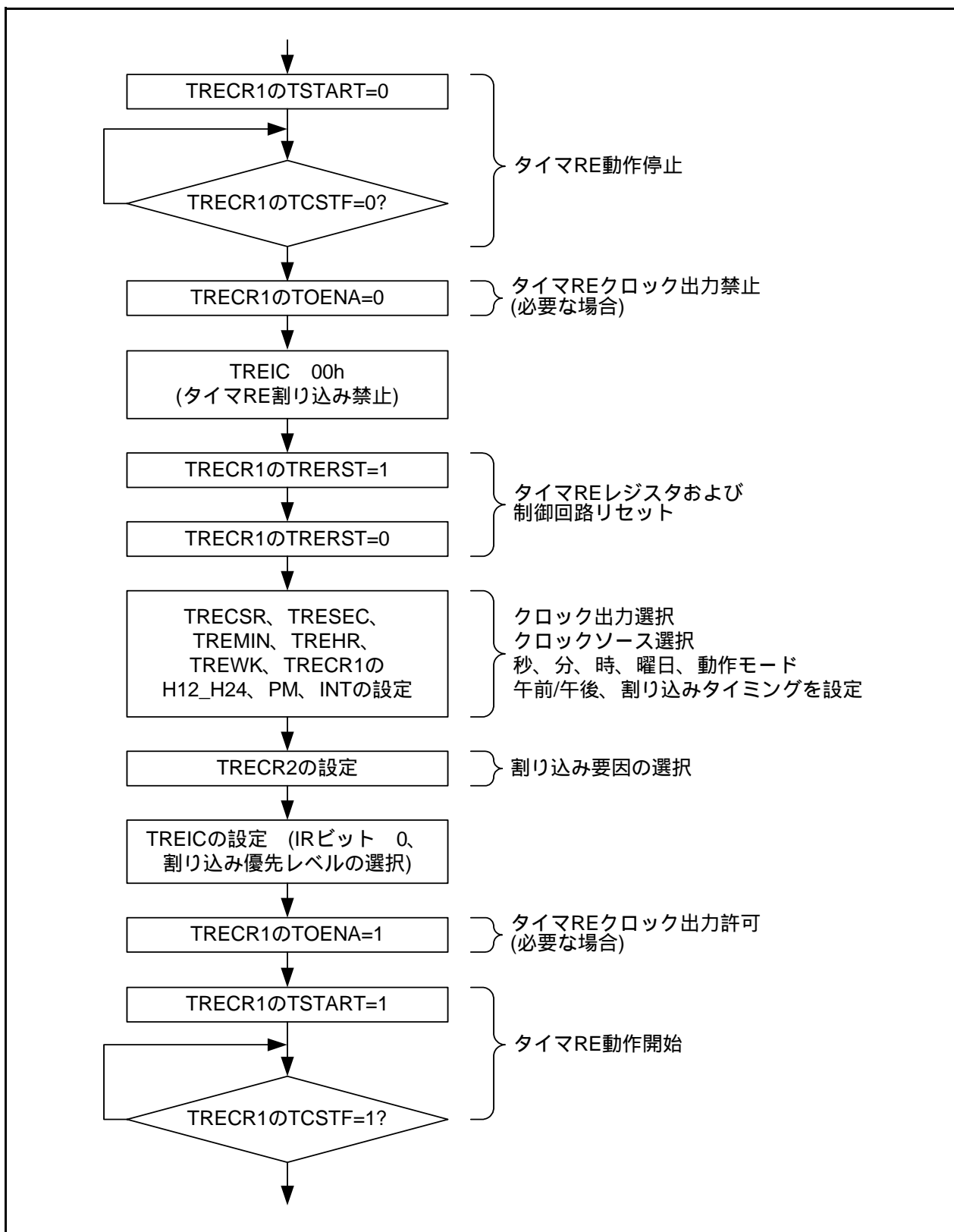
図31.2 リアルタイムクロックモード時の設定例
