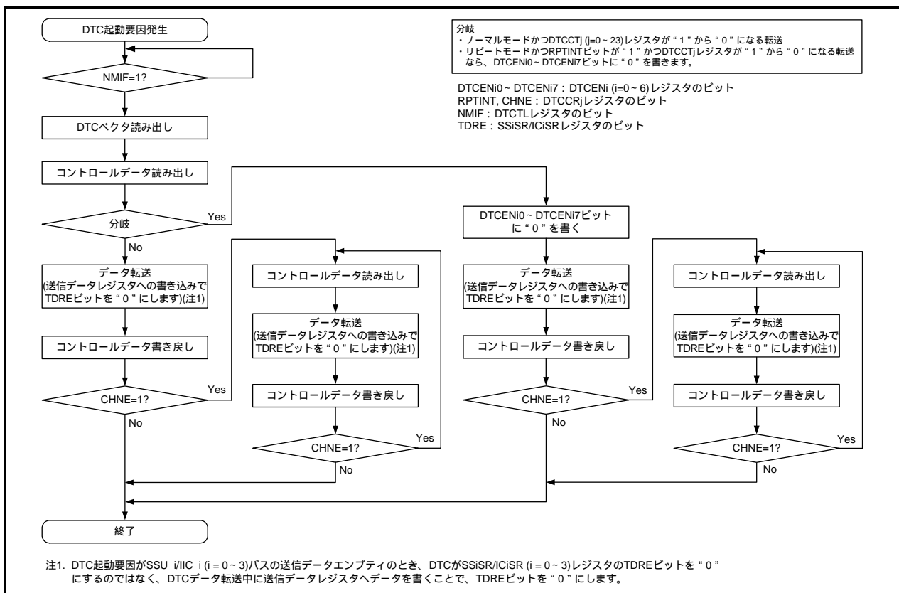
図 15.6 DTC 起動要因が SSU_i/iIC_i (i = 0 ~ 3) の送信データエンptyであるときの DTC 内部動作フローチャート
