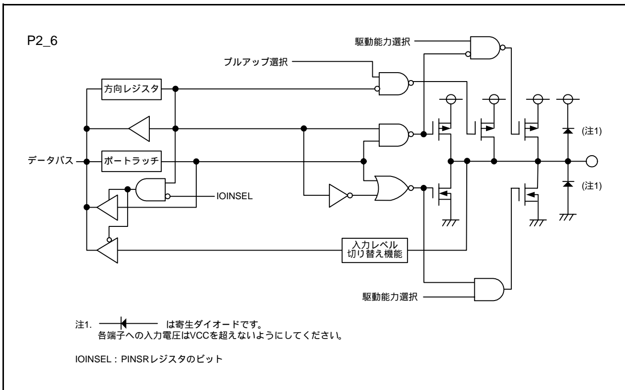
図7.6 I/Oポートの構成(6)
