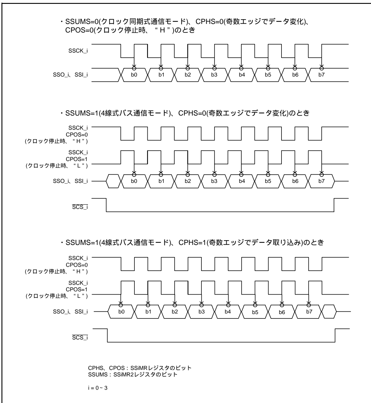
図24.2 転送クロックの極性、位相および転送データの関係
