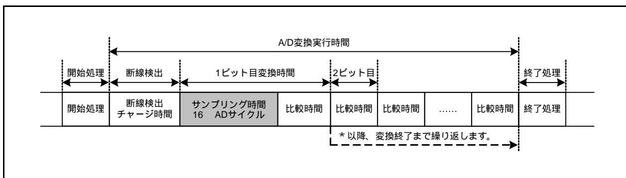
図26.2 A/D変換タイミング図
