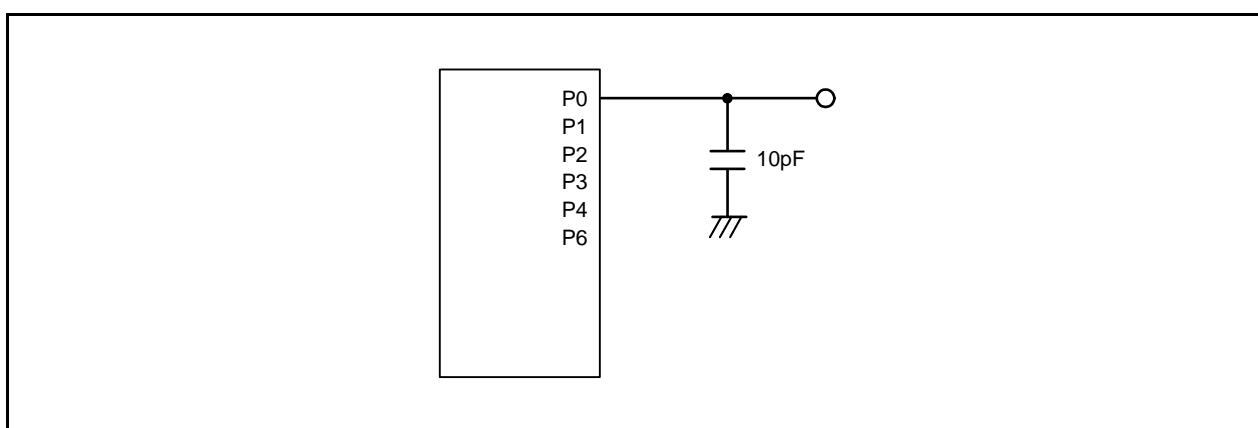
図30.1 ポートP0～P4、P6のタイミング測定回路
