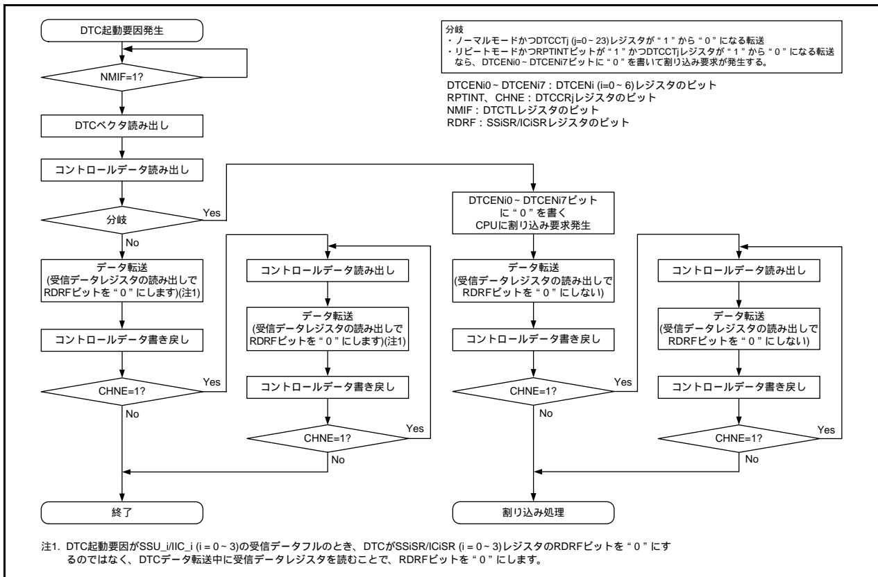
図 15.5 DTC 起動要因が SSU_i/iIC_i (i = 0 ~ 3) の受信データフルであるときの DTC 内部動作フローチャート
