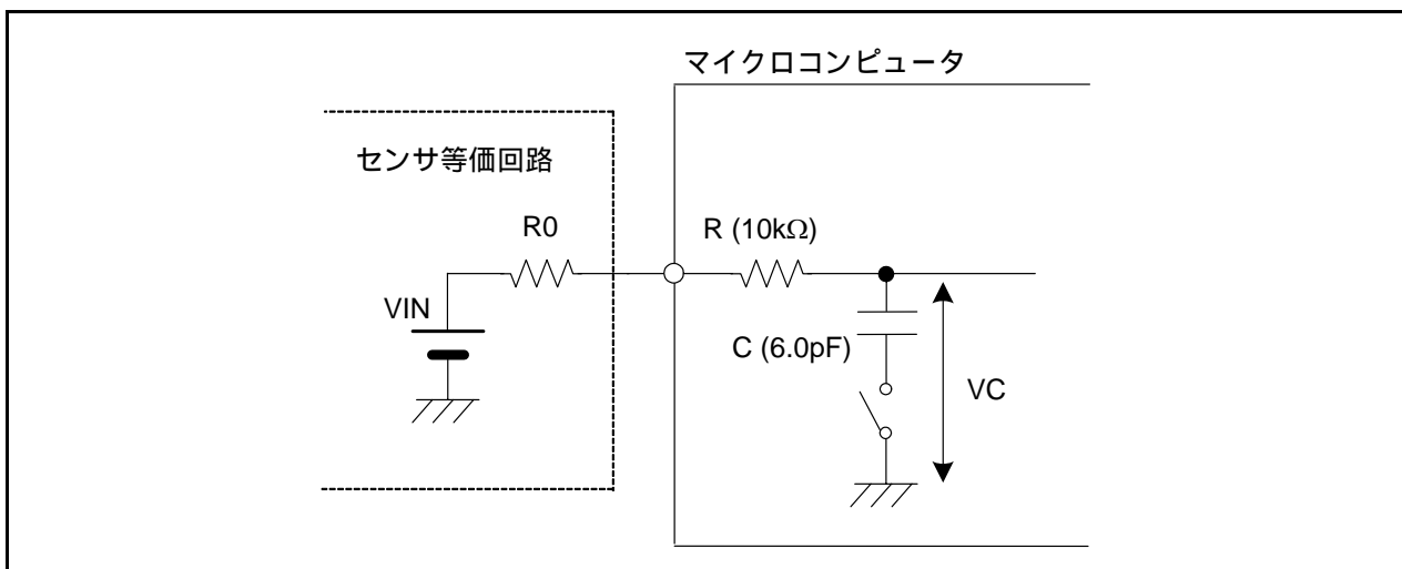
図26.10 アナログ入力端子と外部センサの等価回路例
