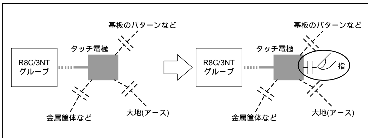
図27.1 指による浮遊容量の増加
