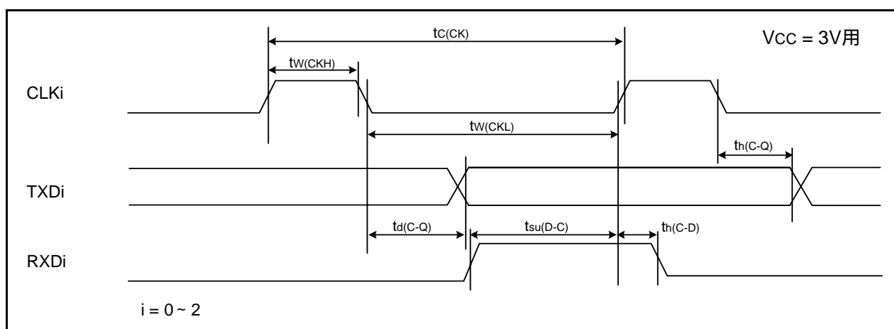
図30.14 VCC = 3V時のシリアルインタフェースのタイミング
