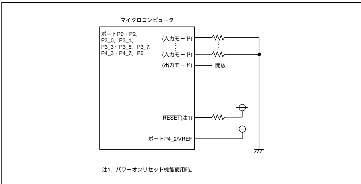
図7.16 未使用端子の処理例
