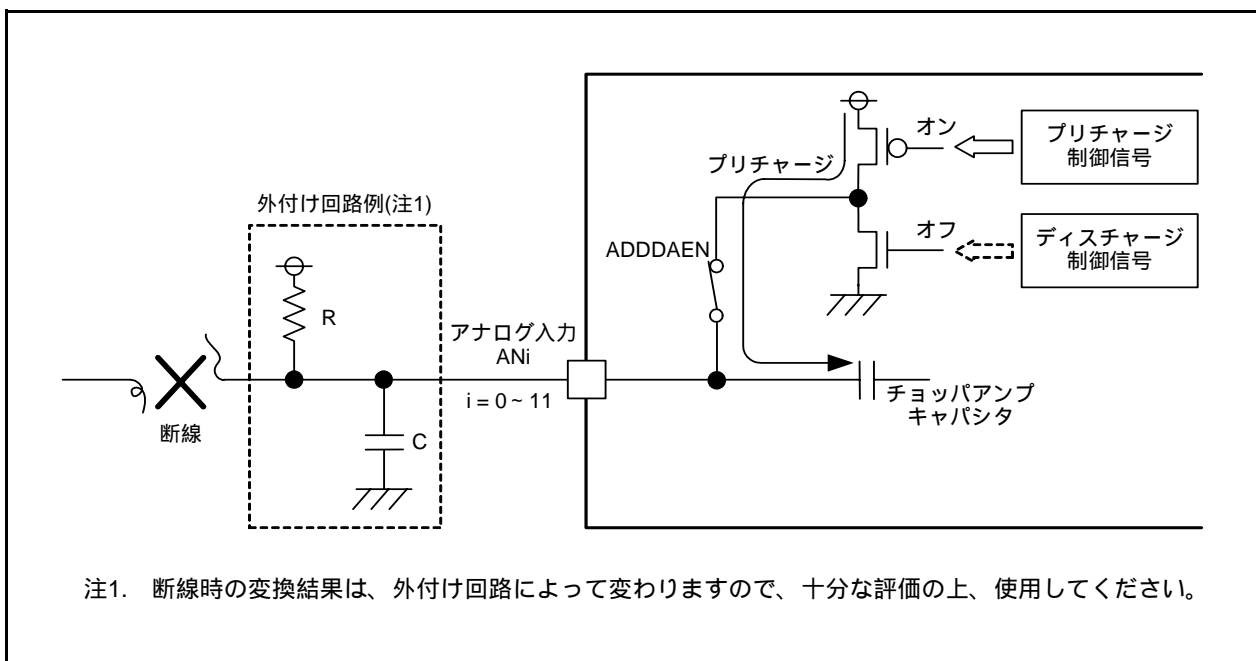
図26.5 AVCC側でのA/D断線検出例(変換前プリチャージを選択)
