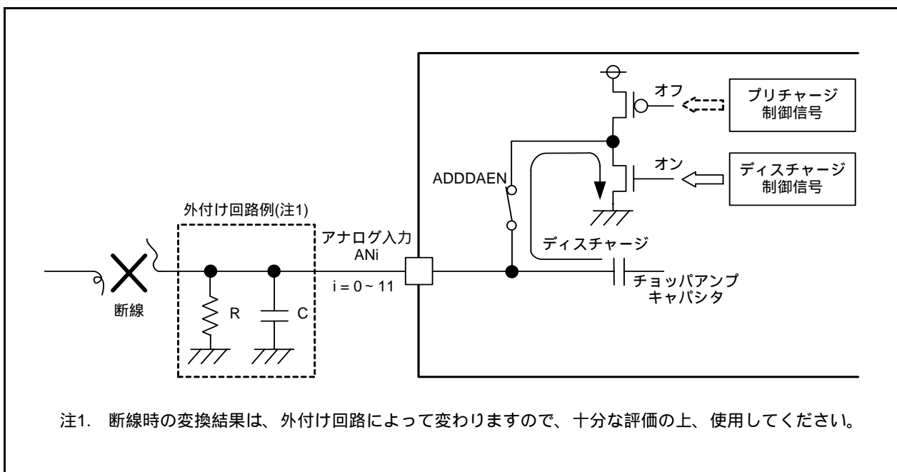
図26.6 AVSS側でのA/D断線検出例(変換前ディスチャージを選択)
