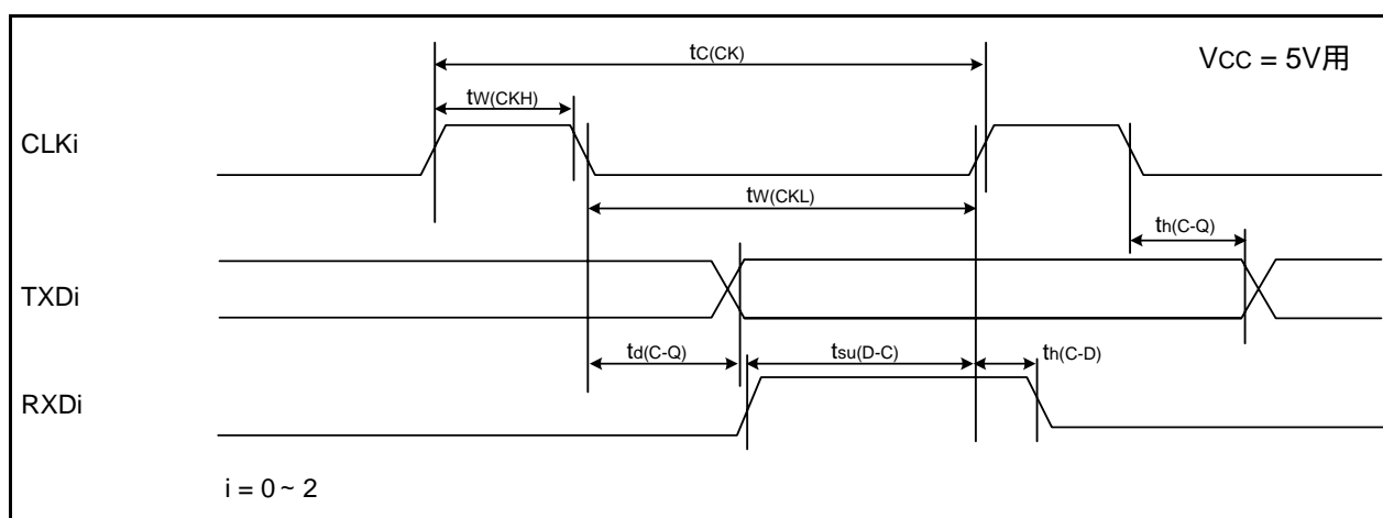
図30.10 VCC = 5V時のシリアルインタフェースのタイミング
