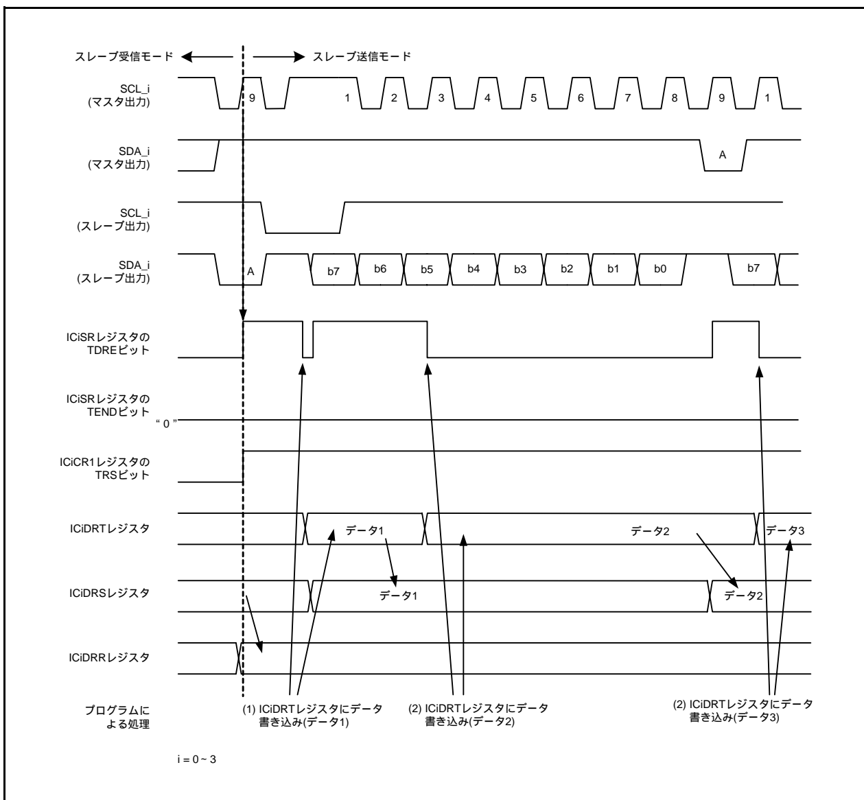
図25.9 スレープ送信モードの動作タイミング(I 2 Cバスインタフェースモード)(1)
