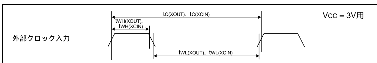
図30.12 V_{CC} = 3V 時の外部クロック入力タイミング
