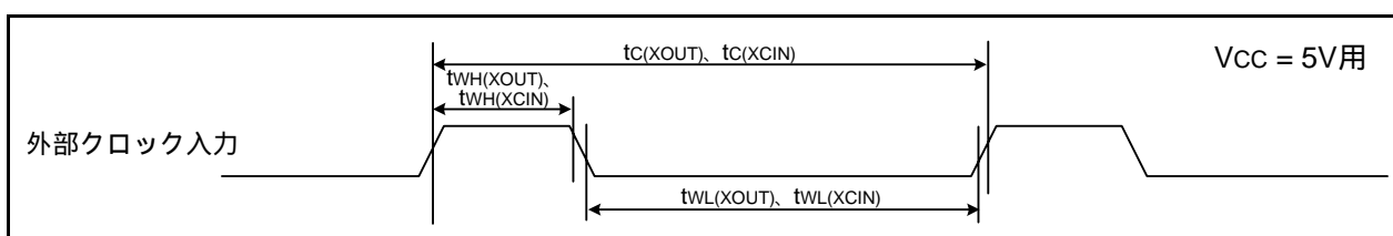
図30.8 V_{CC} = 5V 時の外部クロック入力タイミング
