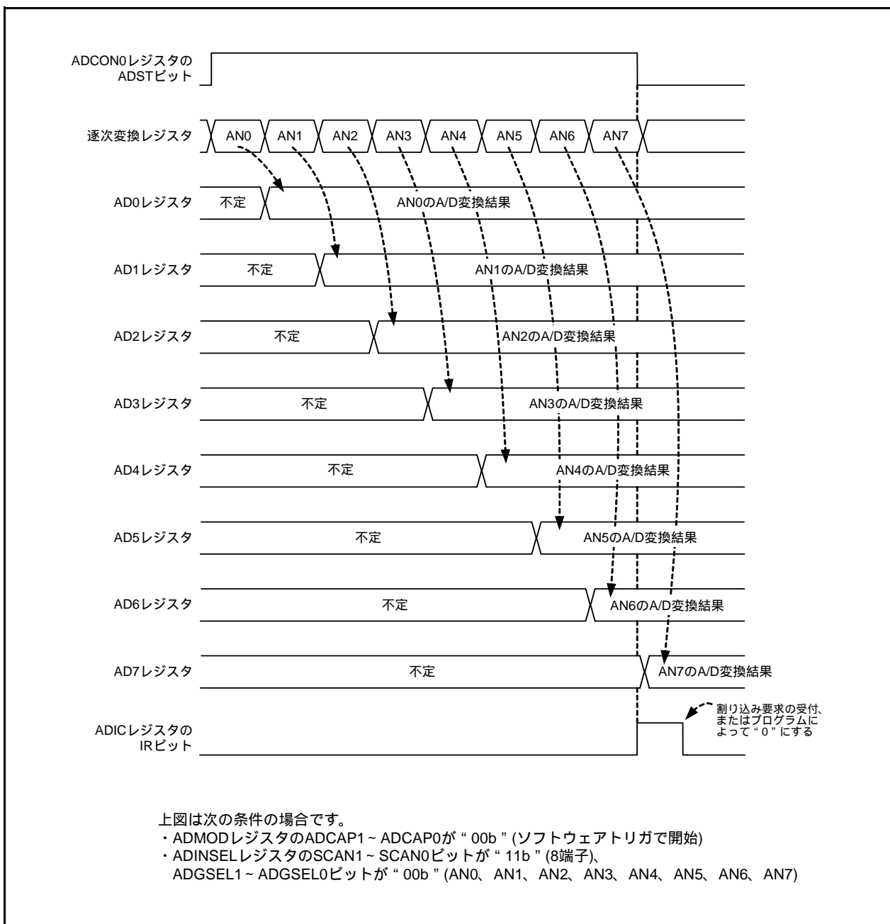
図26.8 単掃引モード時の動作例
