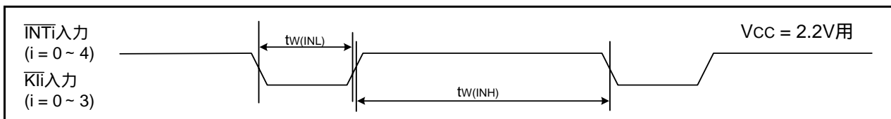
図 30.19 Vcc = 2.2V時の外部割り込みINTiおよびキー入力割り込みKli入力タイミング
