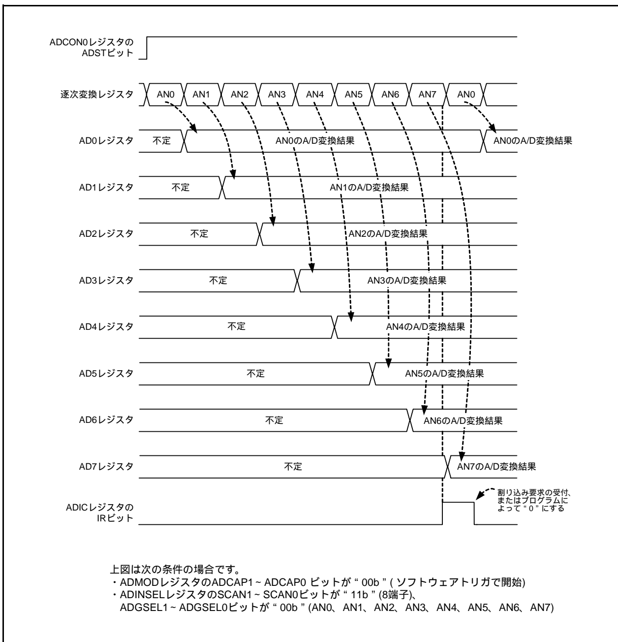
図26.9 繰り返し掃引モード時の動作例
