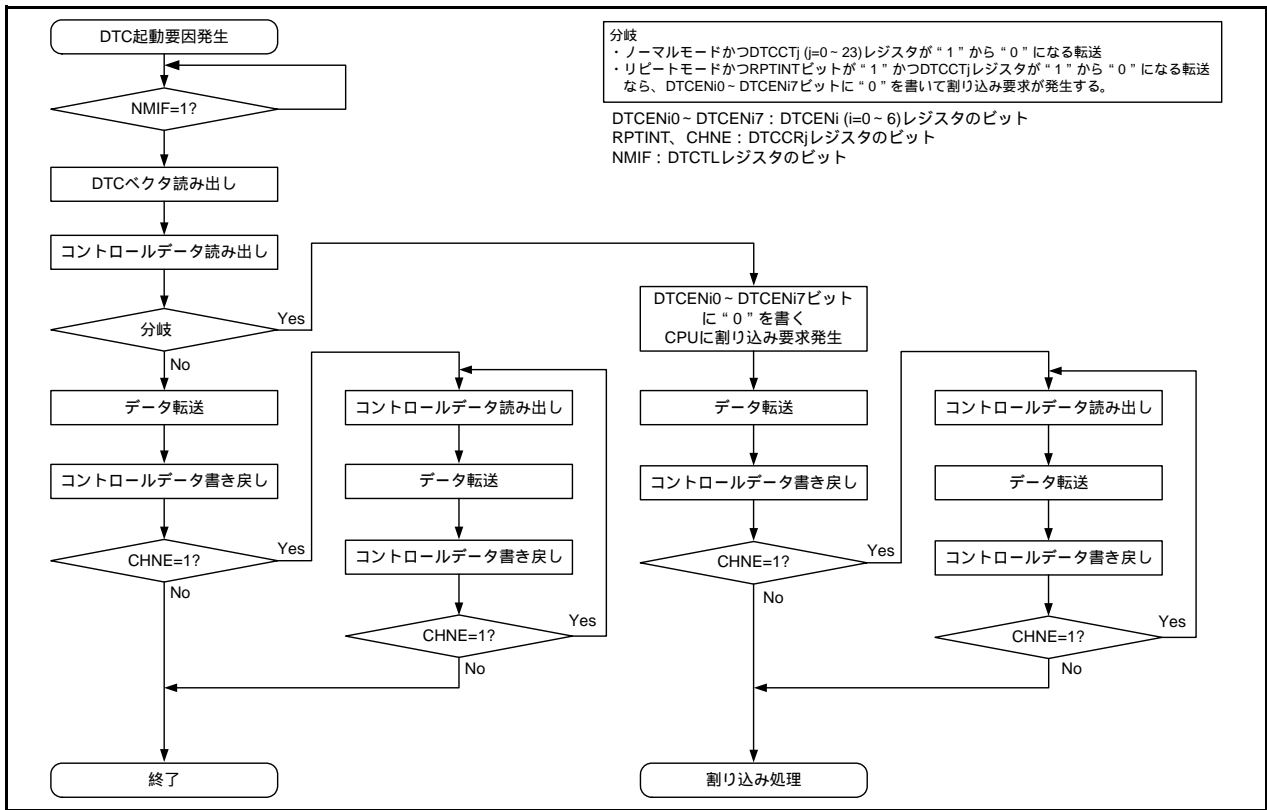
図 15.3 DTC 起動要因が SSU_I/IIC_i (i = 0 ~ 3)、タイマ RC、フラッシュメモリの割り込み要因でないときの DTC 内部動作フローチャート
