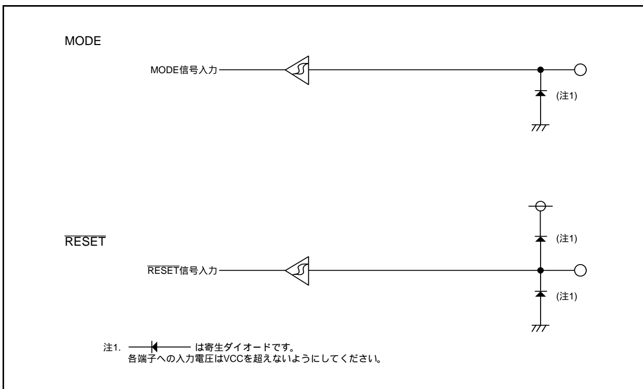
図7.15 端子の構成
