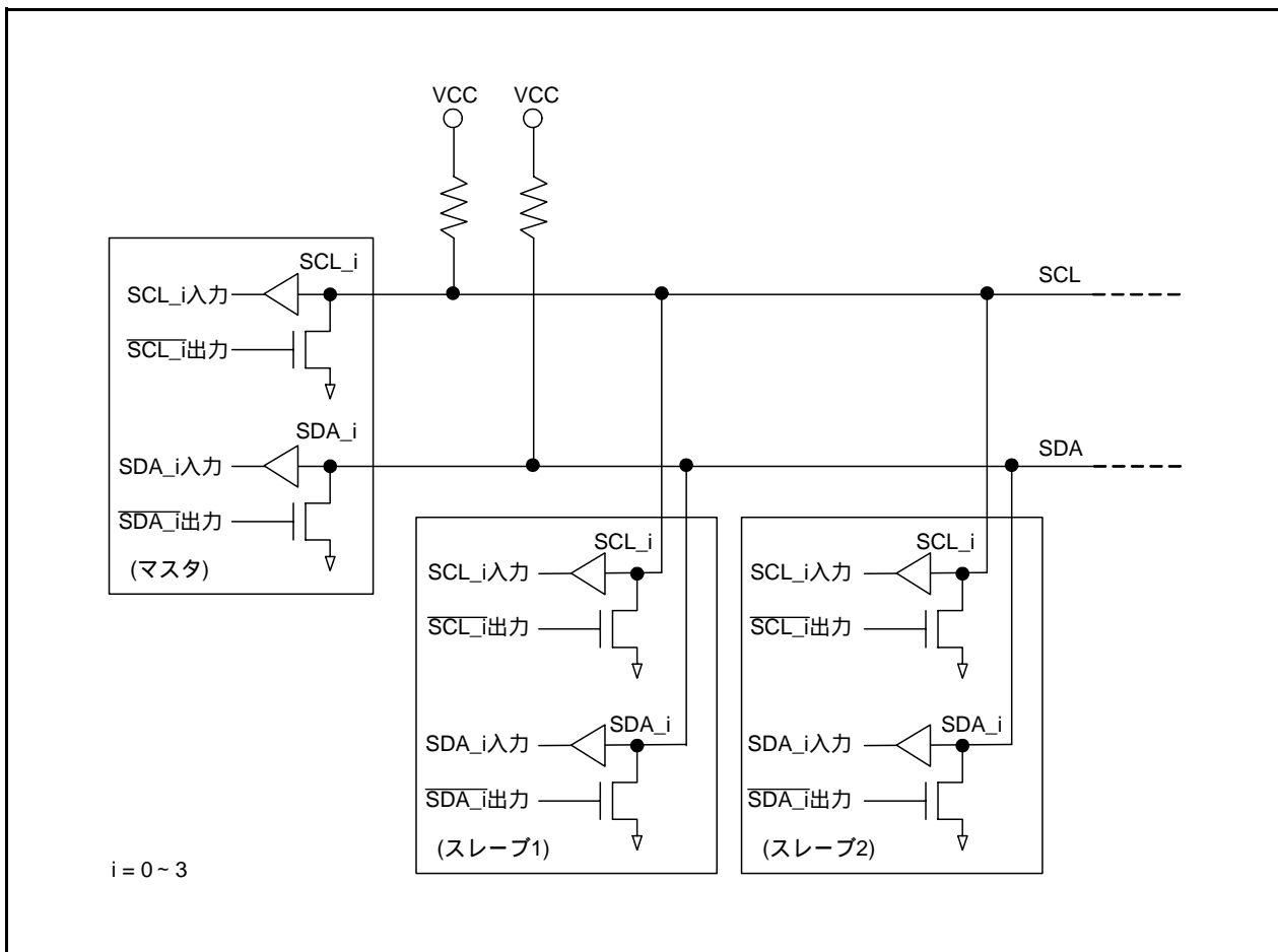
図25.2 SCL i (i = 0 ~ 3)、SDA i (i = 0 ~ 3) 端子の外部回路接続例
