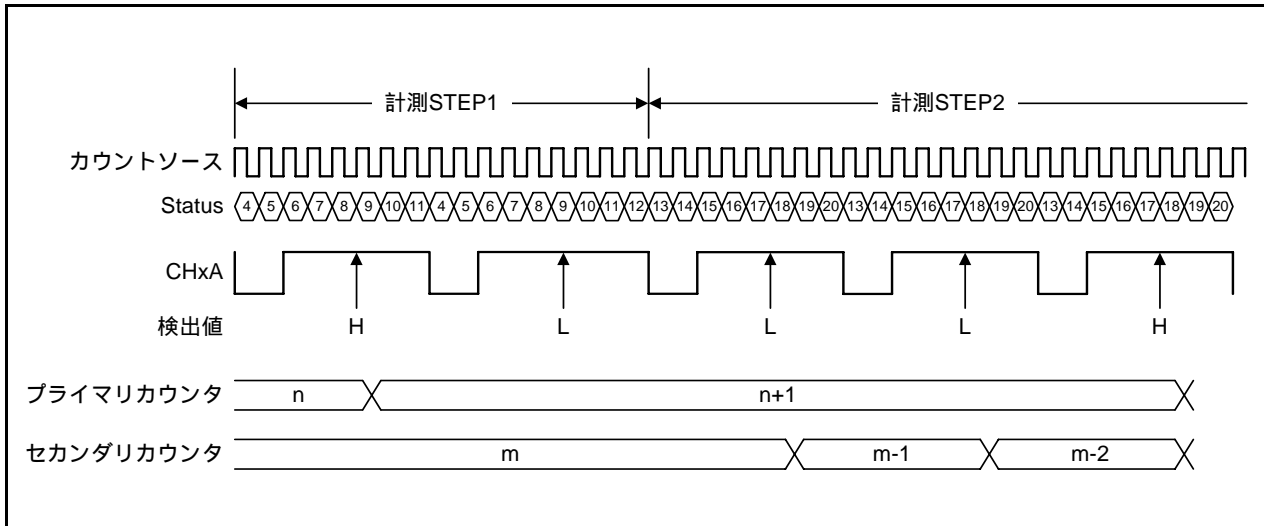
図27.4 センサコントロールユニットの検出動作例
