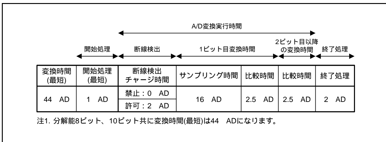
図26.3 A/D変換サイクル数(AD = fADのとき)
