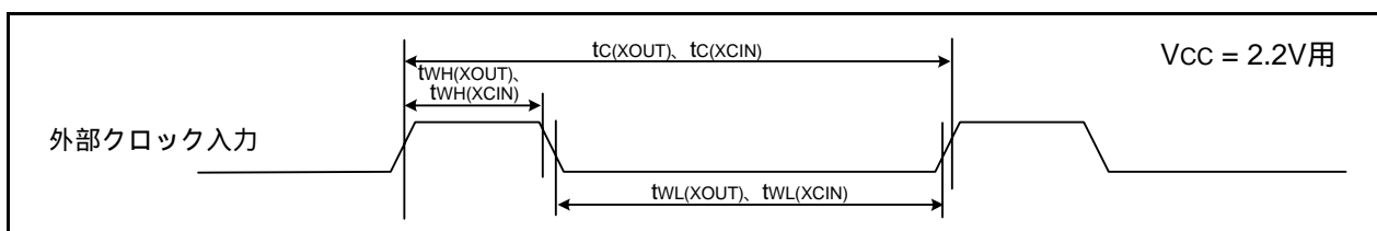
図30.16 V_{CC} = 2.2V 時の外部クロック入力タイミング
