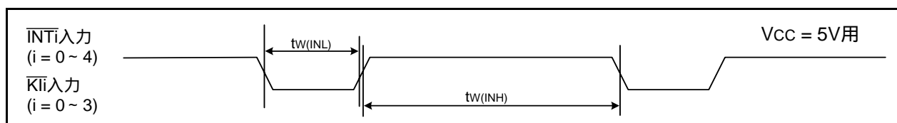
図30.11 VCC = 5V時の外部割り込み \overline{\text{INT}}_i およびキー入力割り込み \overline{\text{K}}_i 入力タイミング
