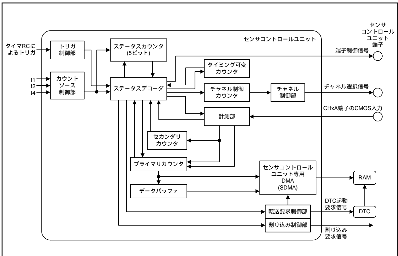
図27.2 センサコントロールユニットのブロック図
