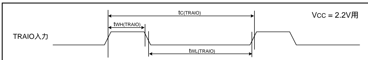
図30.17 V_{CC} = 2.2V 時のTRAIO入力タイミング
