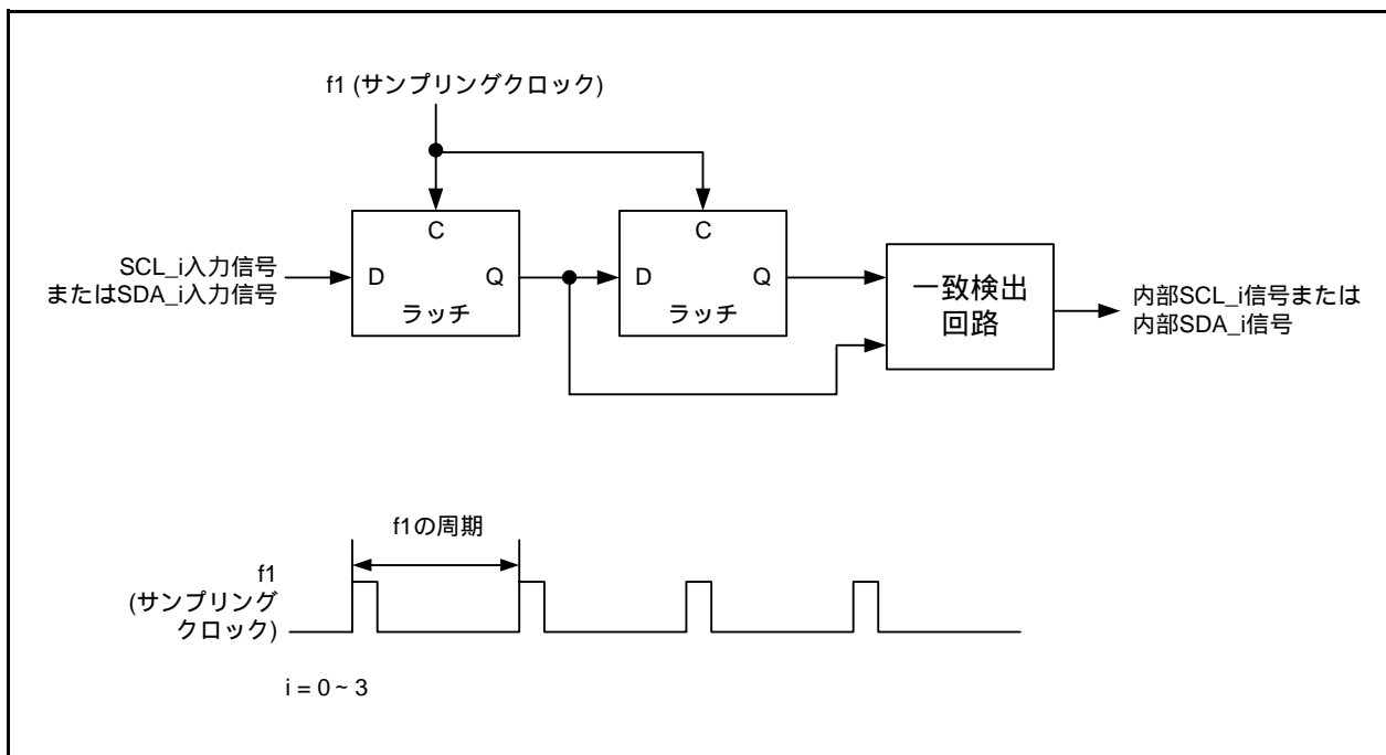
図25.20 ノイズ除去回路のブロック図
