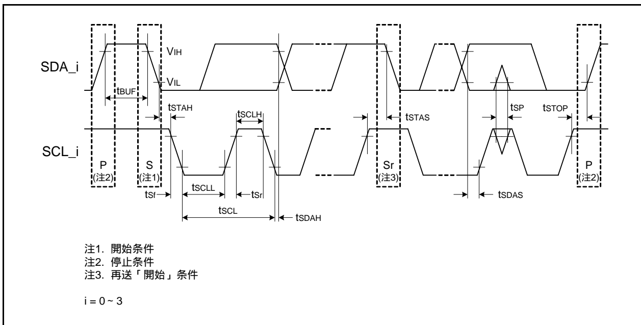
図30.7 I 2 Cバスインタフェースの入出力タイミング
