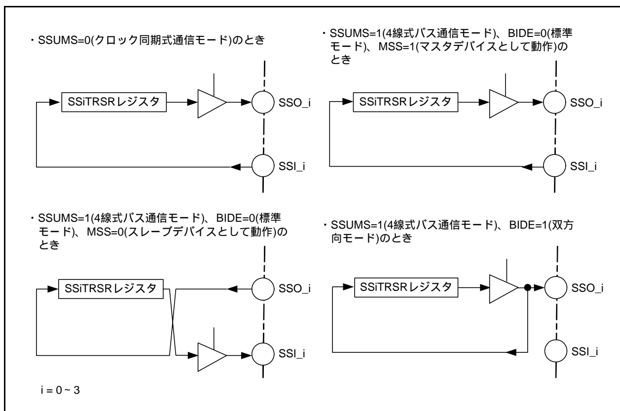
図24.3 データ入出力端子とSSiTRSRレジスタの接続関係
