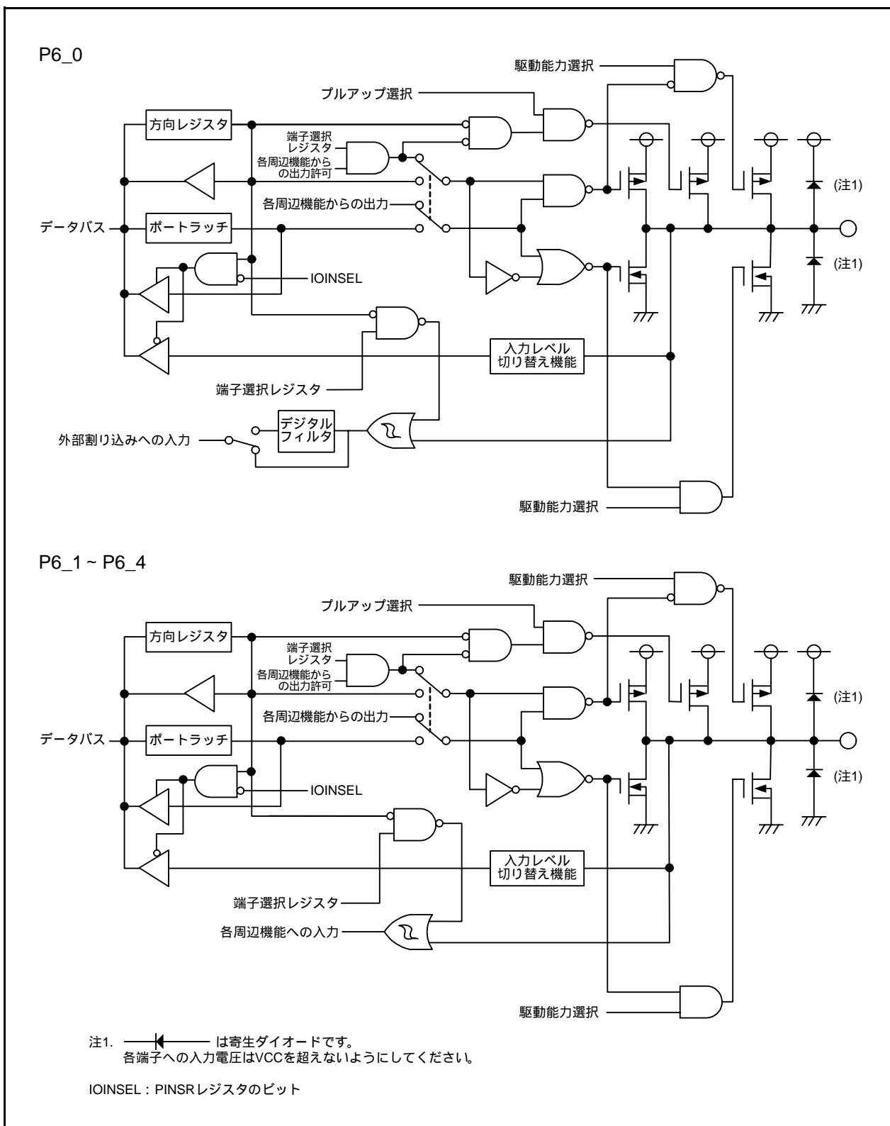
図7.13 I/Oポートの構成(13)
