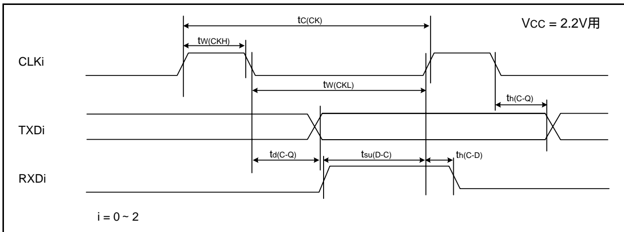
図 30.18 Vcc = 2.2V時のシリアルインタフェースのタイミング
