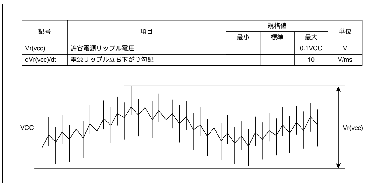
図31.3 電源リップルの定義
