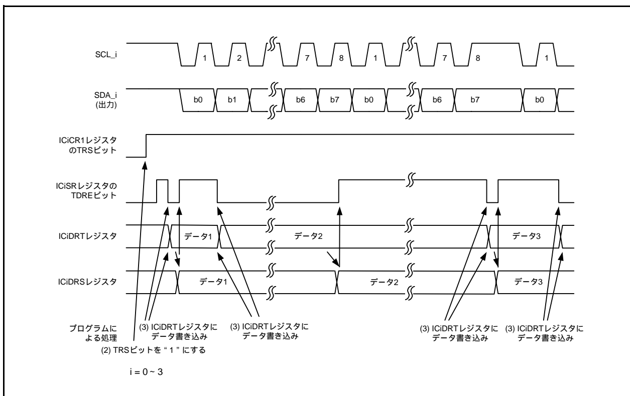
図25.14 送信モードの動作タイミング(クロック同期式シリアルモード)
