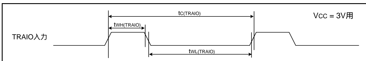
図30.13 V_{CC} = 3V 時のTRAIO入力タイミング
