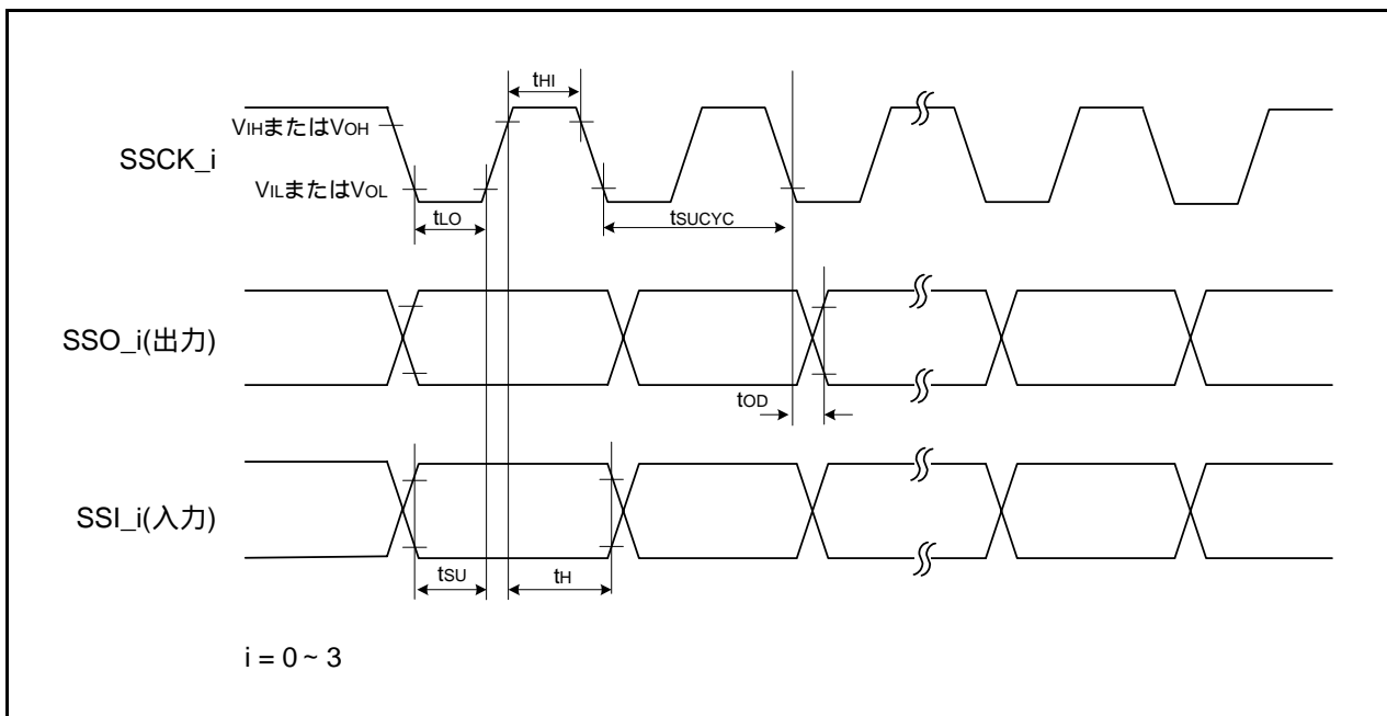
図30.6 シンクロナスシリアルコミュニケーションユニット(SSU)の入出力タイミング(クロック同期式通信モード)
