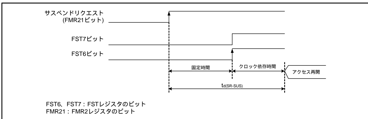
図30.2 サスペンドへの遷移時間
