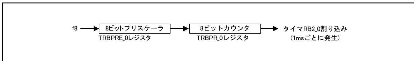
図1.1 ブロック図
