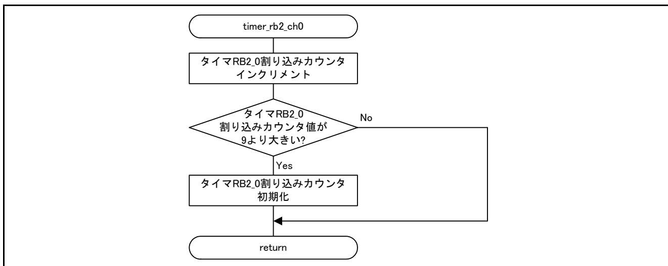
図3.5 タイマ RB2_0 割り込み処理
