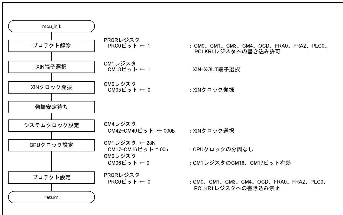
図3.3 システムクロック設定処理
