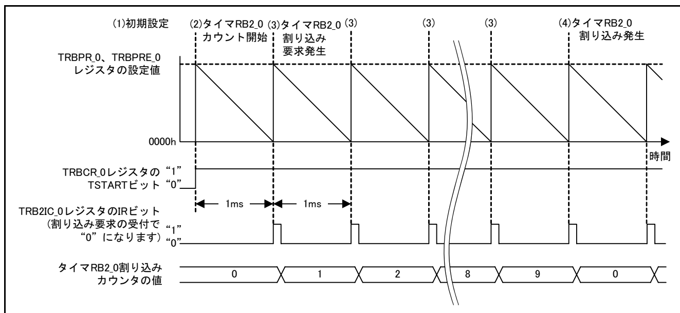
図3.1 タイミング図
