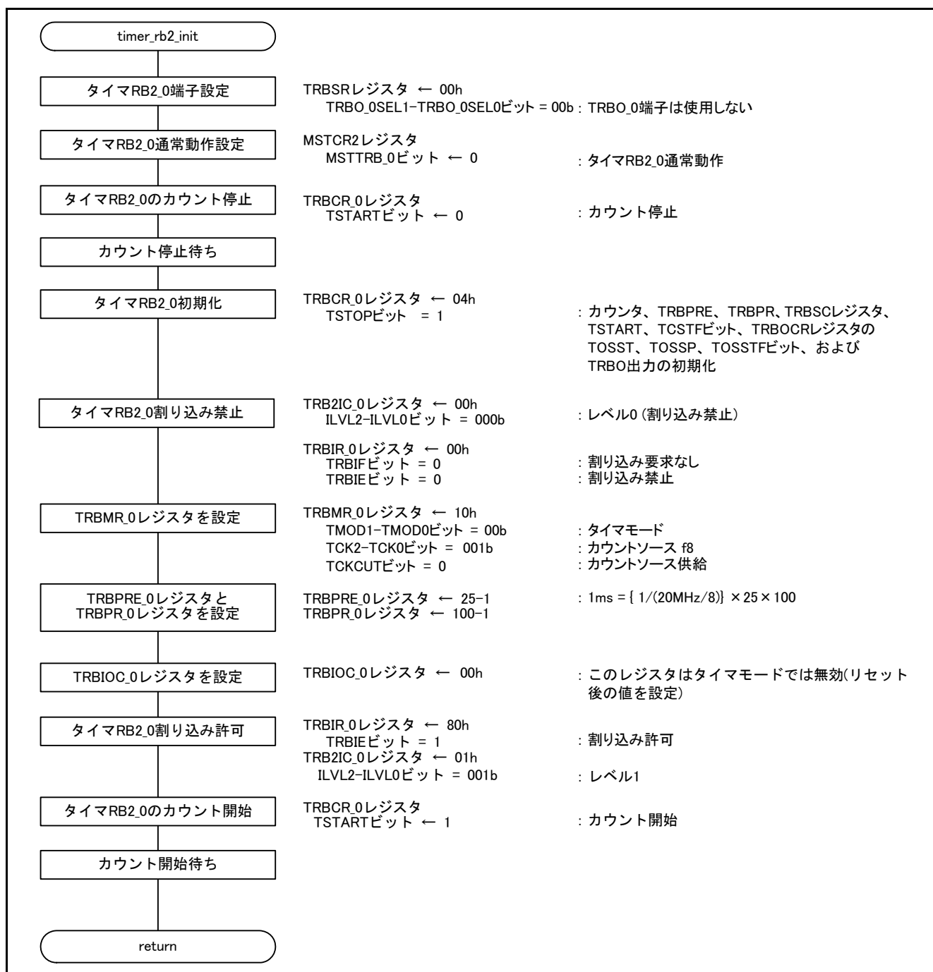
図3.4 タイマ RB2_0 初期設定処理
