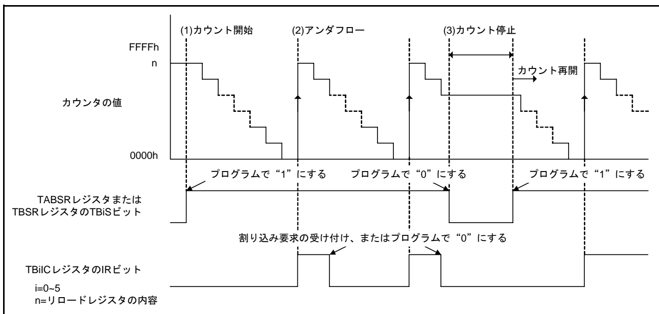
図 3.1 タイマモードの動作
