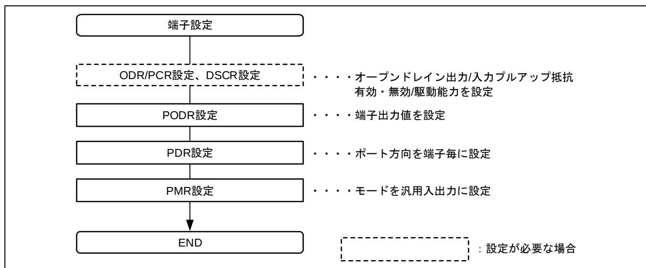
図 2.3 RX651 I/O 汎用入出力を使用する場合
