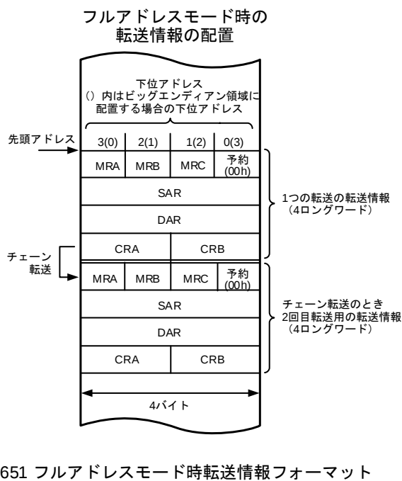
図 2.9 SH7044、RX651 DTC 転送情報フォーマット
