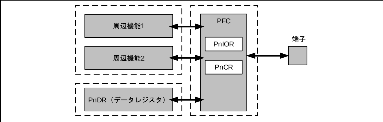
図 2.1 SH7044 I/O 設定
